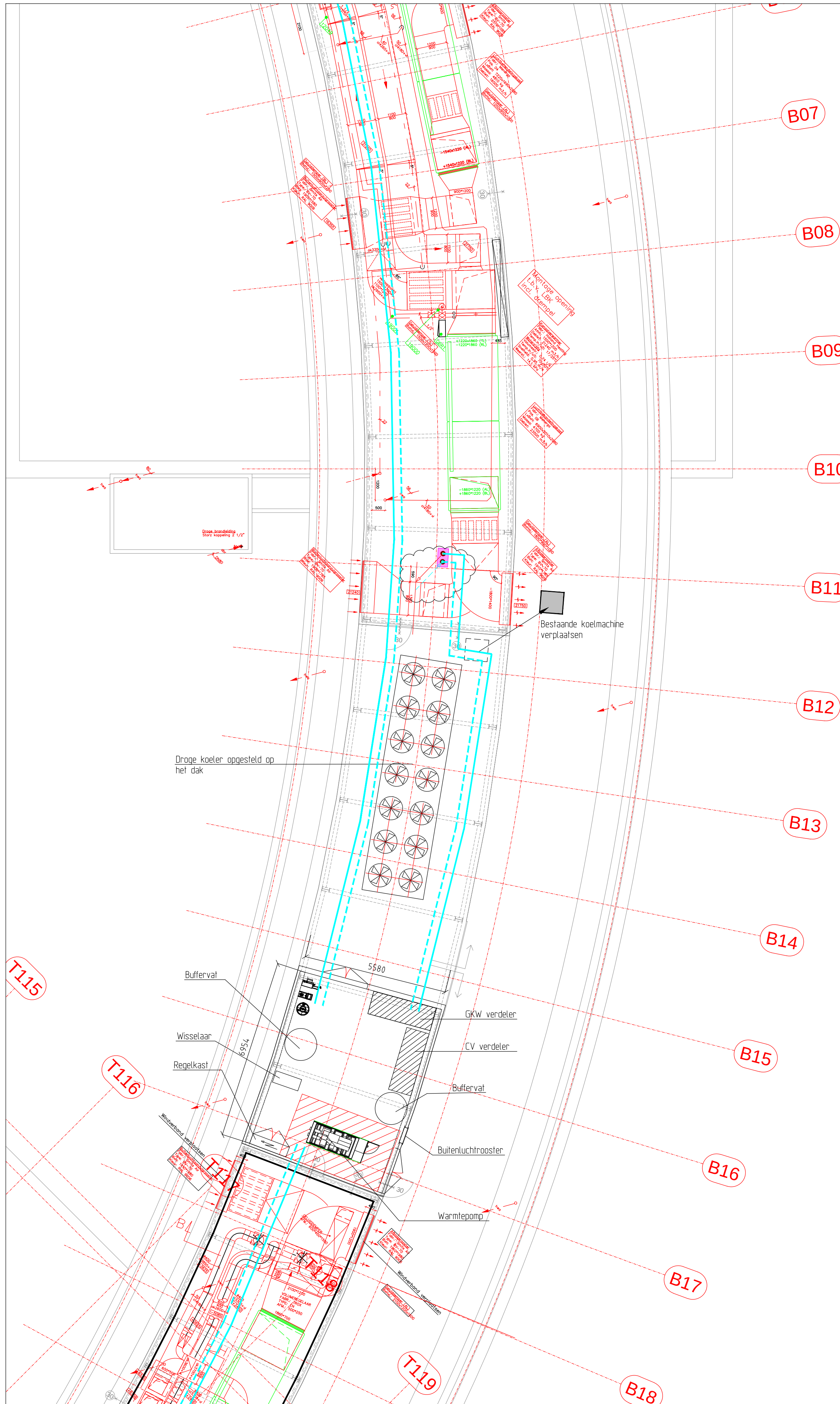
6e verdieping, A-Vleugel
