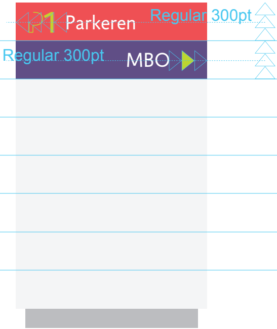
Voorzijde zuil 1600 x 1000 mm (h x b) RAL 9003 Signal wit
