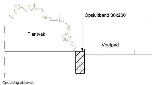
Afsluiting groenvakken
