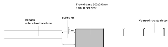
Opsluiting rijbaan – trottoir binnenstad (3)
