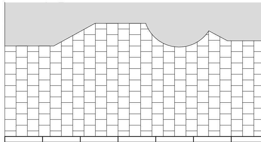
Aansluiting betontegels om trottoirband en schuine gevel
