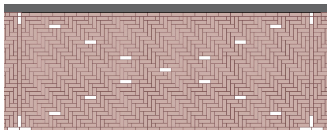
Principe kruismarkering parkeervakken (parkeren in vak, dikformaat)
