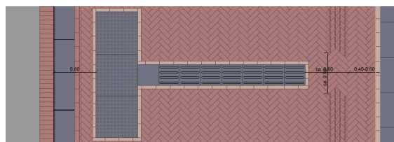
Voorbeelddetail geleidesysteem Breestraat met standaard detail oversteek, bij de overgang tussen de twee lijnen is een attentievak vrijgehouden. De noppentegels vormen de waarschuwingsmarkering. Voor de verplichte onderbreking tussen ribbels en noppentegels is gekozen voor een vlakke natuursteen tegel.
