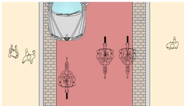
Principe inrichting smalle fietsstraat (bron: CROW)
