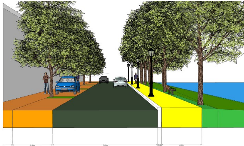
Figuur 1: principeprofiel singelweg (naar Rijnsburgersingel-Maresingel)
