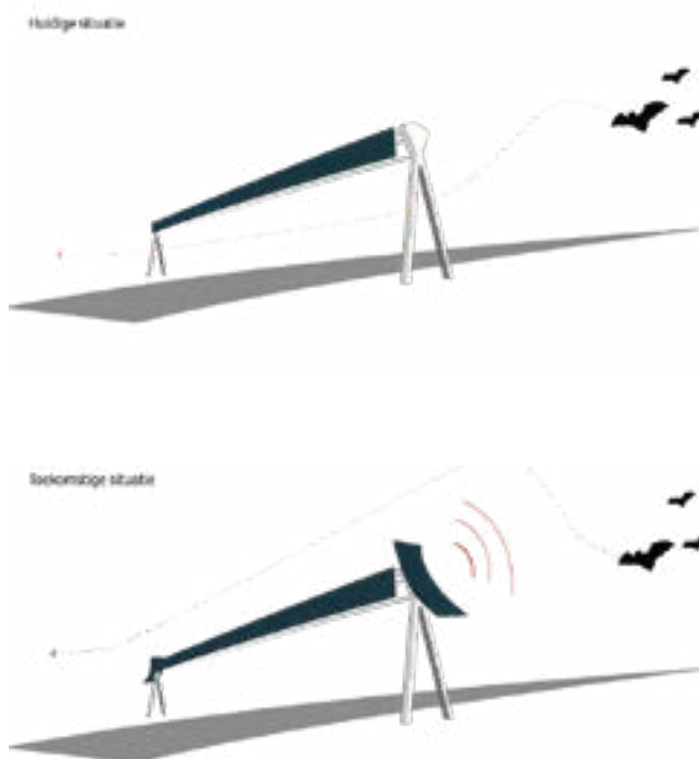
Voorziening aan de kopse einden van het portaal, zodat de vleermuizen horen waar het portaal begint. NB: het portaal wordt zo geplaatst dat het aansluit op bomen aan weerszijden van de weg (niet weergegeven in deze figuur)
