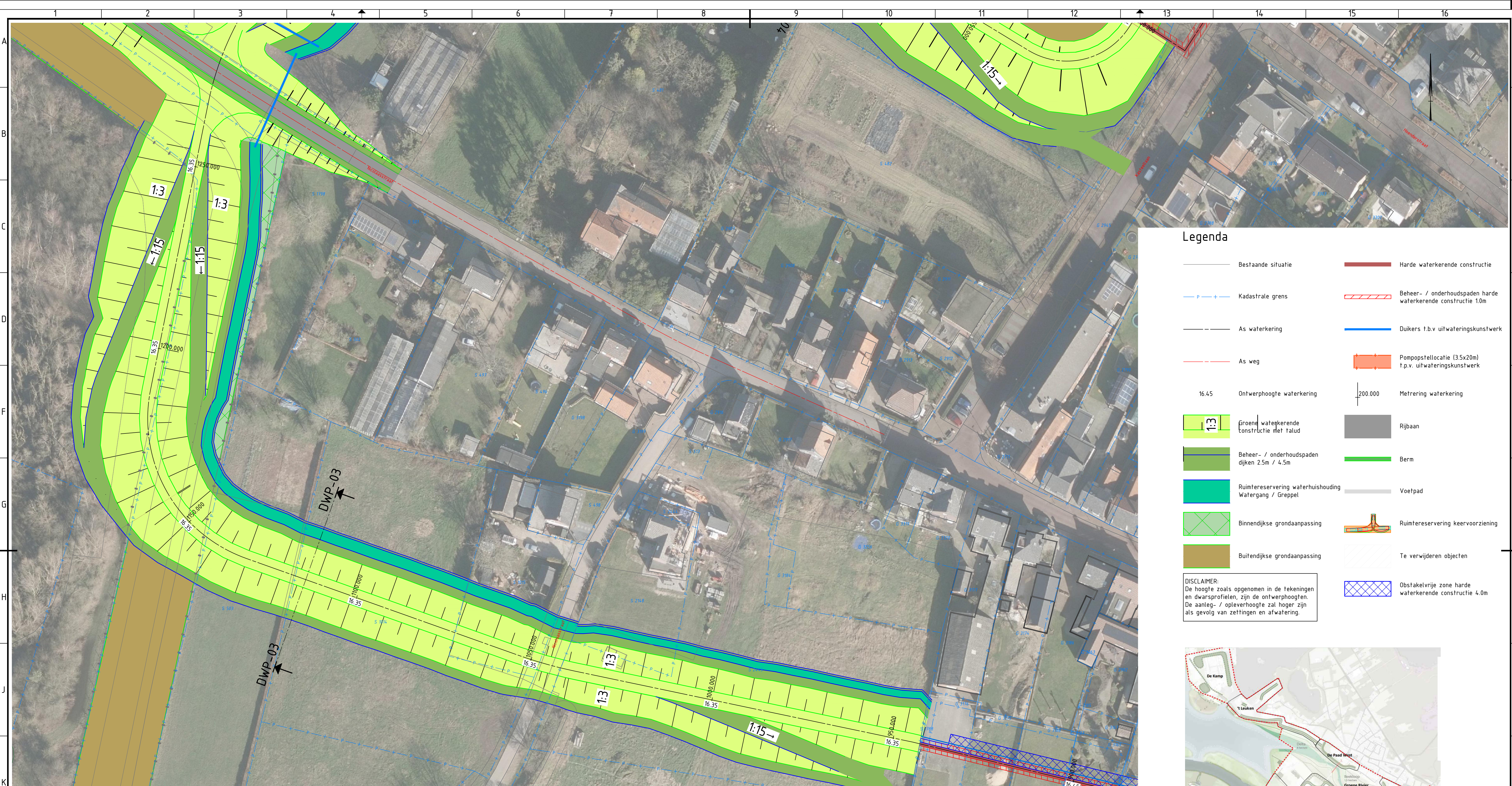
Overzicht Oud Well - Dijkteruglegging SCHAAL 1 : 500
