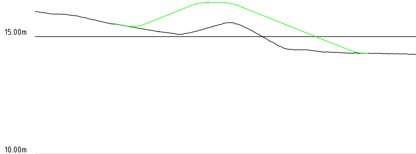
ALM-AS-Weg-Weideweg-DG1 13 Lengteprofiel as ALM-AS-Weg-Weideweg-DG1 Metrering 0.000 tot 161.822
