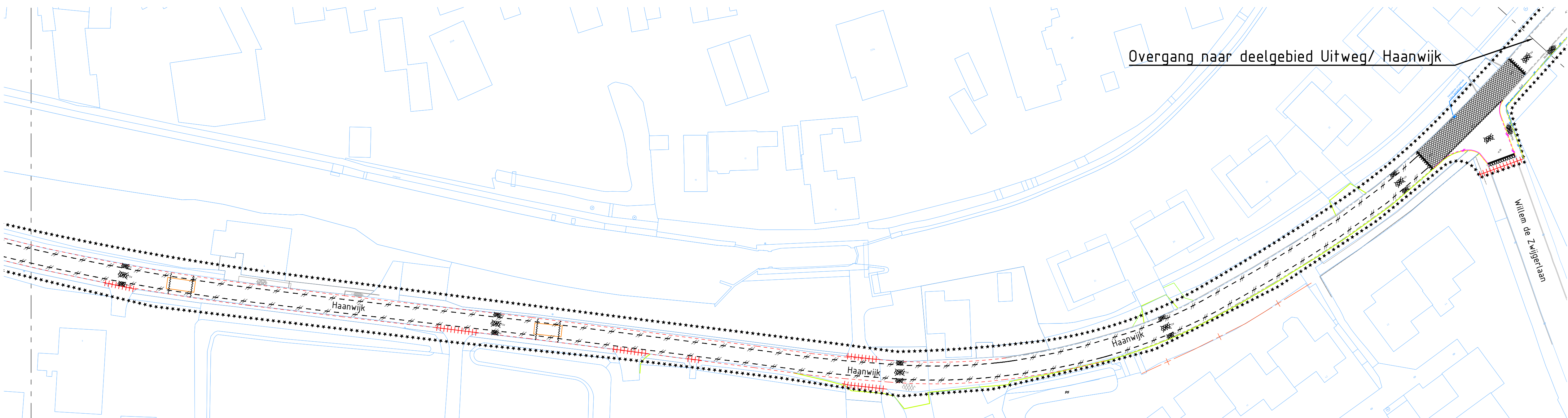
OVERZICHTSTEKENING Haanwijk SCHAAL 1:500
