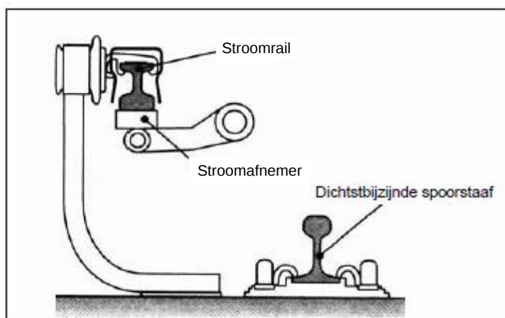
Figuur 9-1 Doorsnede spoorstaaf en stroomrail
