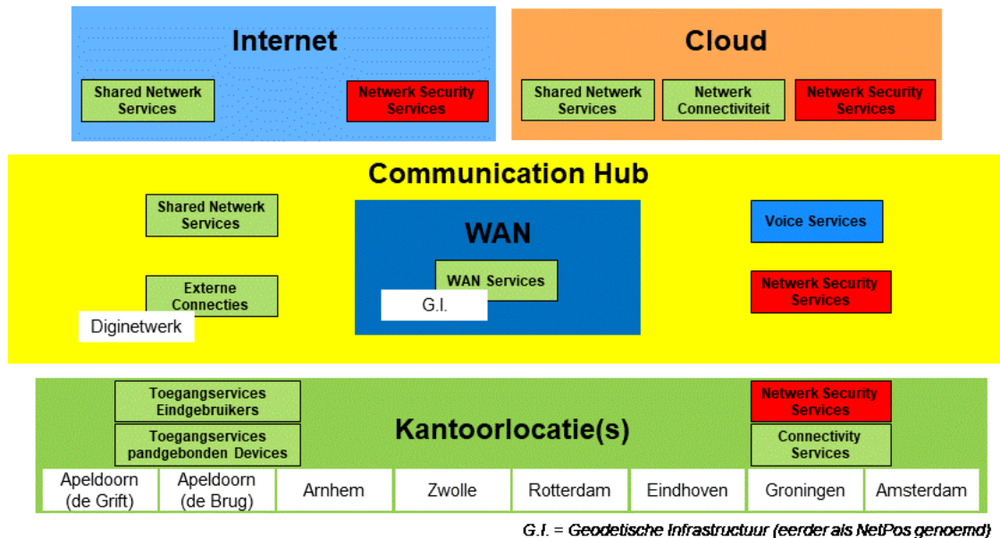
Figuur 4: Visuele weergave doelarchitectuur
