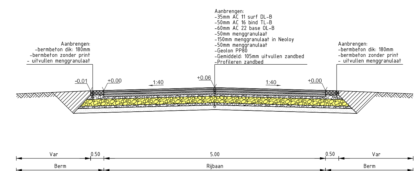
Principeprofiel G-G
