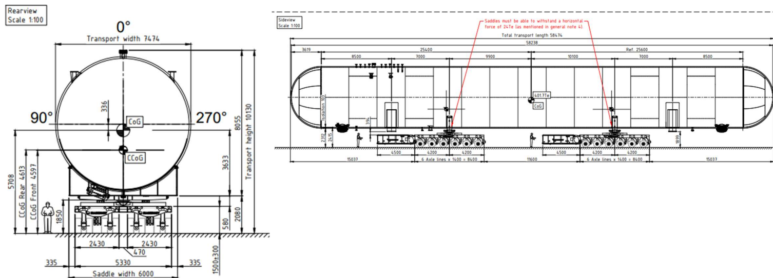
Figuur 2 Afmetingen bullets
