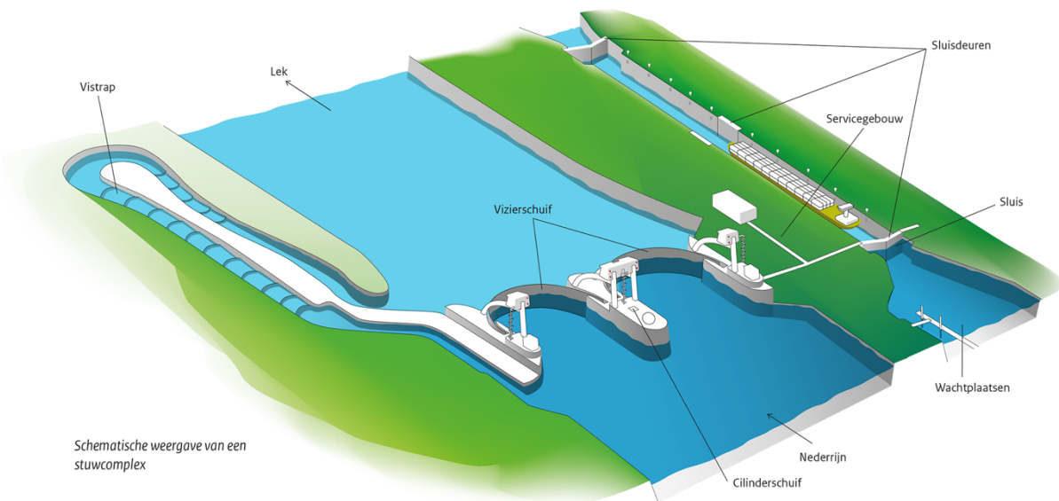
Figuur 3 Sluis- en stuwcomplex Vlotdorp
