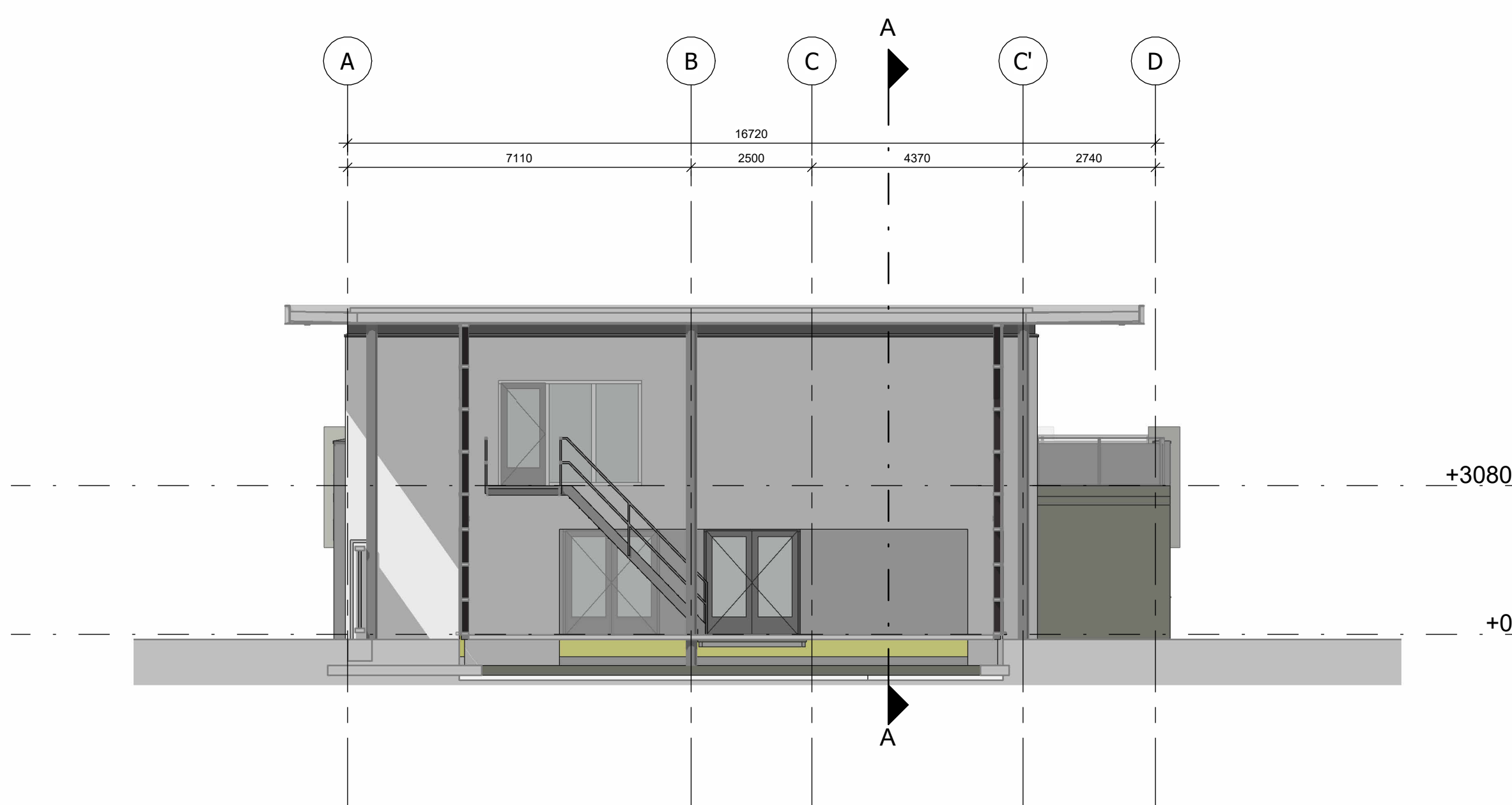
RECHTER ZIJGEVEL (OOST)
