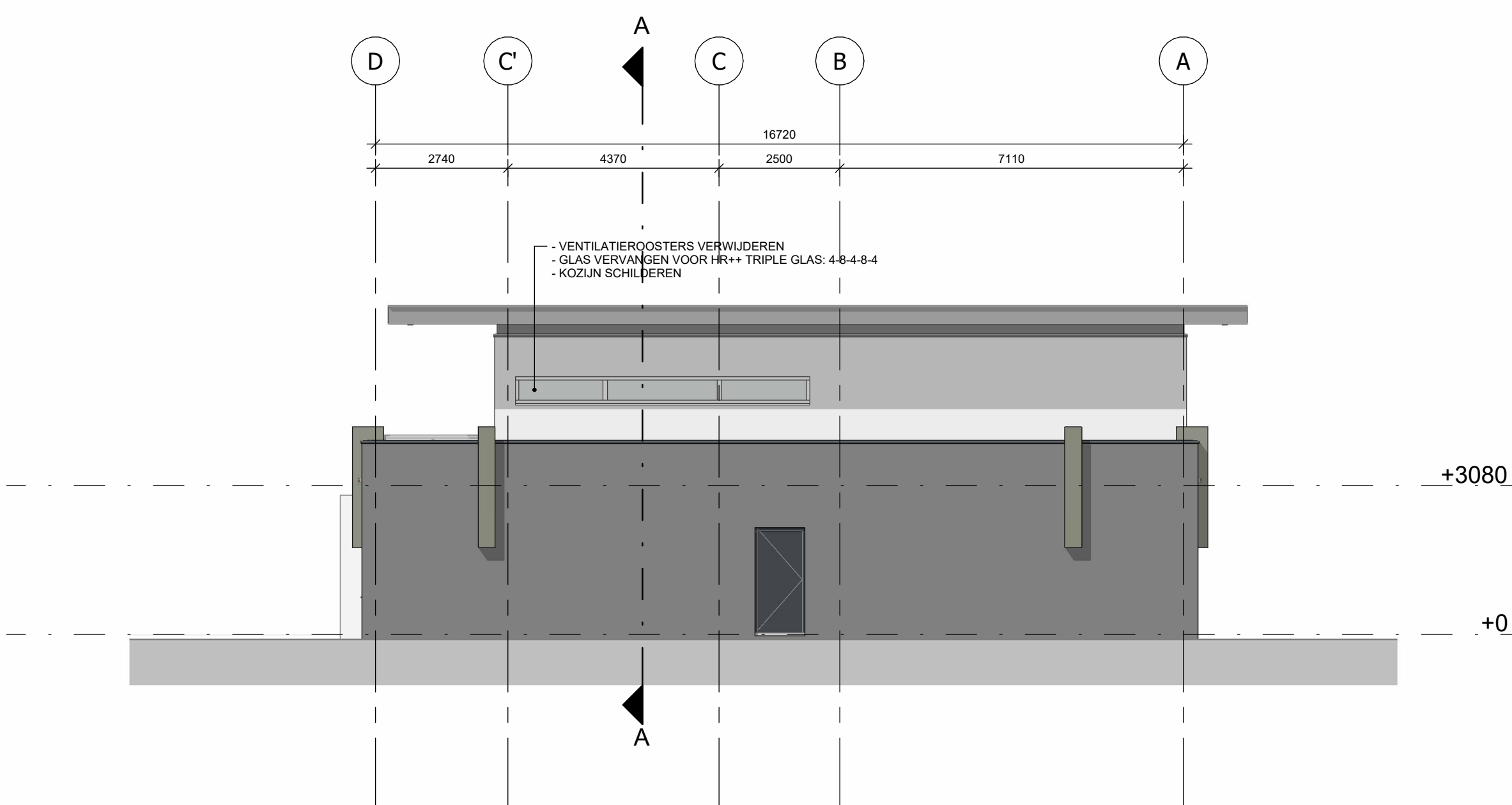
LINKER ZIJGEVEL (WEST)
