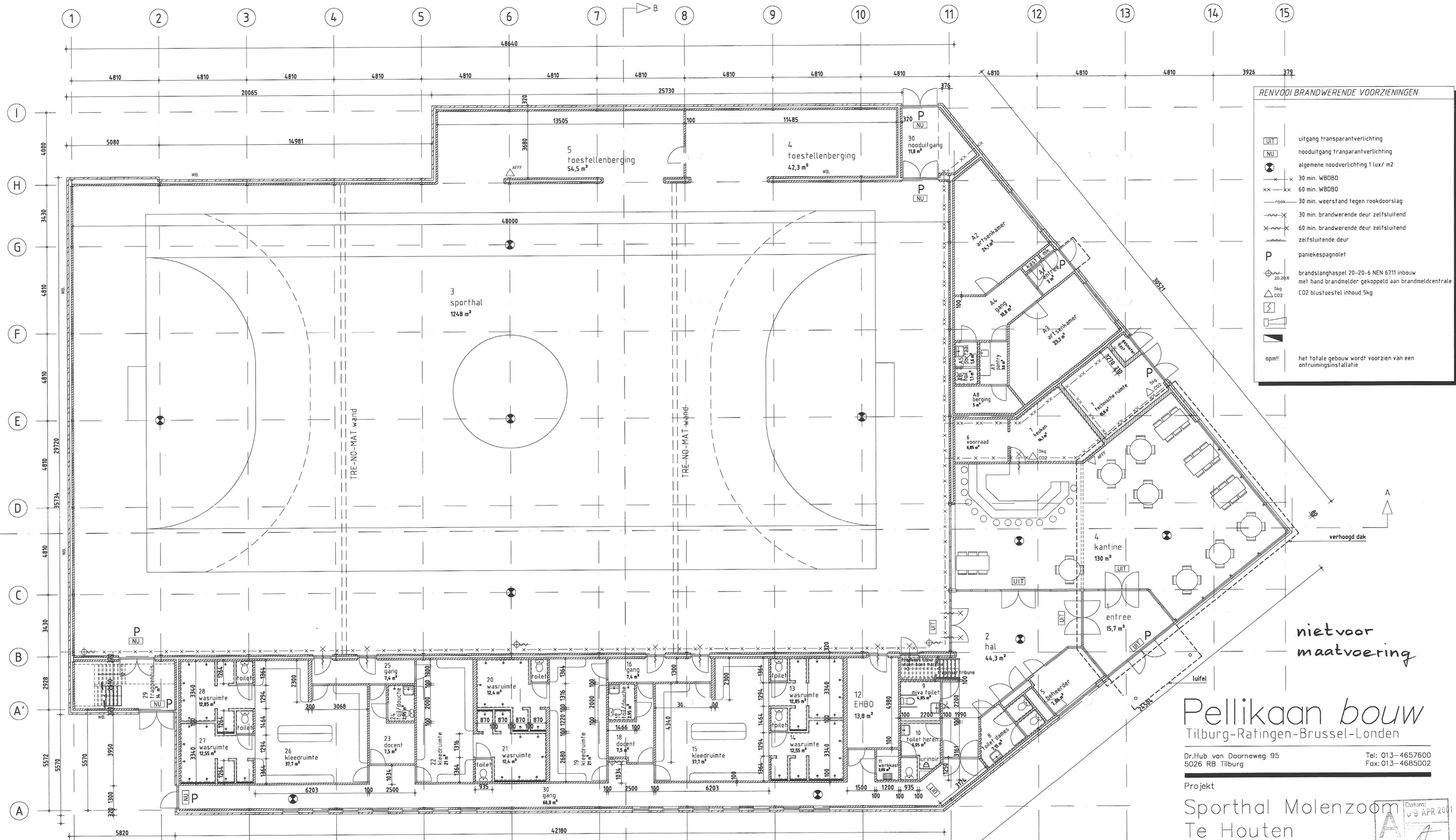
PLATTEGROND BEGANE GROND
