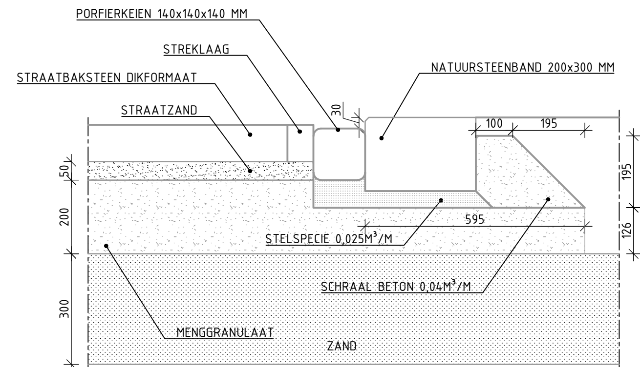
DETAIL 45 CATEGORIE 7 (FIETSPAD) NATUURSTEENBAND LANGS ELEMENTEN OP FUNDERING LAAG/HOOG PROFIEL MET GOOTLAAG VAN KEIEN SCHAAL 1:10
