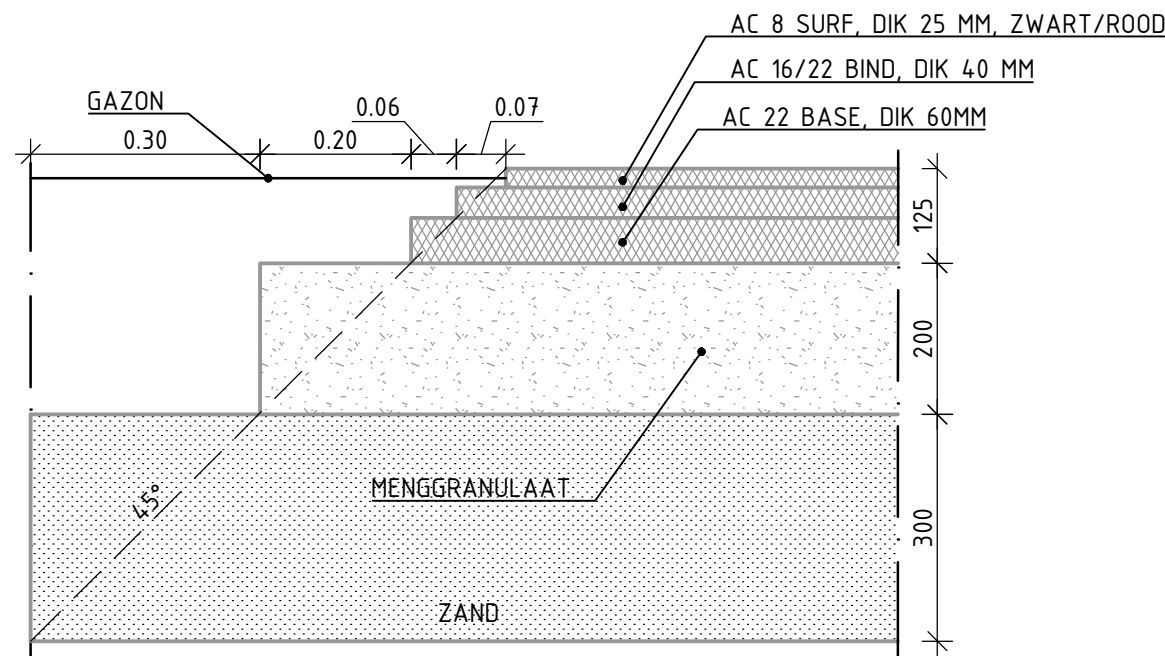
DETAIL 33 CATEGORIE 7 (FIETSPAD) ZONDER KANTOPSLUITING SCHAAL 1:10
