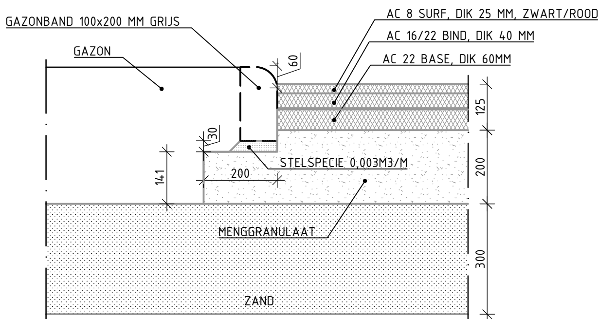
DETAIL 35 CATEGORIE 7 (FIETSPAD) GAZONBAND LANGS ASFALT SCHAAL 1:10
