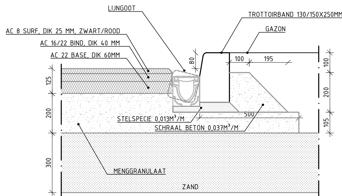
DETAIL 40 CATEGORIE 7 (FIETSPAD) TROTTOIRBAND LANGS ASFALT OP FUNDERING LAAG PROFIEL MET LIJNGOOT INCL. GOOTLAAG VAN KEIEN SCHAAL 1:10
