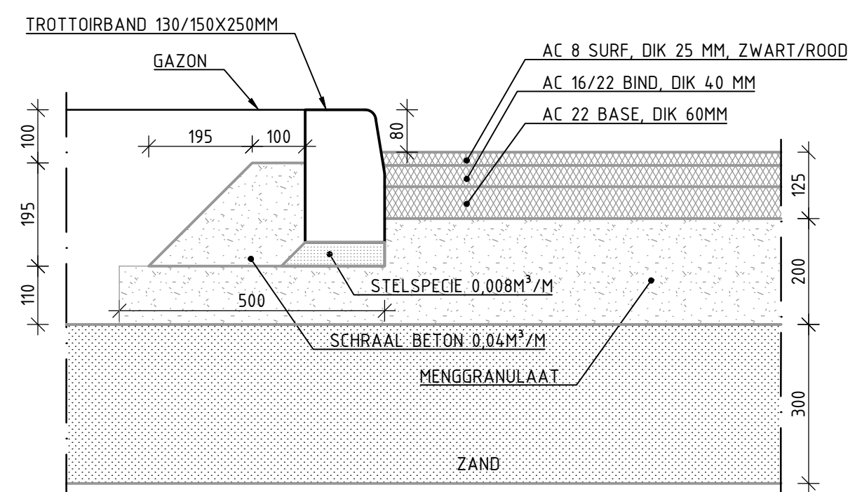
DETAIL 36 CATEGORIE 7 (FIETSPAD) TROTTOIRBAND LANGS ASFALT OP FUNDERING HOOG PROFIEL ZONDER GOOTLAAG SCHAAL 1:10
