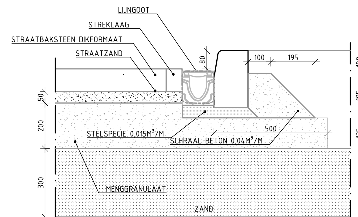
DETAIL 42 CATEGORIE 7 (FIETSPAD) TROTTOIRBAND LANGS ELEMENTEN OP FUNDERING LAAG PROFIEL MET LIJNGOOT INCL. GOOTLAAG VAN KEIEN SCHAAL 1:10
