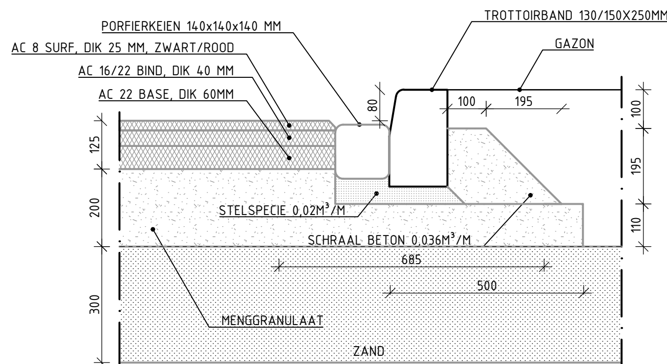
DETAIL 39 CATEGORIE 7 (FIETSPAD) TROTTOIRBAND LANGS ASFALT OP FUNDERING LAAG/HOOG PROFIEL MET GOOTLAAG VAN KEIEN SCHAAL 1:10
