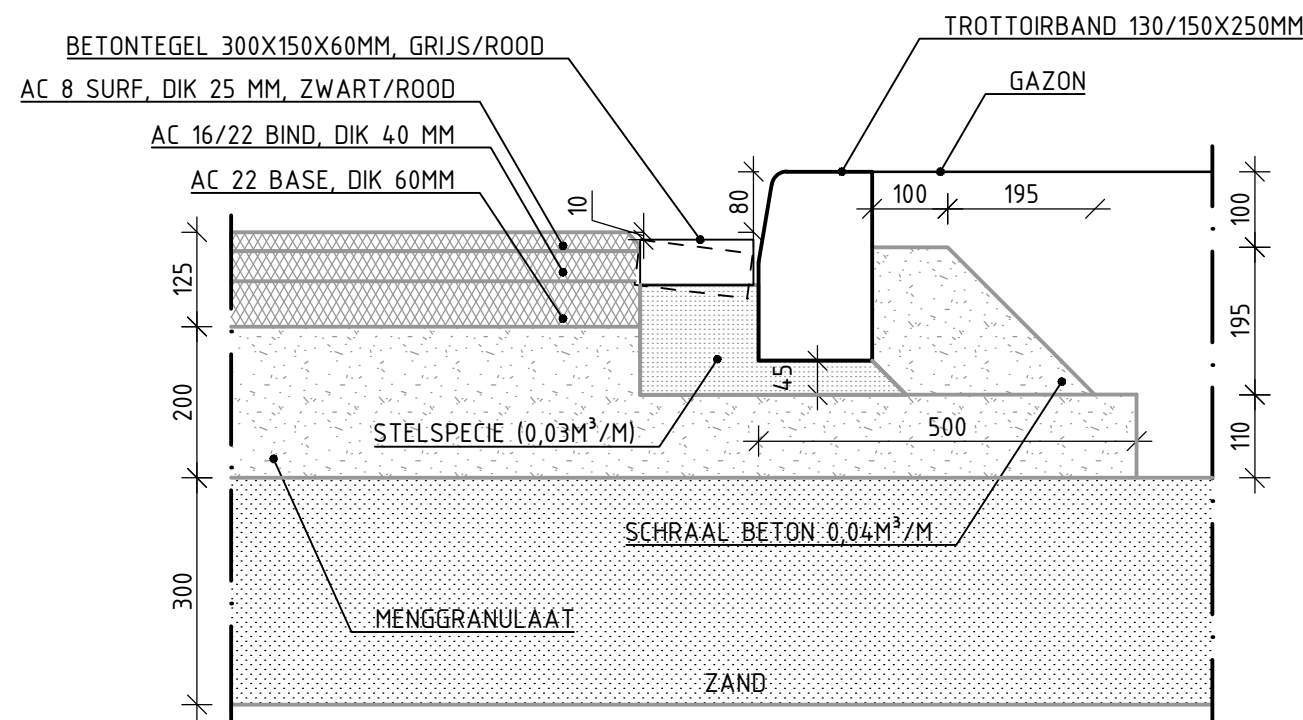
DETAIL 37 CATEGORIE 7 (FIETSPAD) TROTTOIRBAND LANGS ASFALT OP FUNDERING LAAG PROFIEL MET GOOTLAAG VAN TEGELS SCHAAL 1:10
