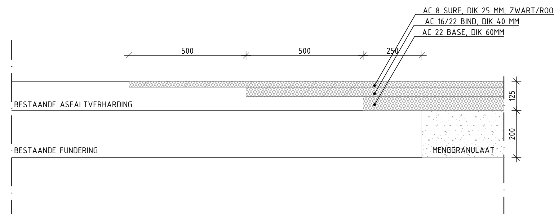
DETAIL 47 CATEGORIE 7 (FIETSPAD) LIPLAS SCHAAL 1:10
