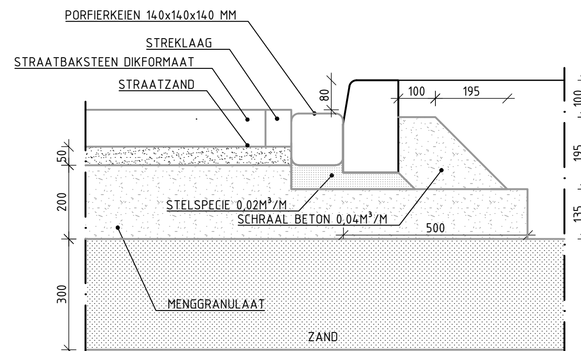
DETAIL 41 CATEGORIE 7 (FIETSPAD) TROTTOIRBAND LANGS ELEMENTEN OP FUNDERING LAAG/HOOG PROFIEL MET GOOTLAAG VAN KEIEN SCHAAL 1:10
