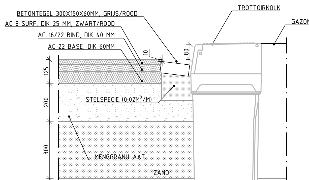
DETAIL 38 CATEGORIE 7 (FIETSPAD) TROTTOIRKOLK LANGS ASFALT LAAG PROFIEL MET GOOTLAAG VAN TEGELS SCHAAL 1:10
