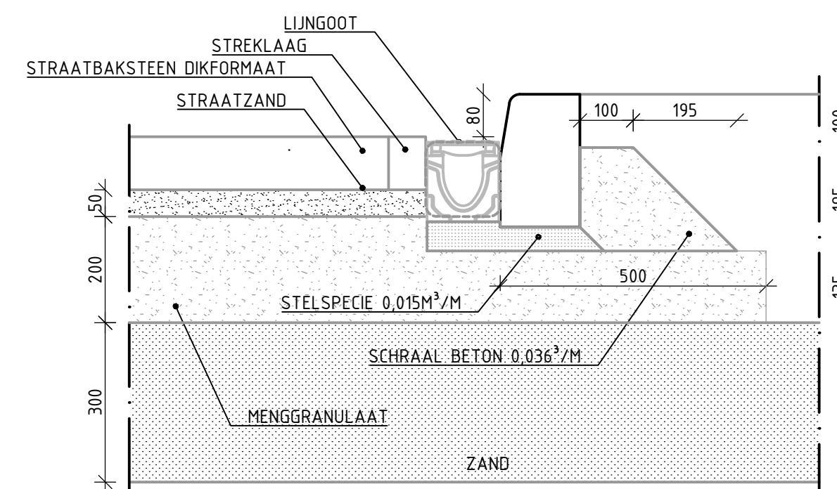
DETAIL 44 CATEGORIE 7 (FIETSPAD) TROTTOIRBAND LANGS ELEMENTEN OP FUNDERING LAAG PROFIEL MET LIJNGOOT INCL. GOOTLAAG VAN KEIEN SCHAAL 1:10
