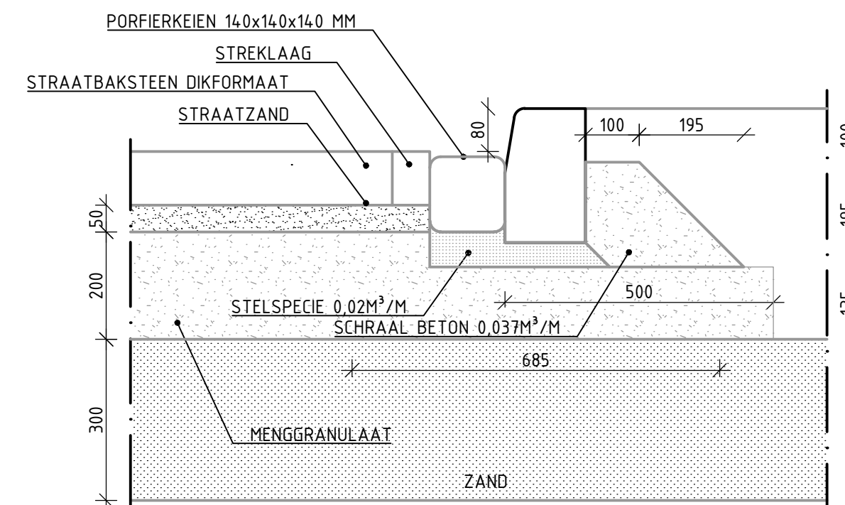
DETAIL 43 CATEGORIE 7 (FIETSPAD) TROTTOIRBAND LANGS ELEMENTEN OP FUNDERING LAAG/HOOG PROFIEL MET GOOTLAAG VAN KEIEN SCHAAL 1:10
