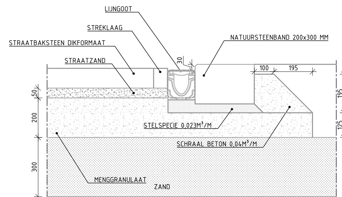
DETAIL 46 CATEGORIE 7 (FIETSPAD) NATUURSTEENBAND LANGS ELEMENTEN OP FUNDERING LAAG PROFIEL INCL. LIJNGOOT MET GOOTLAAG VAN KEIEN SCHAAL 1:10
