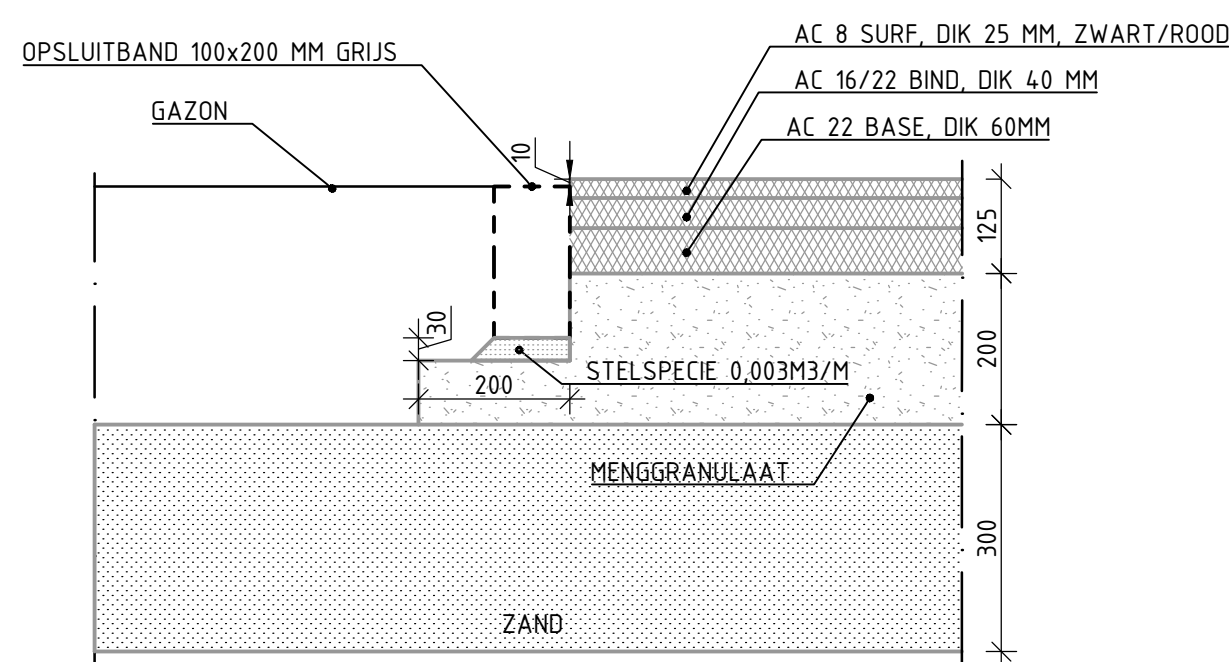
DETAIL 34 CATEGORIE 7 (FIETSPAD) OPSLUITBAND LANGS ASFALT SCHAAL 1:10
