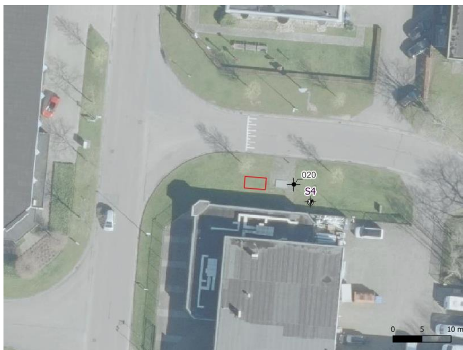
Figuur 3-1 Overzichtstekening met sondering S4 en de nabije boring van BK Ingenieurs B.V.
