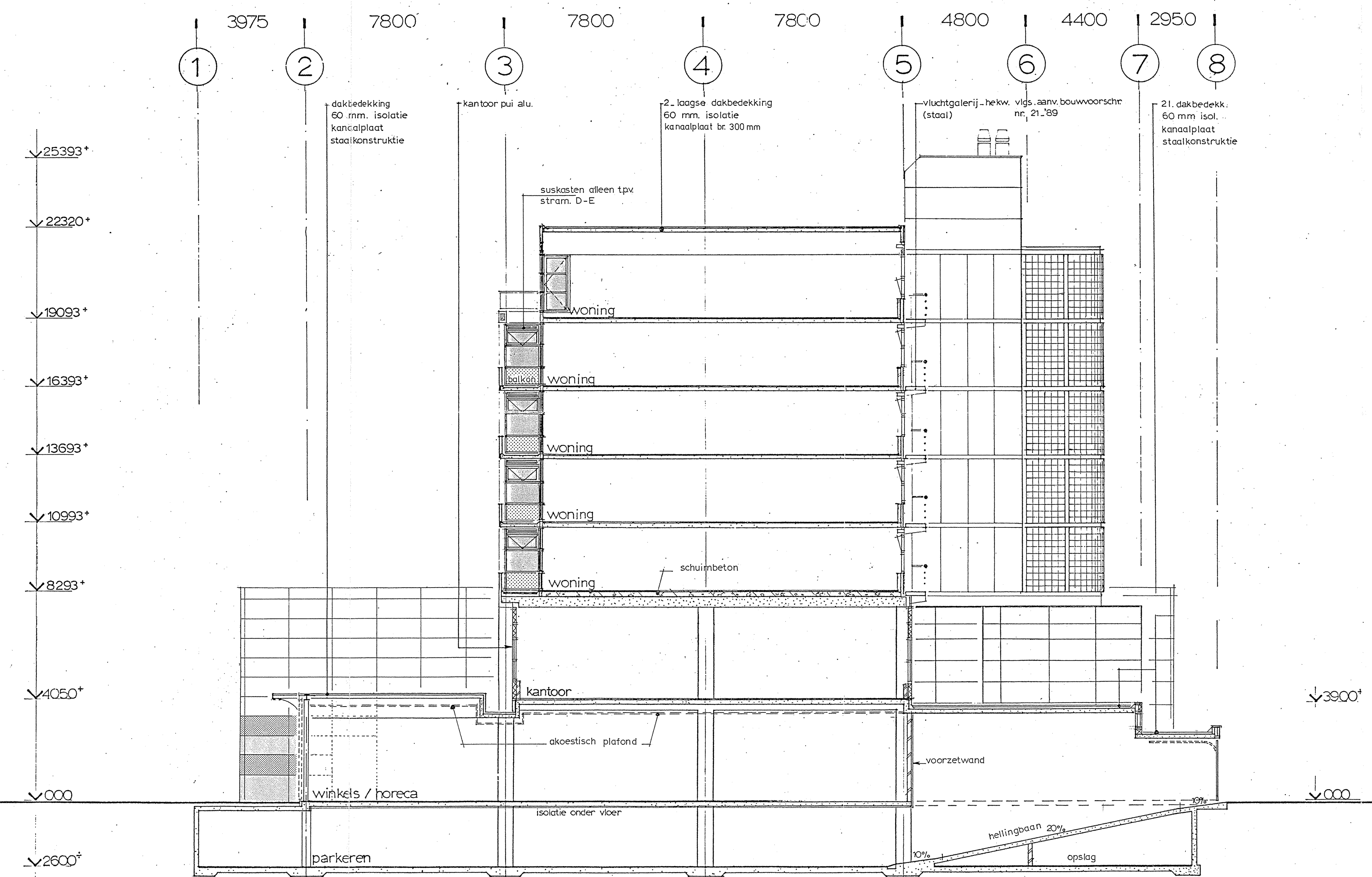
dwarsdoorsnede A-A
