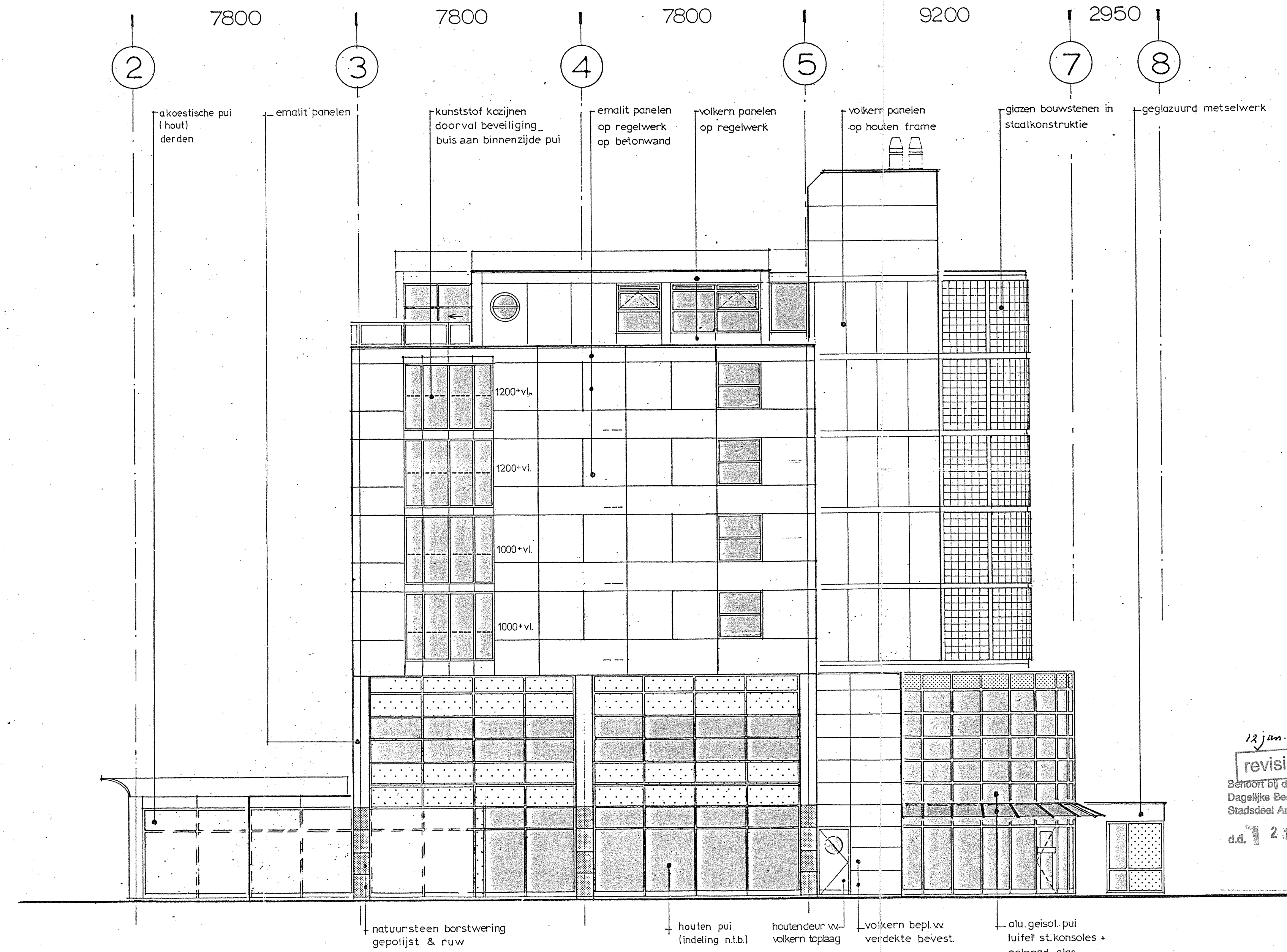
zuid - oost gevel
