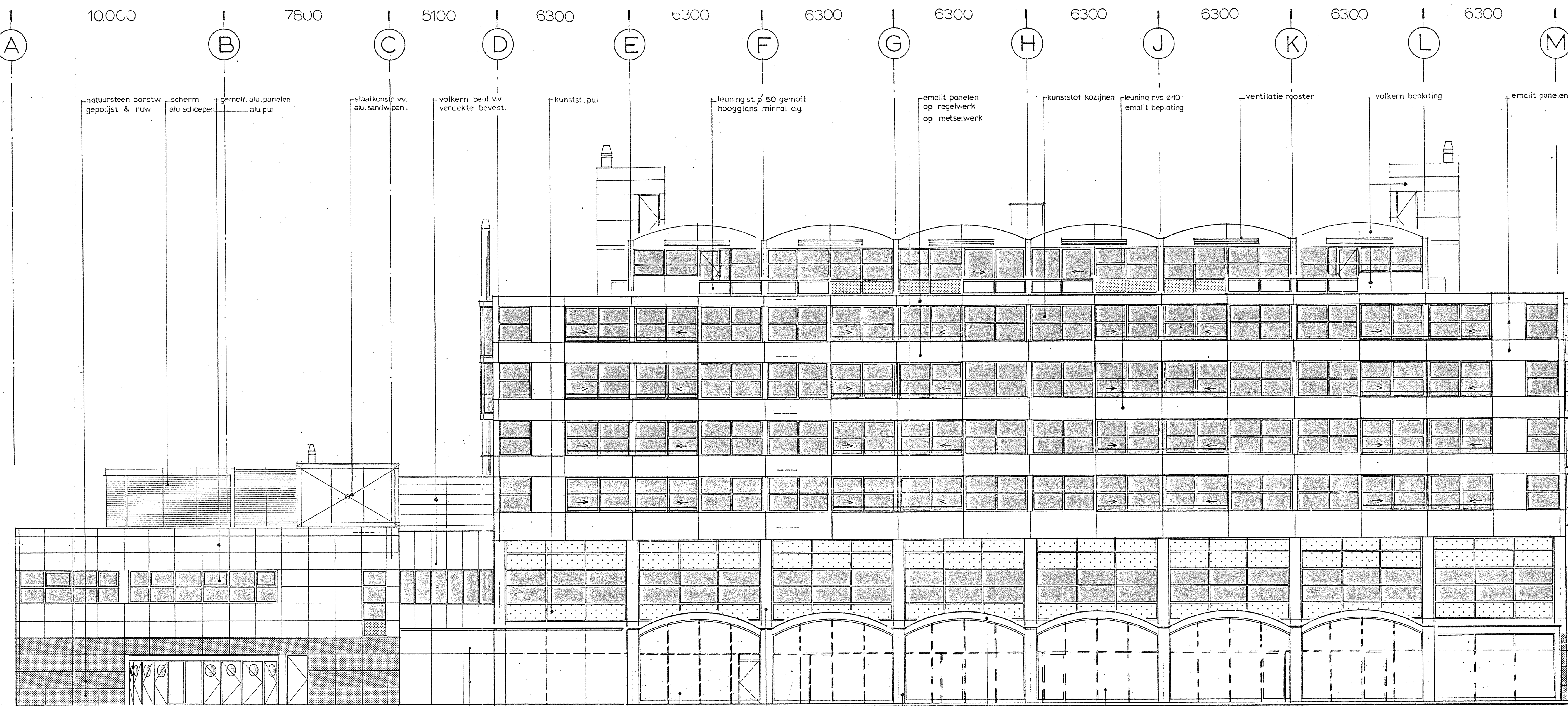
zuid - west gevel buikslotermeerplein
