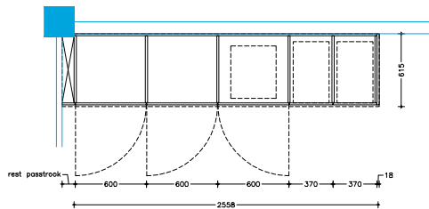
- horizontale snede -
