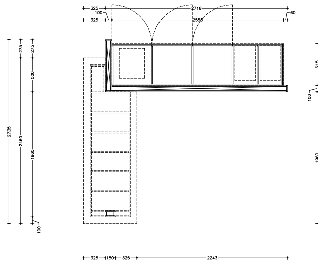
- horizontale snede -
