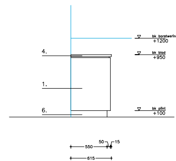
- zij aanzicht -
