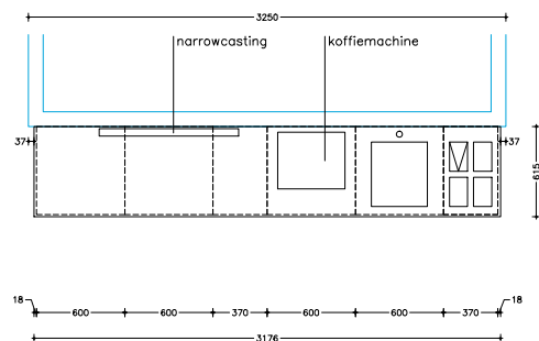
- boven aanzicht -
