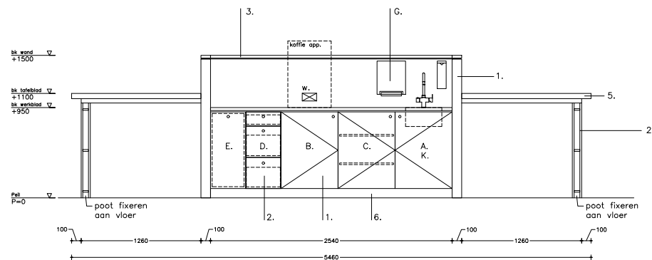
- voor aanzicht -
