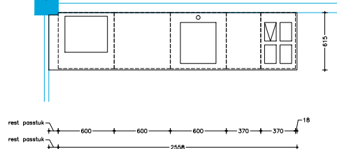
- boven aanzicht -
