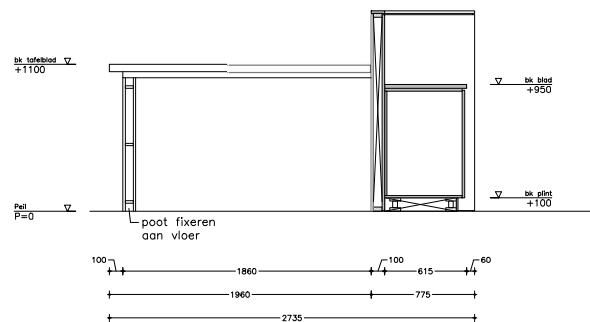
- verticale snede -
