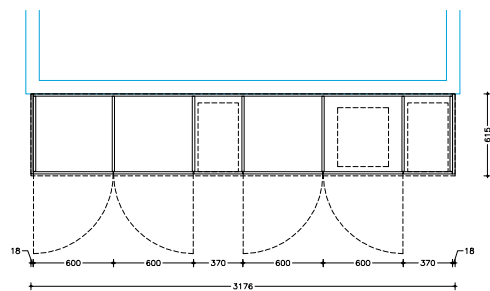
- horizontale snede -
