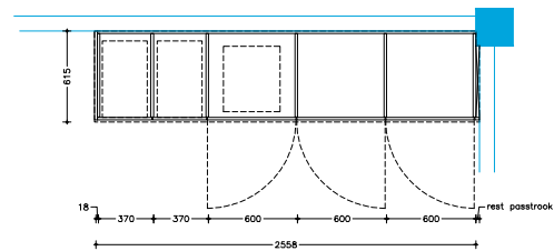
- horizontale snede -
