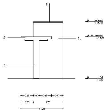
- zij aanzicht -
