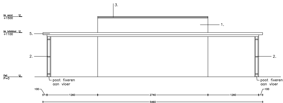
- achter aanzicht -
