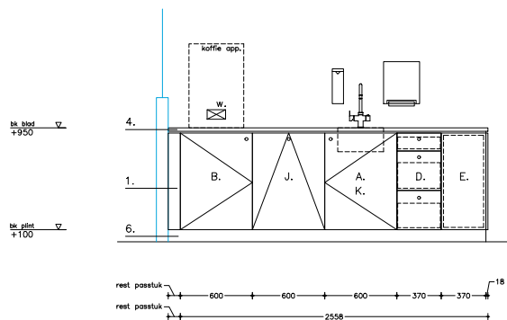
- voor aanzicht -
