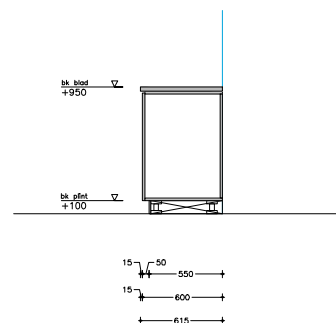
- verticale snede -
