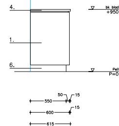
- zij aanzicht -
