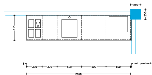
- boven aanzicht -
