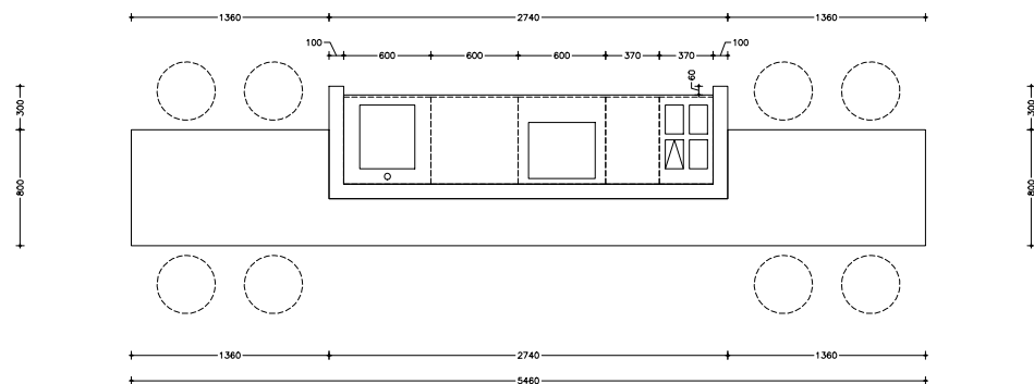
- boven aanzicht -
