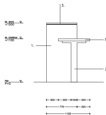
- zij aanzicht -
