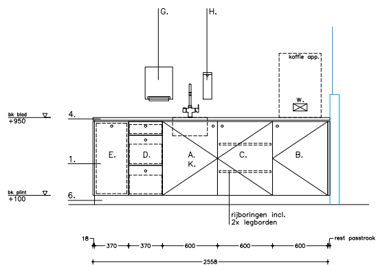
- vooraanzicht -
