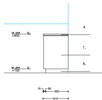
- zij aanzicht -
