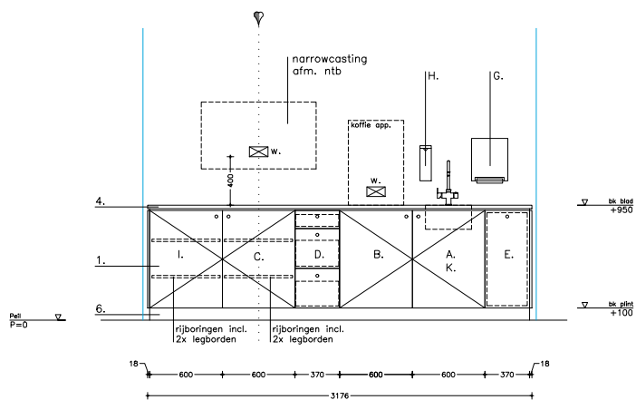
- voor aanzicht -
