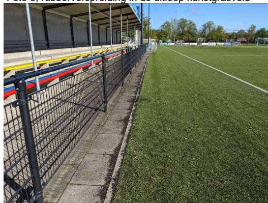
Foto 3; rubberverspreiding in de uitloop kunstgrasveld
