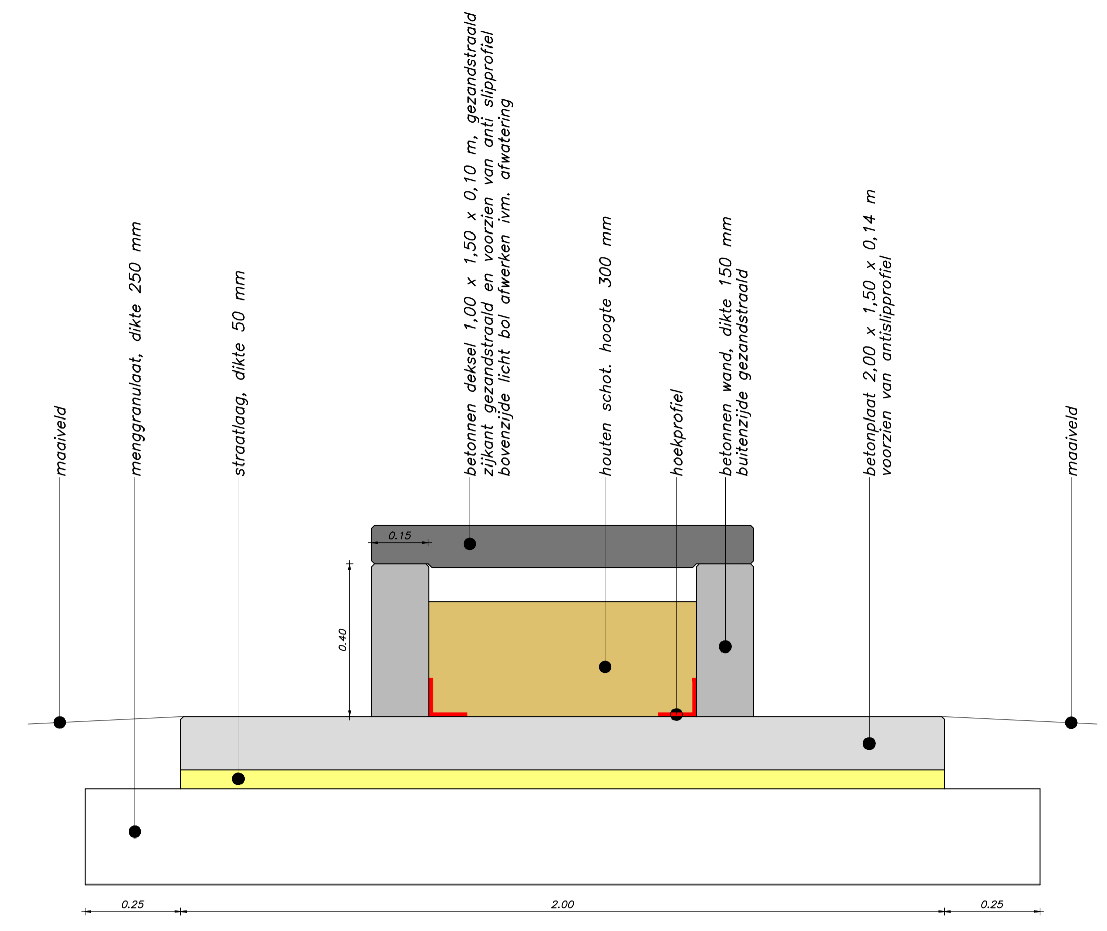
Dwarsprofiel plint Schaal 1:10
