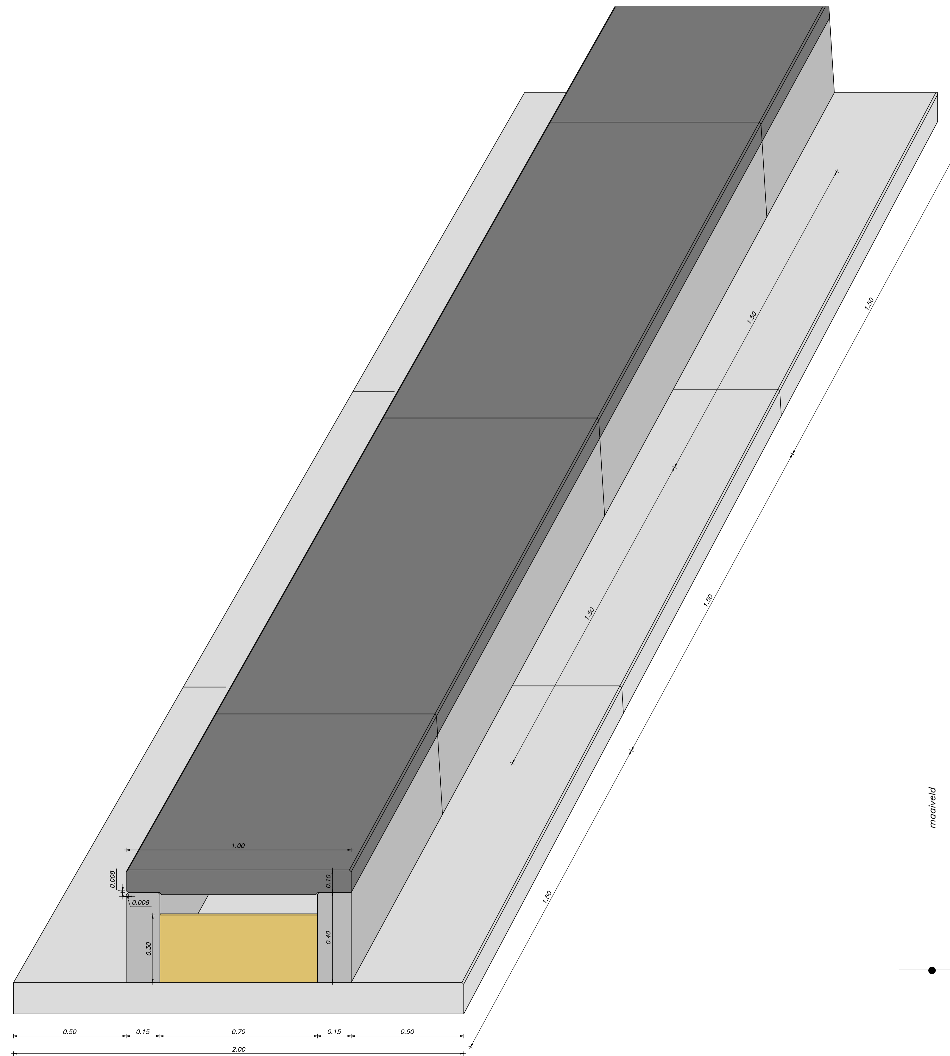
Principe3D aanzicht plint Schaal 1:10
