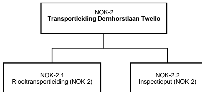
Figuur 3.2 Objectenboom
