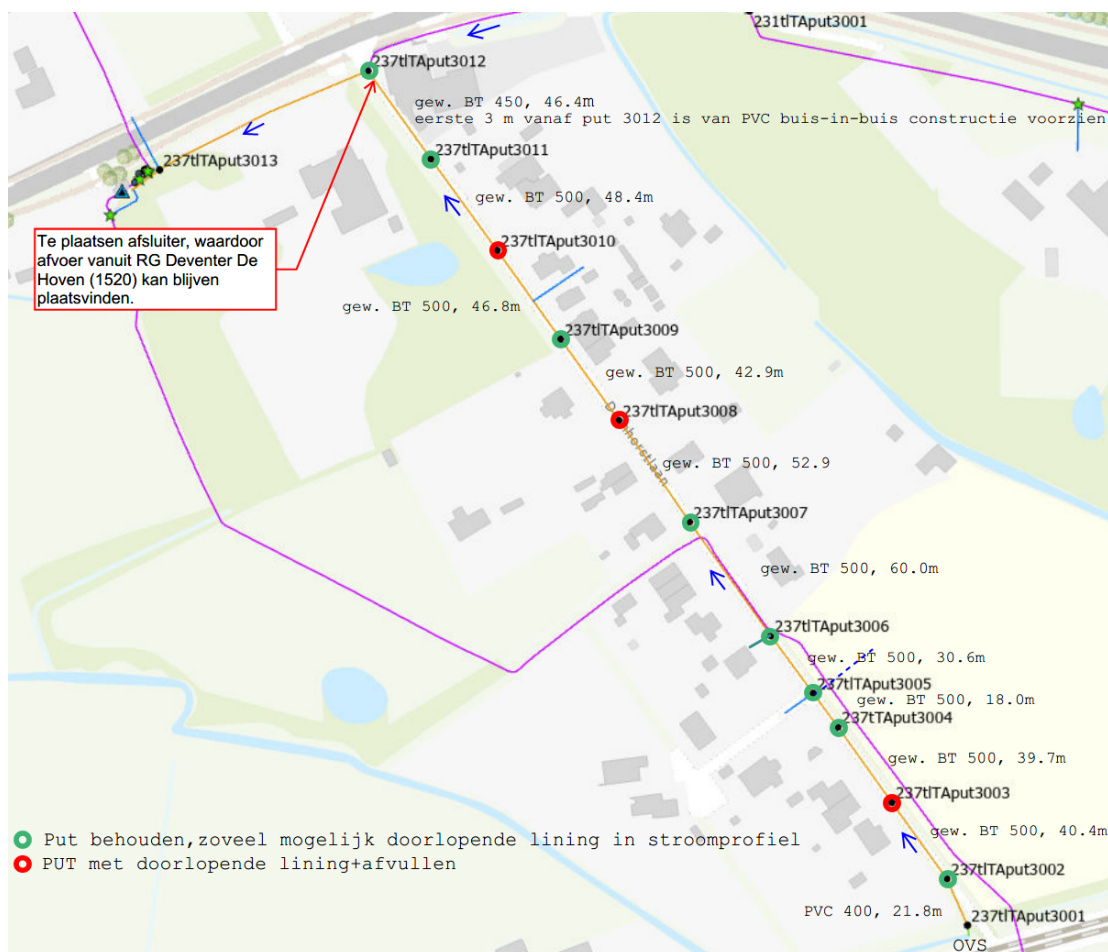
Figuur 2.1 Riooltransportleiding Dernhorstlaan Twello
