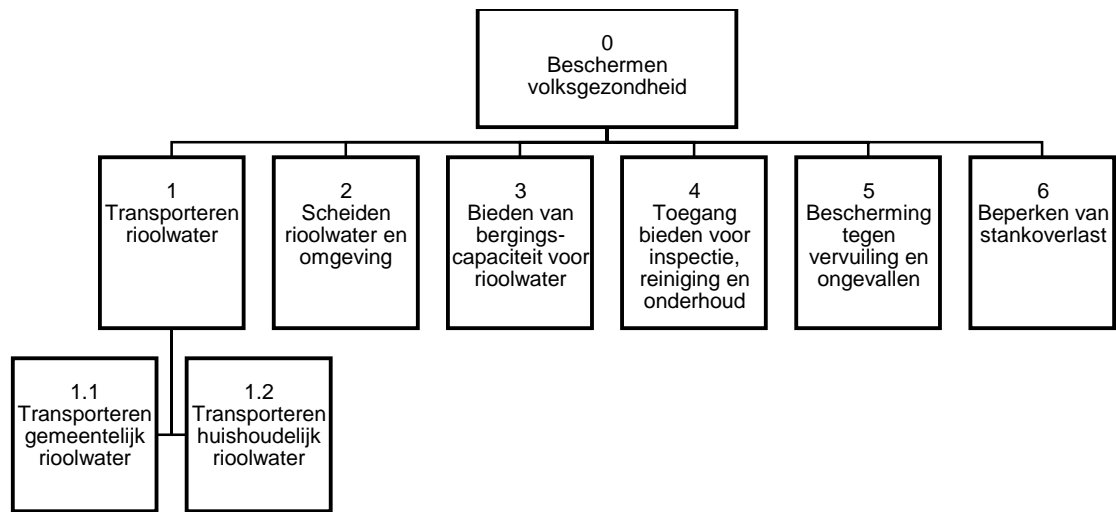
Figuur 3.1 Functieboom
