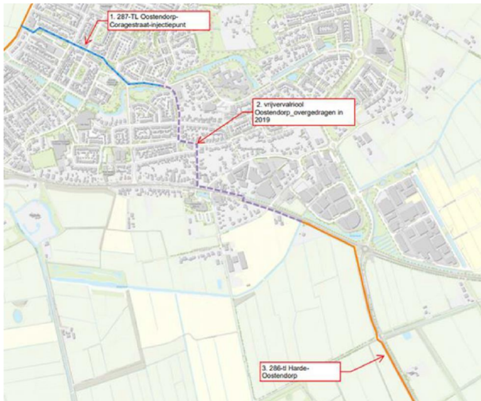
Figuur 2.1 Riooltransportleiding 't Harde - Oostendorp
