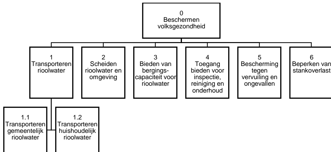
Figuur 3.1 Functieboom
