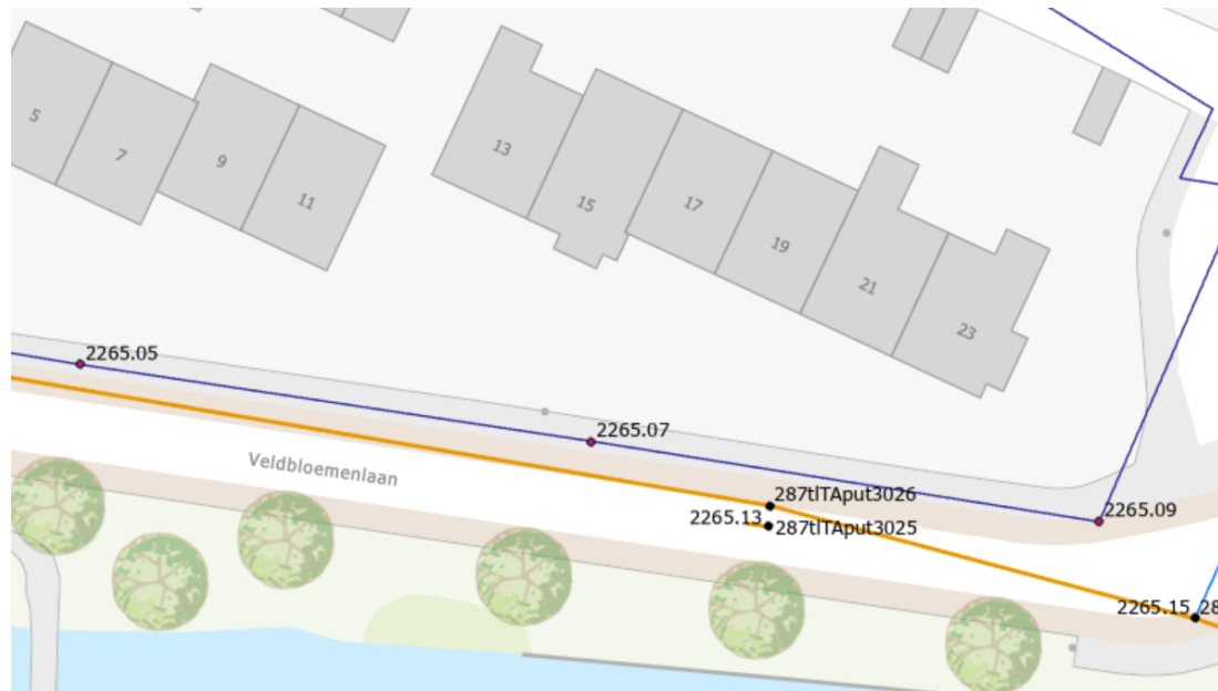
Figuur 2.3 De overstortmuur in put 287tITApot3026 stort over in put 287tITApot3025. (Nummering beginnend met 2265.xx is de nummering zoals aangehouden door gemeente Elburg).
