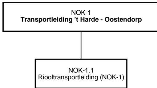
Figuur 3.2 Objectenboom
