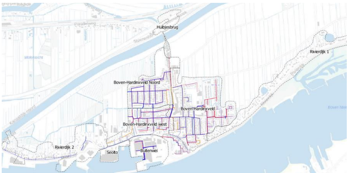
Figuur 5.2 Vrijverval riolering Boven-Hardinxveld (bron: Sweco)
