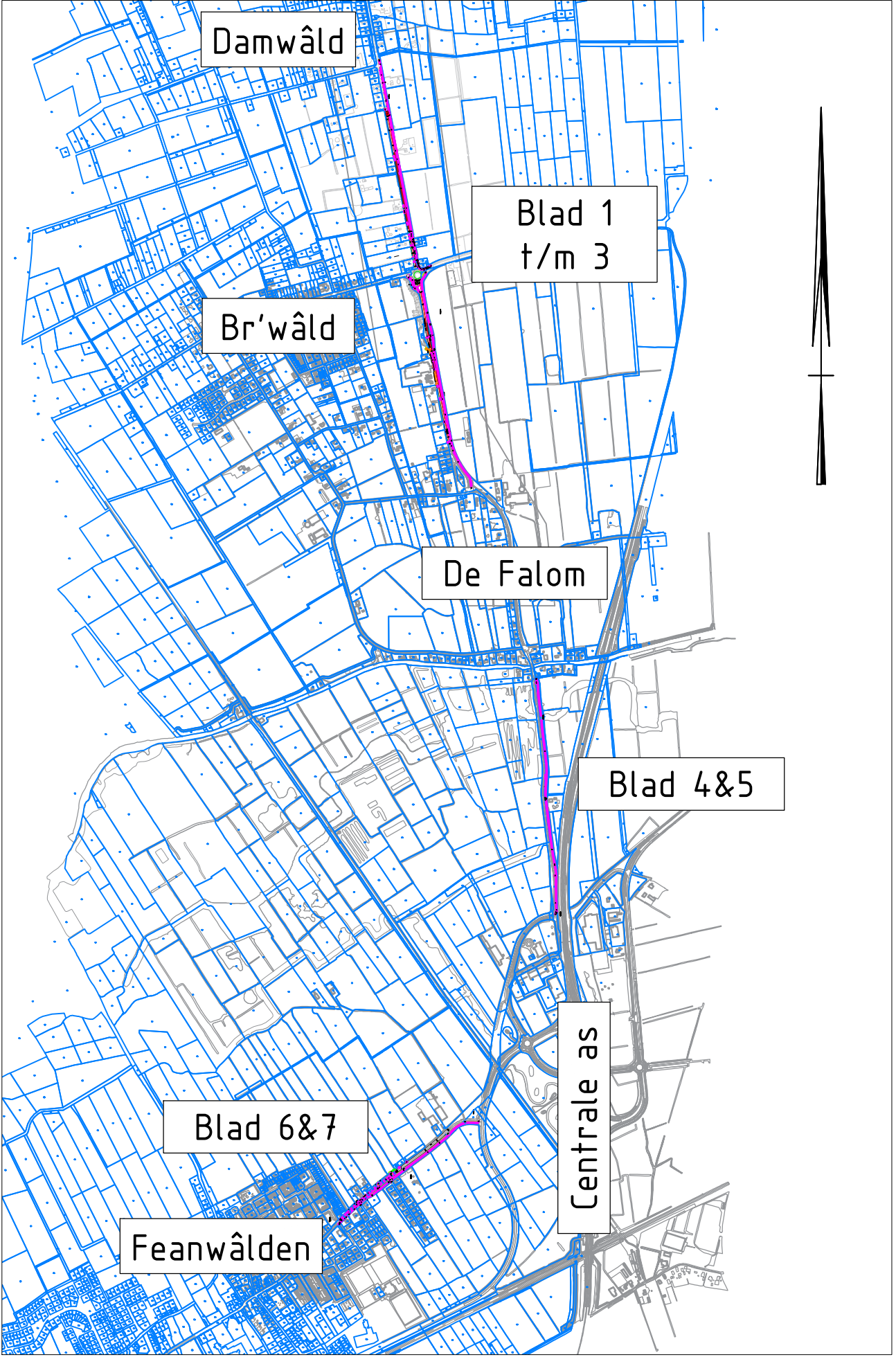
Overzichtstekening SCHAAL 1 : 2000
