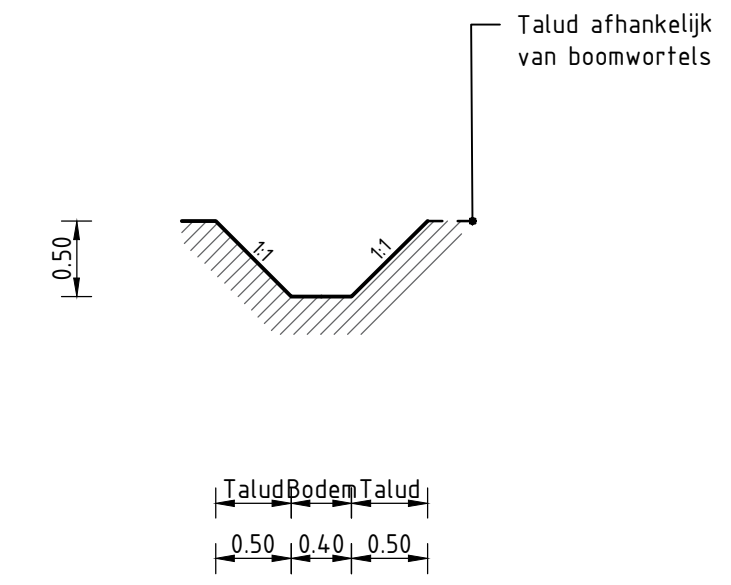
UITSNEDE C-C': Dwarsprofiel afvoergreppel Schaal 1:50
