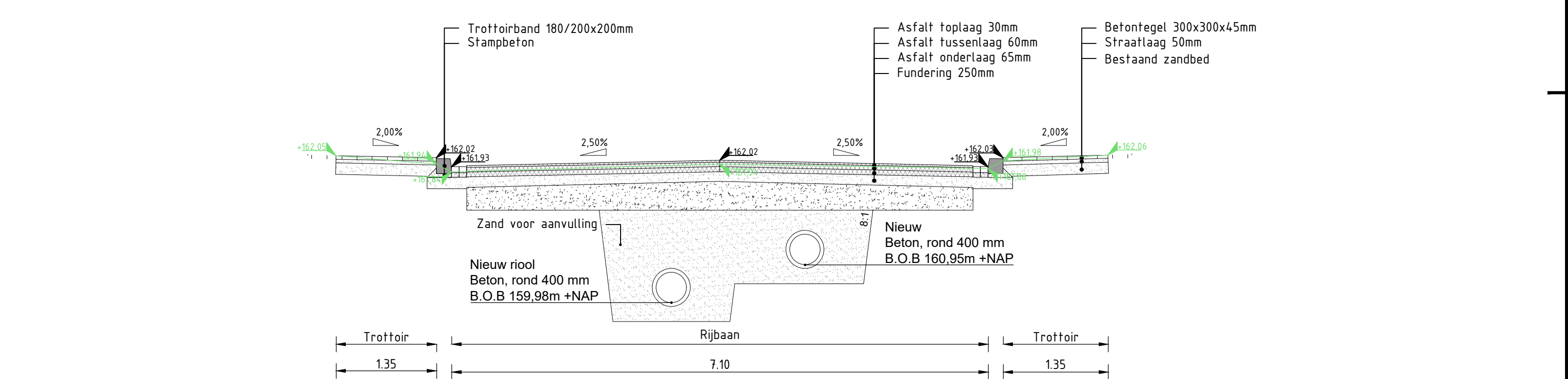
UITSNEDE A-A': Dwarsprofiel Stevensweg Schaal 1:50
