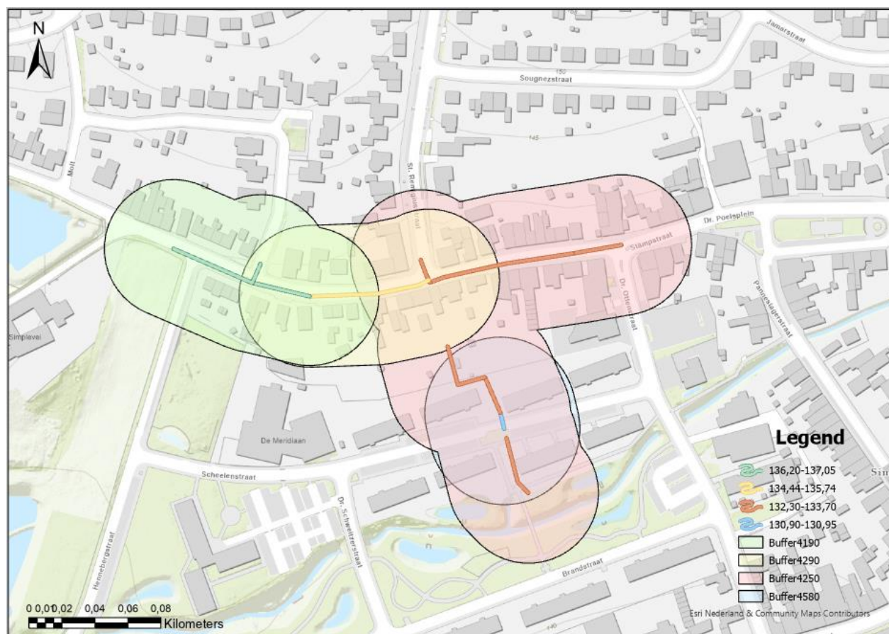
Figuur 4-1: Invloedsgebied (invloed < 5 cm) in de omgeving stampstraat (freatisch)
