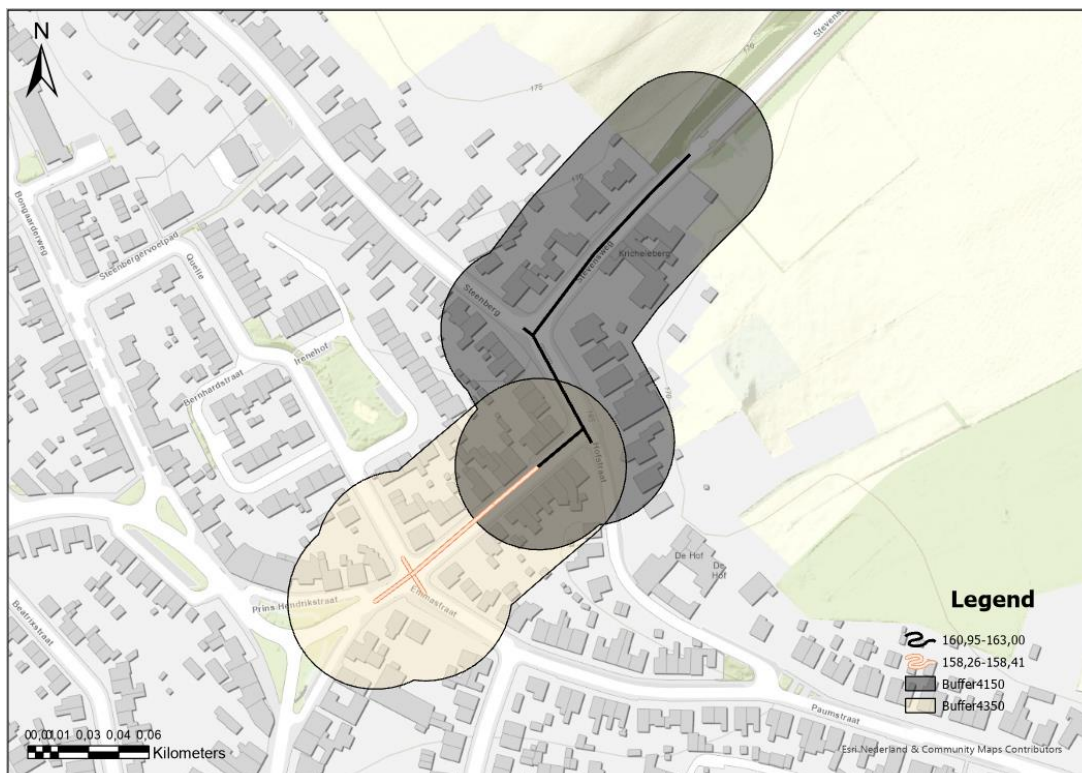
Figuur 4-3: Invloedsgebied (invloed < 5 cm) in de omgeving Stevenweg (freatisch)
