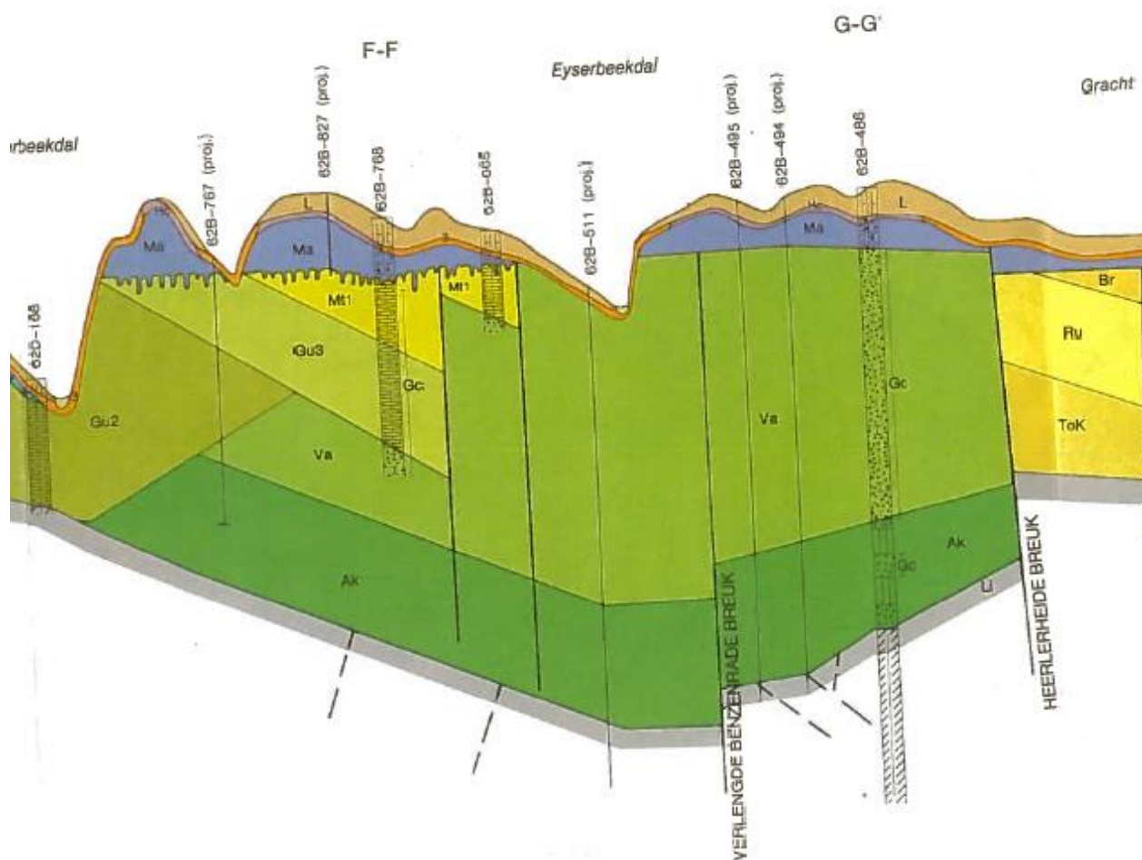
Figuur 3-2: Doorsnijing formatie Maastricht (Ma) in Eyserbeekdal
