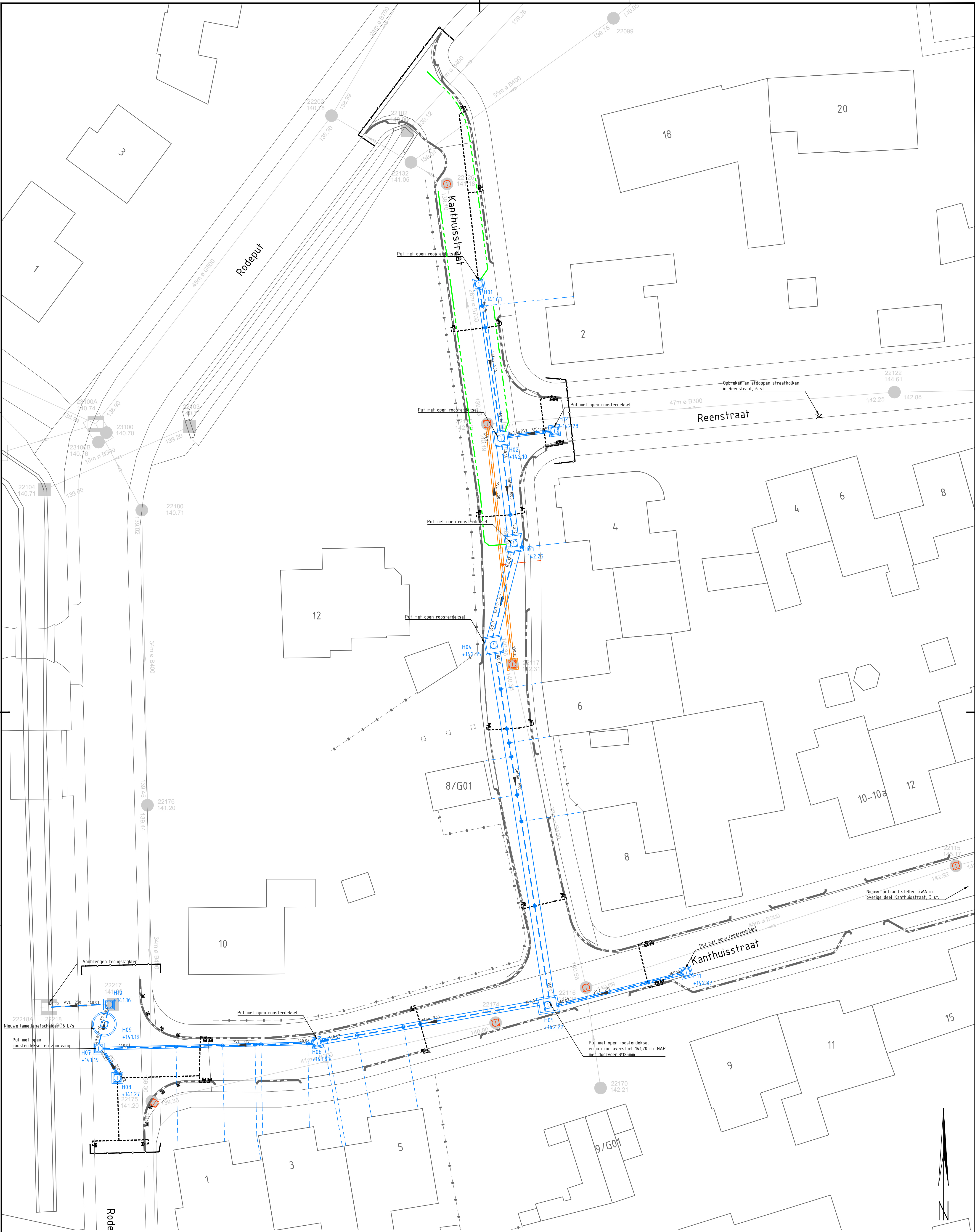
SITUATIE Herinrichting Kanthuisstraat Schaal 1:200
