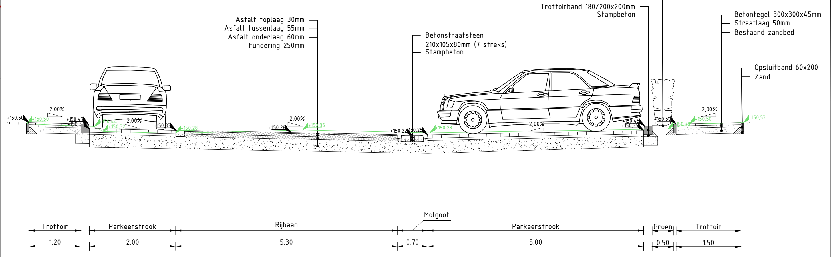
UITSNEDE A-A': Dwarsprofiel Punstelstraat Schaal 1:50
