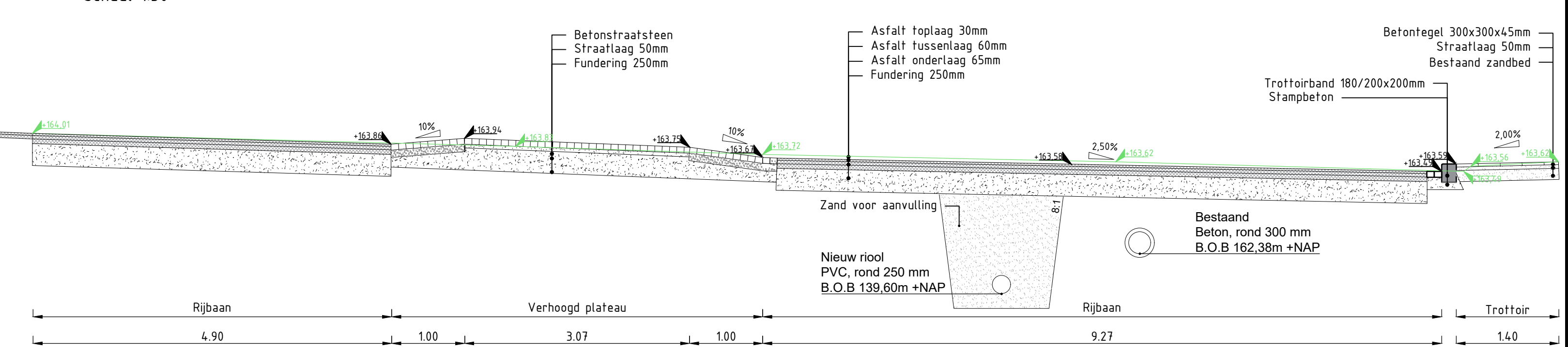
UITSNEDE A-A': Dwarsprofiel Stevensweg Schaal 1:50
