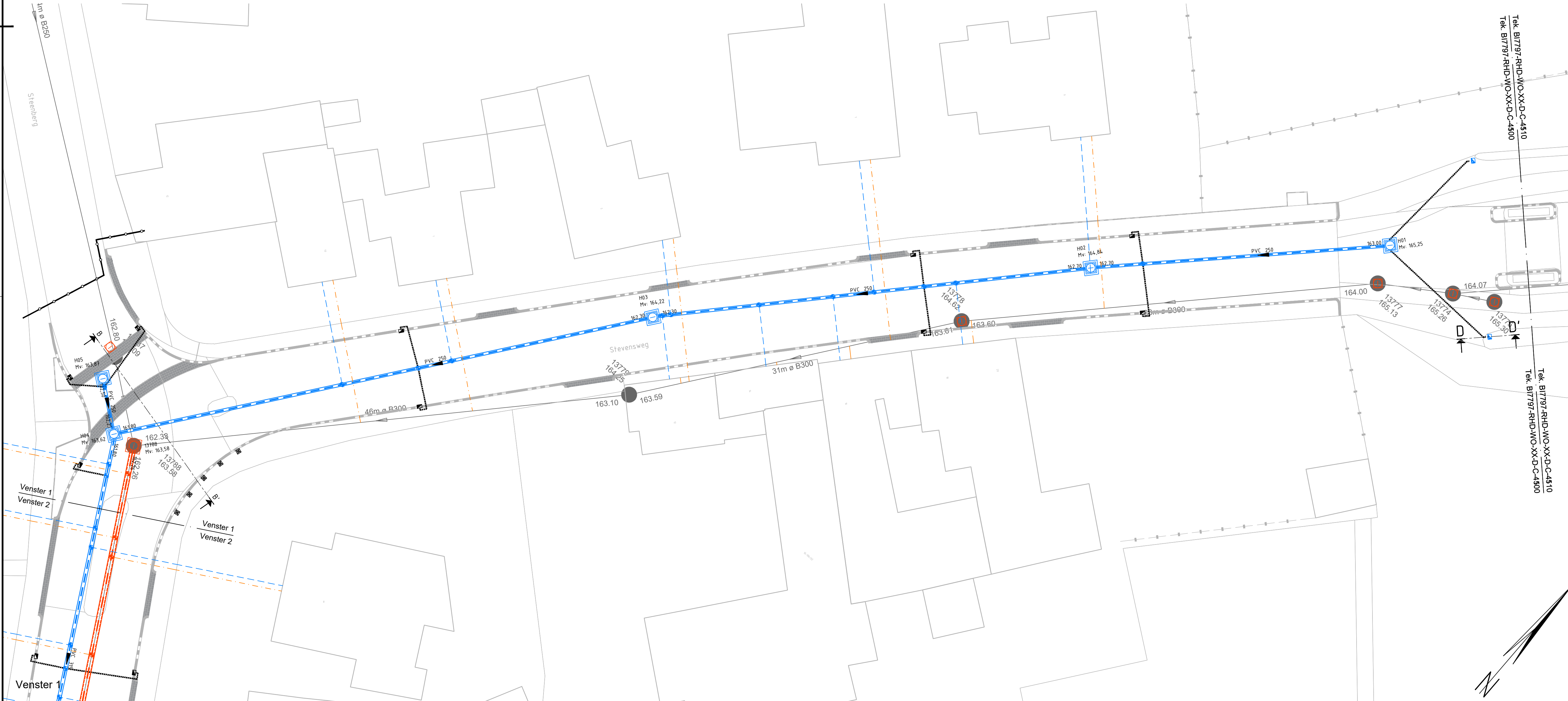
Stevensweg (kruispunt Steenberg t/m komgrens) Schaal 1:200
