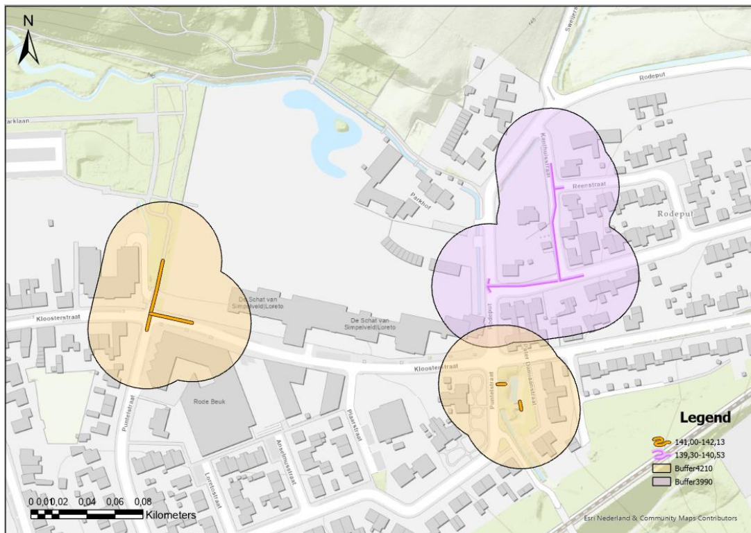
Figuur 4-2: Invloedsgebied (invloed < 5 cm) in de omgeving kanthuisstraat en puntelstraat (freatisch)
