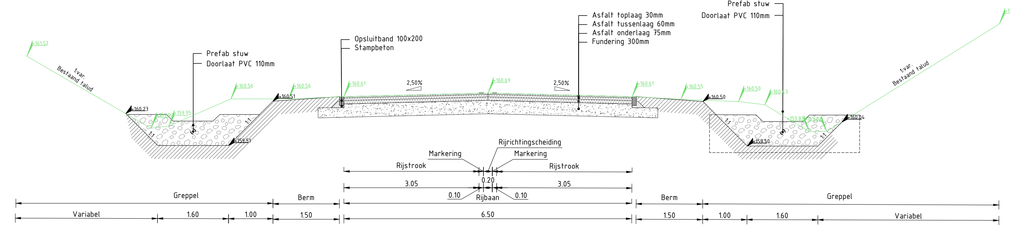
UITSNEDE C-C': Dwarsprofiel Nijswillerweg Schaal 1:50
