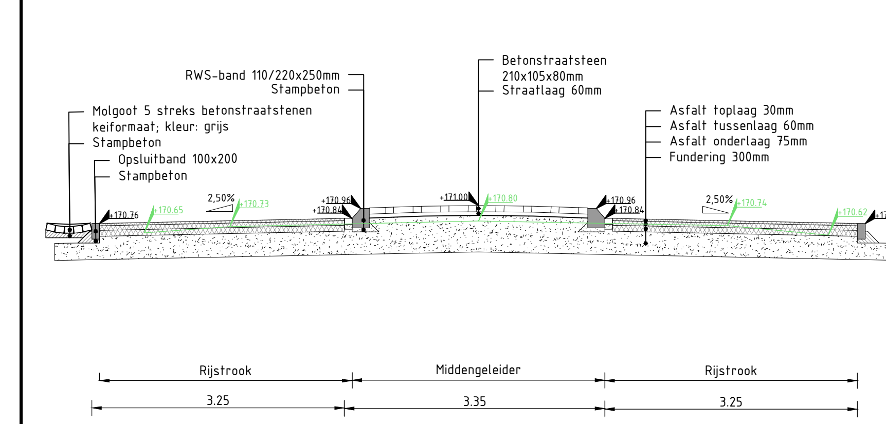
UITSNEDE B-B': Dwarsprofiel Middengedeelte Nijswillerweg Schaal 1:50
