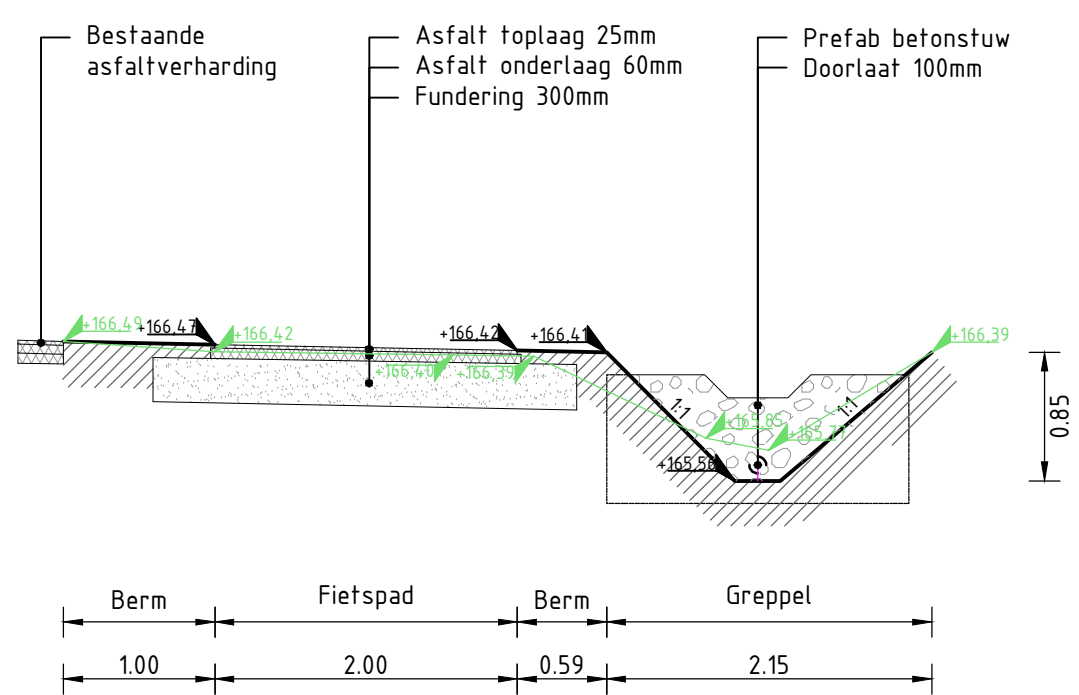
UITSNEDE C-C: Dwarsprofiel vrijliggend fietspad Schaal 1:50
