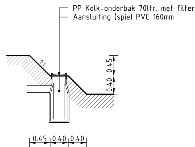
UITSNEDE D-D: Dwarsprofiel stokop greppel Schaal 1:50
