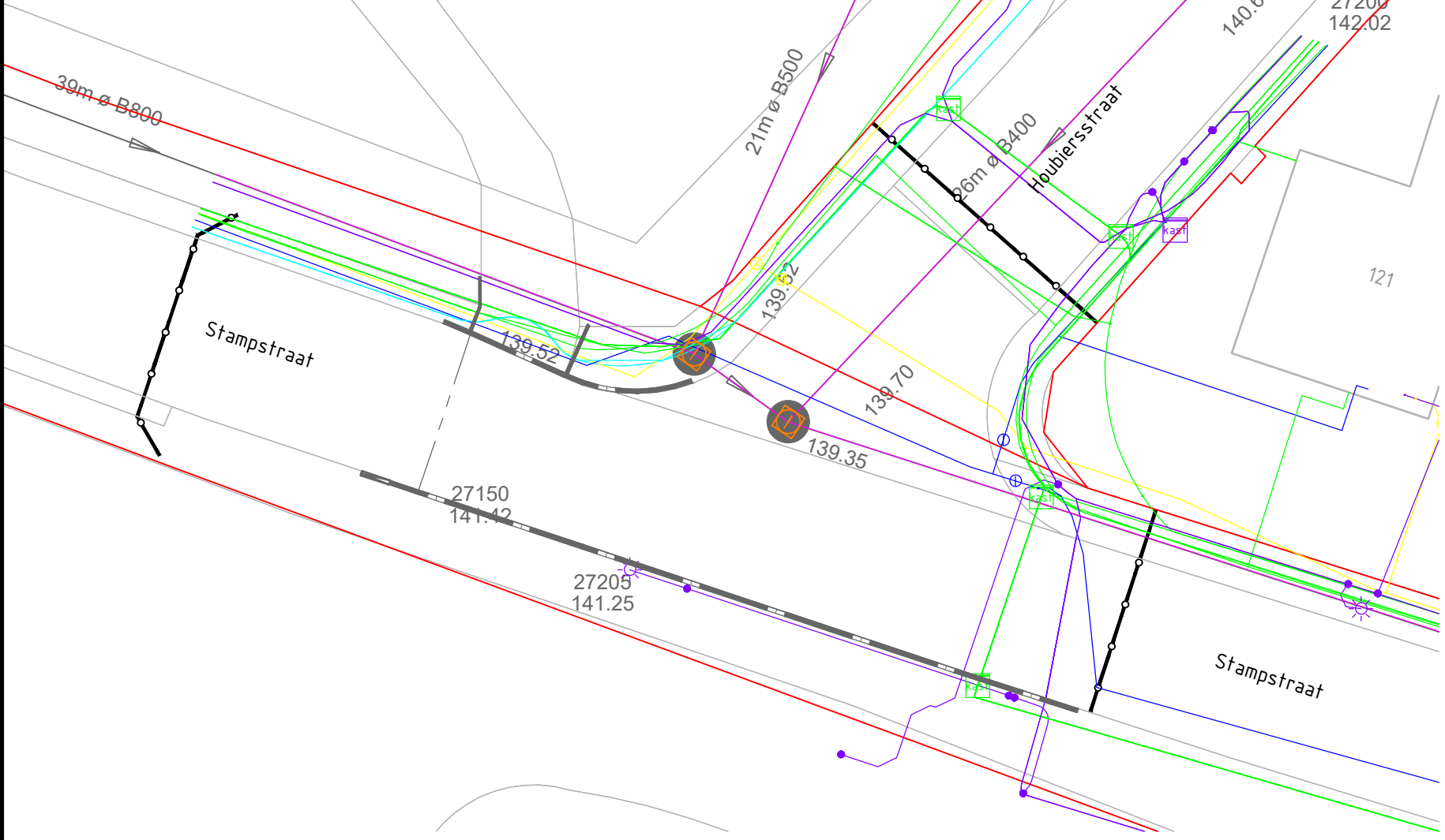
Stampstraat (kruispunt Houbiersstraat) Schaal 1:200
