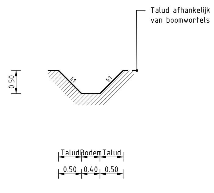
UITSNEDE C-C': Dwarsprofiel afvoergreppel Schaal 1:50
