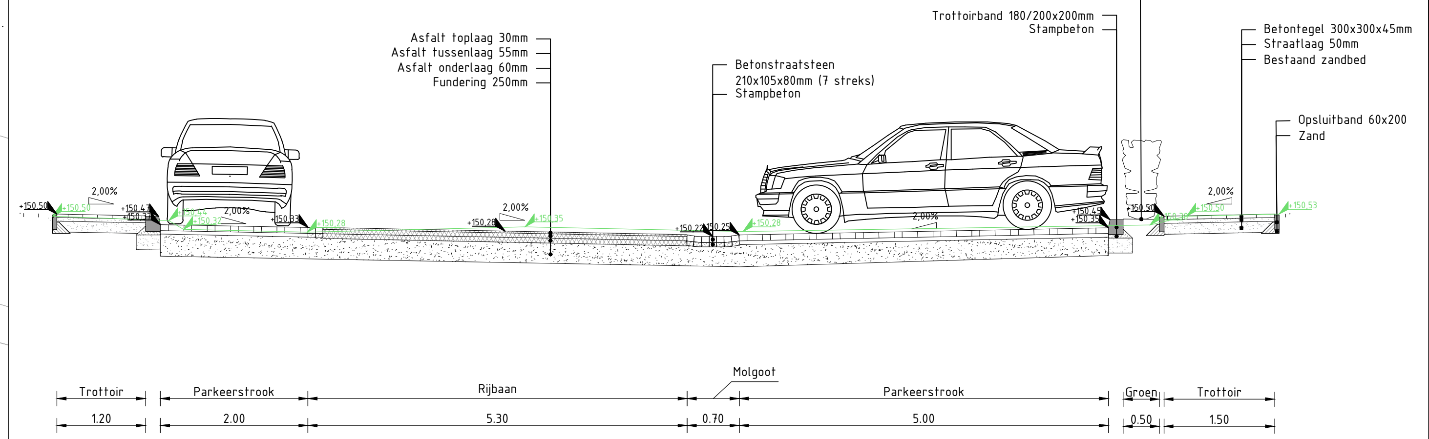
UITSNEDE A-A': Dwarsprofiel Puntelstraat Schaal 1:50
