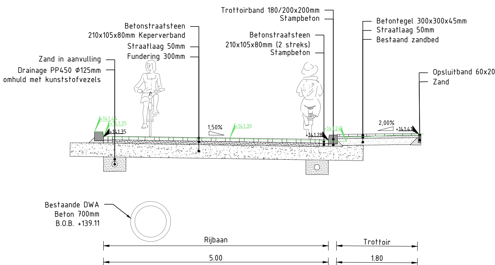
UITSNEDE B-B': Dwarsprofiel Kanthuisstraat Schaal 1:50
