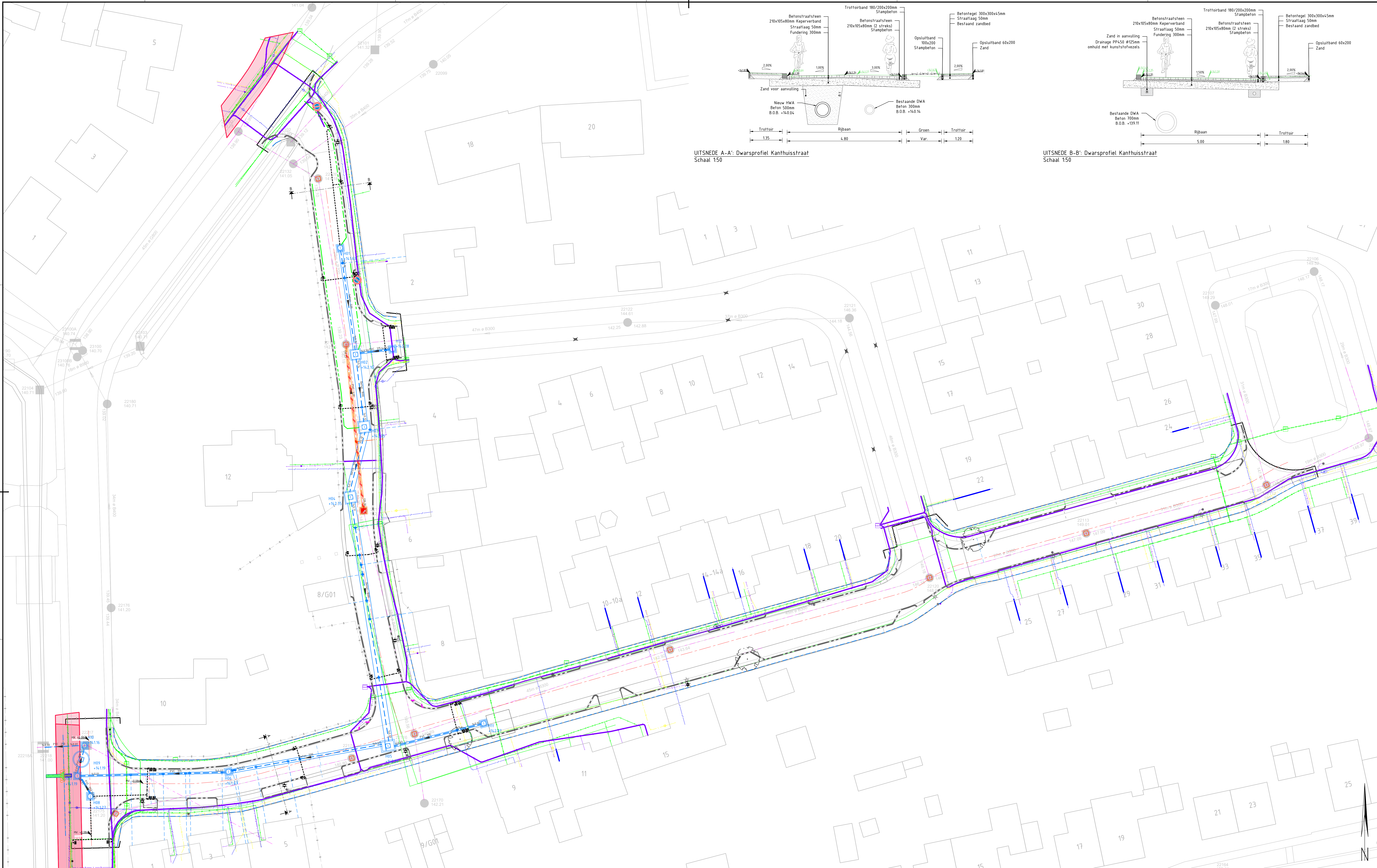
SITUATIE Herinrichting Kanthuisstraat Schaal 1:200
