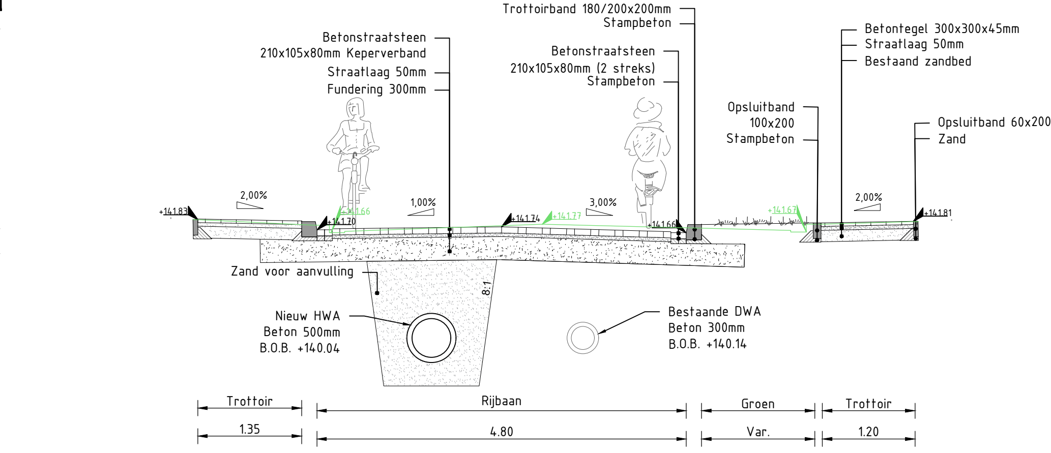
UITSNEDE A-A': Dwarsprofiel Kanthuisstraat Schaal 1:50
