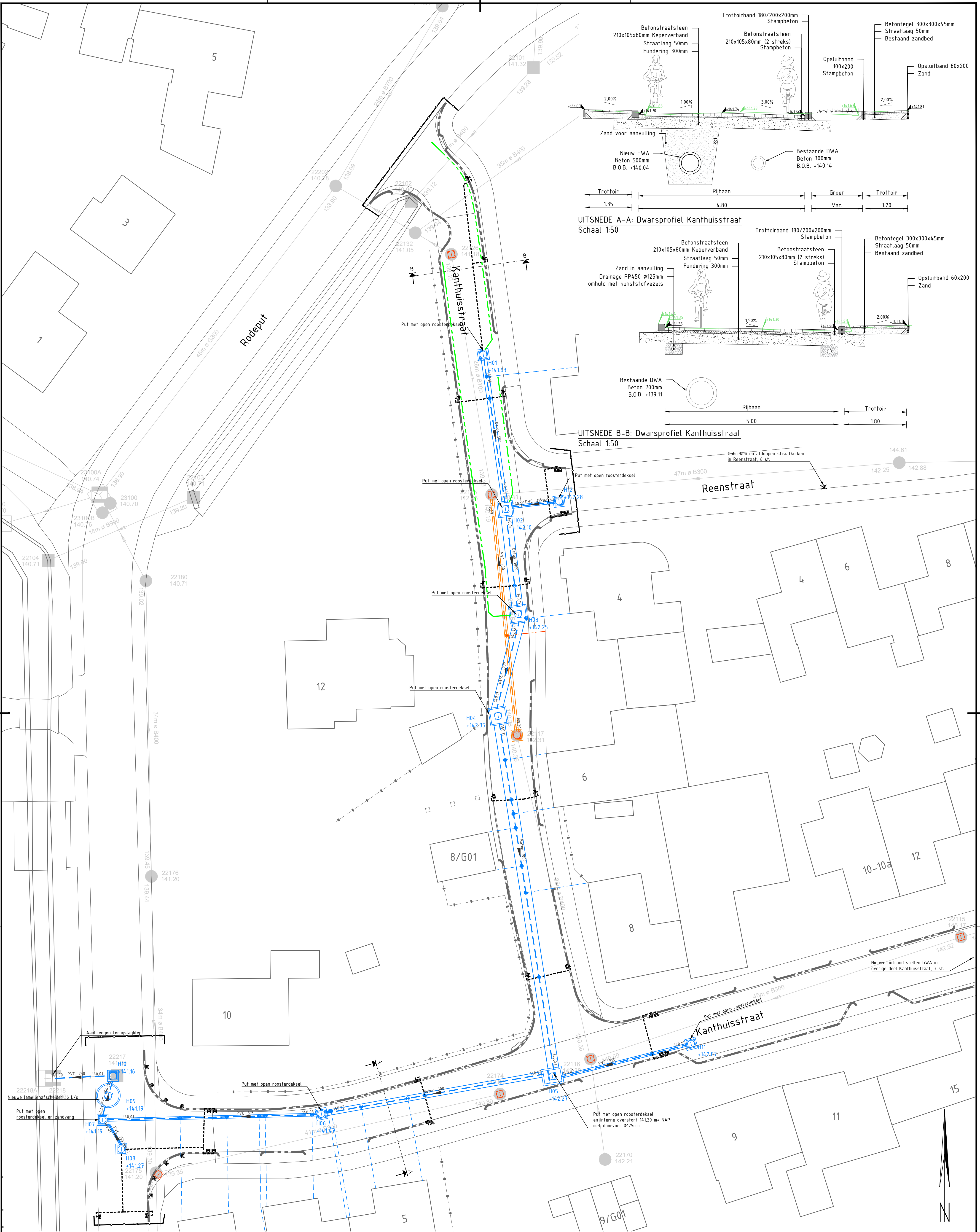
SITUATIE Herinrichting Kanthuisstraat Schaal 1:200
