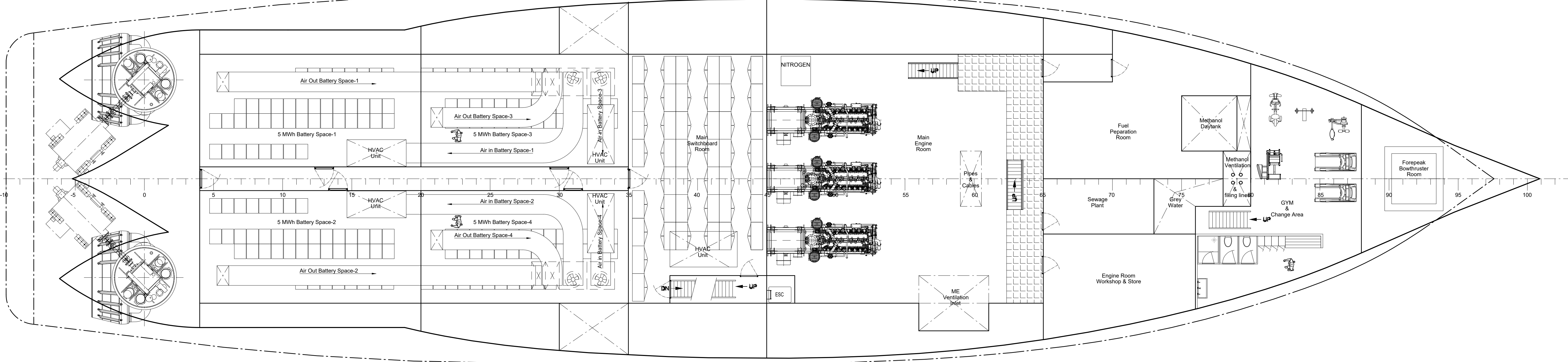
5700 A.B. - TWEEN DECK
