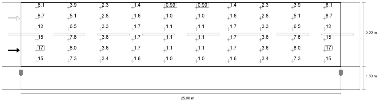
Onderhoudswaarde horizontale verlichtingssterkte [lx] (Waardenraster)
