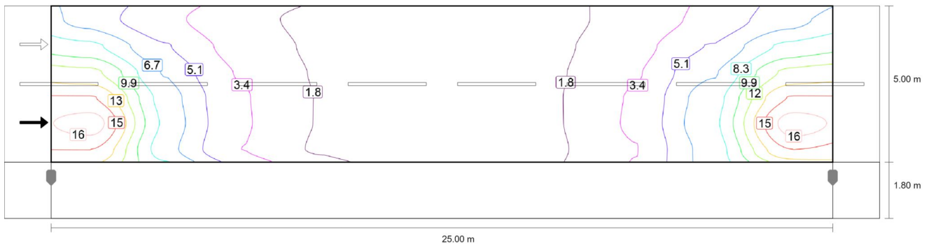
Onderhoudswaarde horizontale verlichtingssterkte [lx] (Isoluxlijnen)
