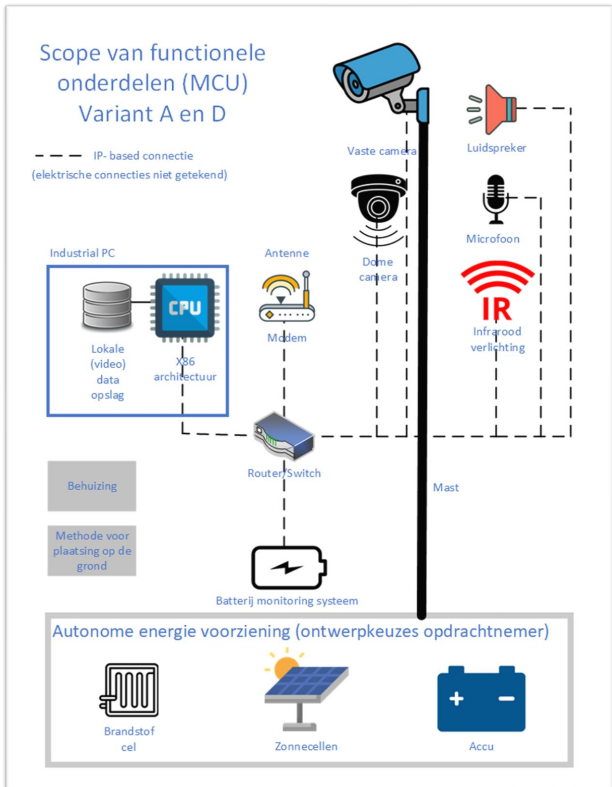
Afbeelding 1 – Functioneel overzicht variant A & D
