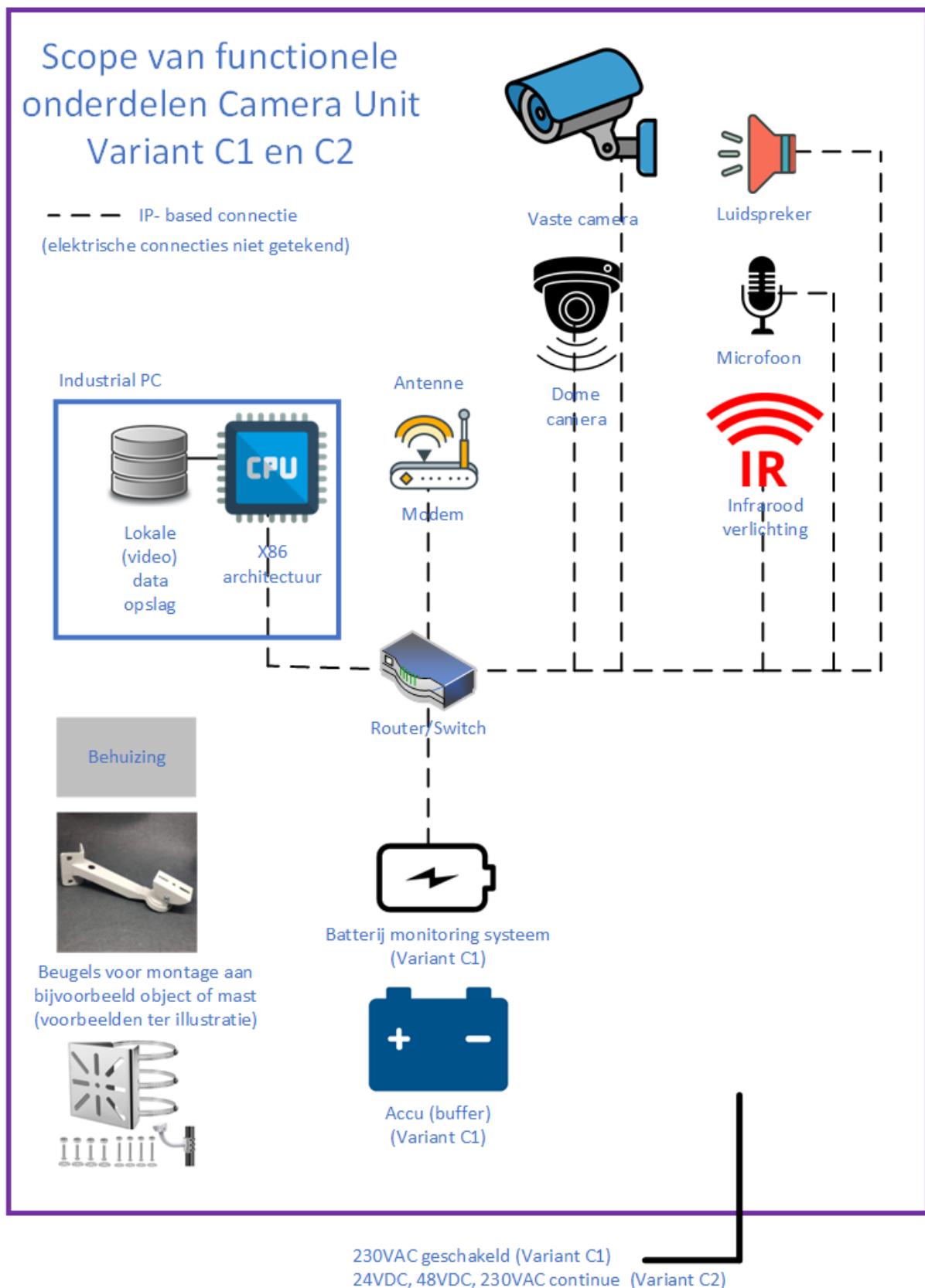
Afbeelding 3 – Functioneel overzicht variant C1 en C2
