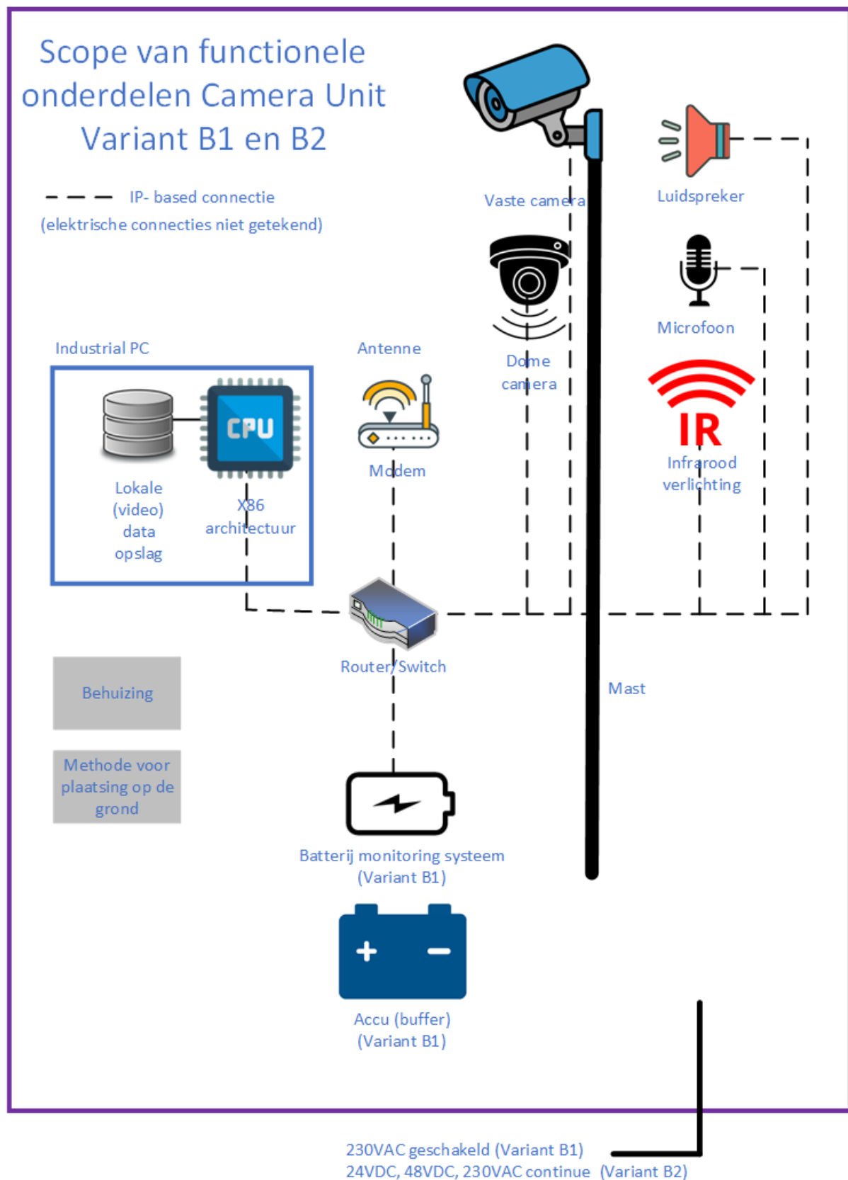
Afbeelding 2 – Functioneel overzicht variant B1 en B2
