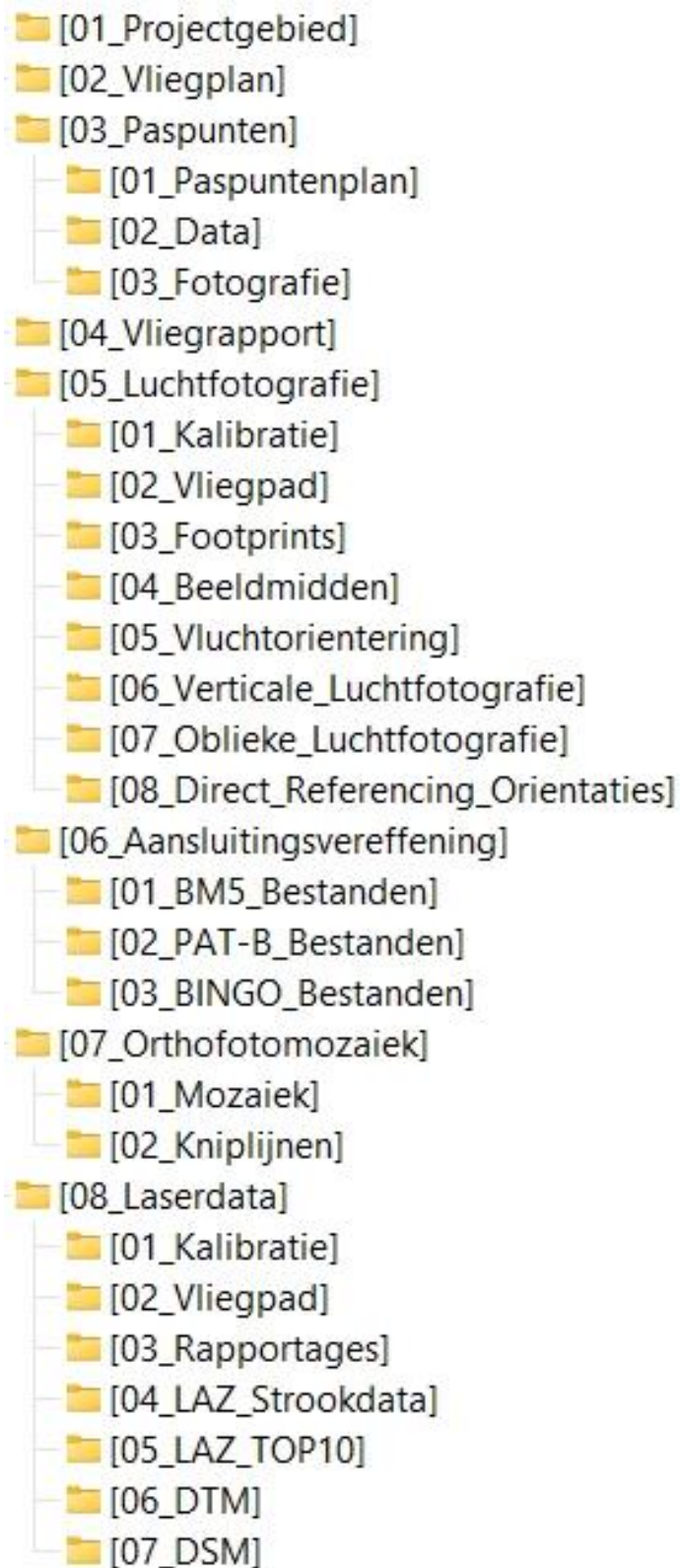
Figuur 2: Mappenstructuur.
