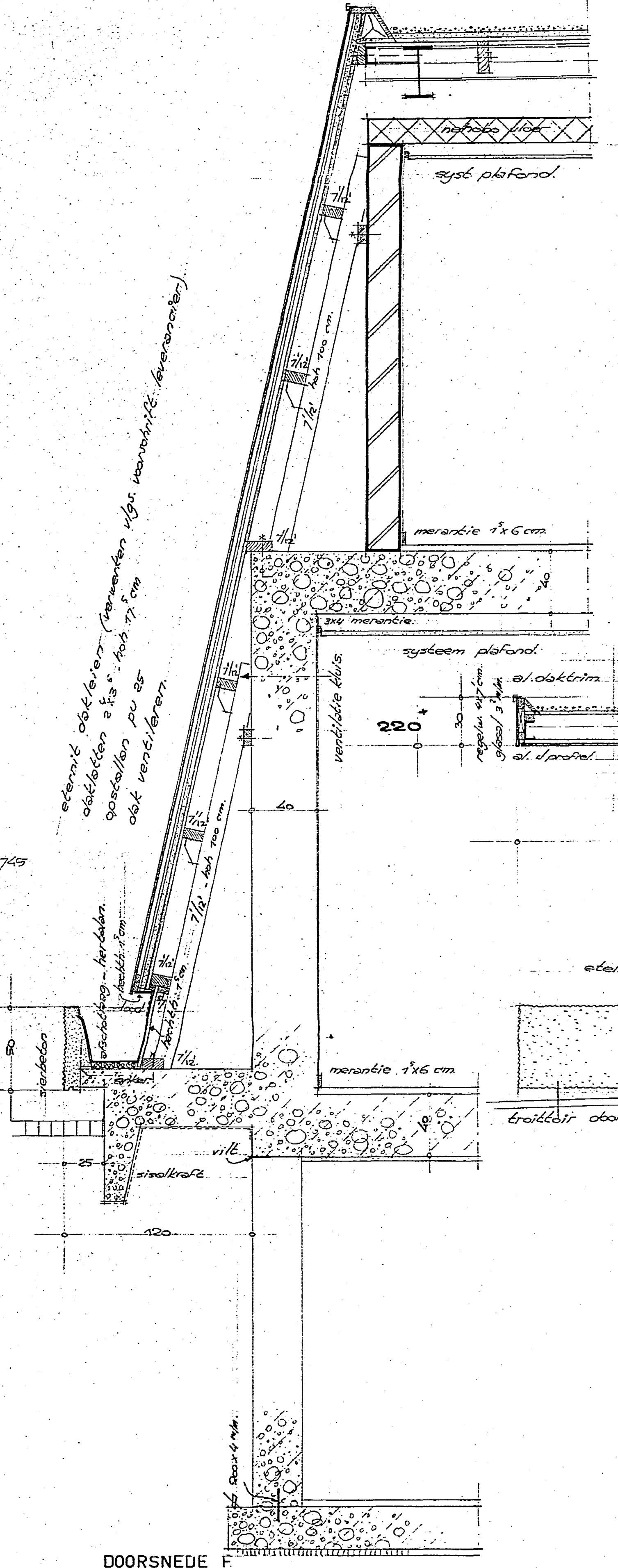
DOORSNEDE F
