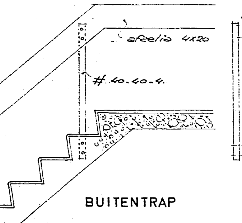
TRAP VERTREK 18
