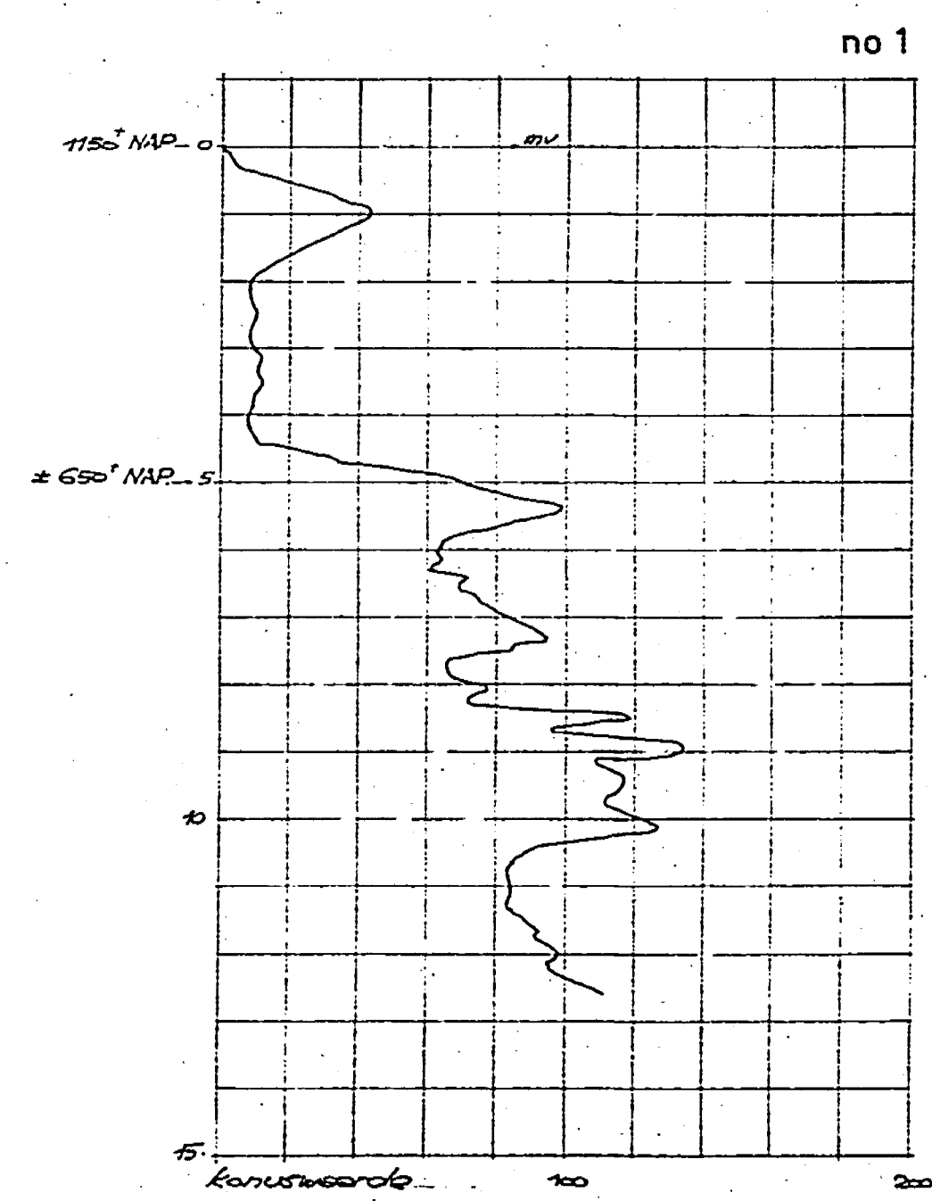
SONDEERGRAFIKEN
