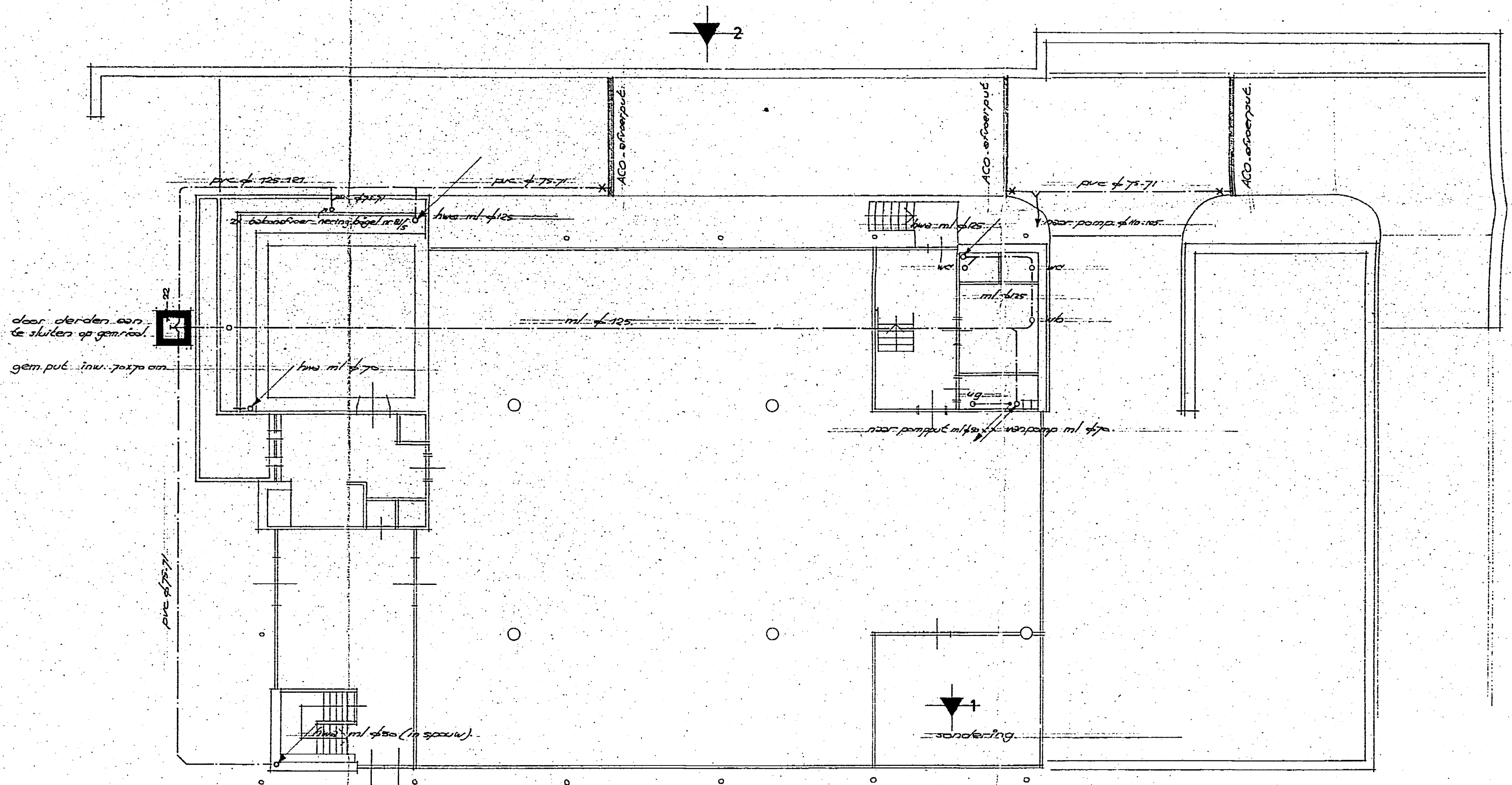
BEGANE GROND
