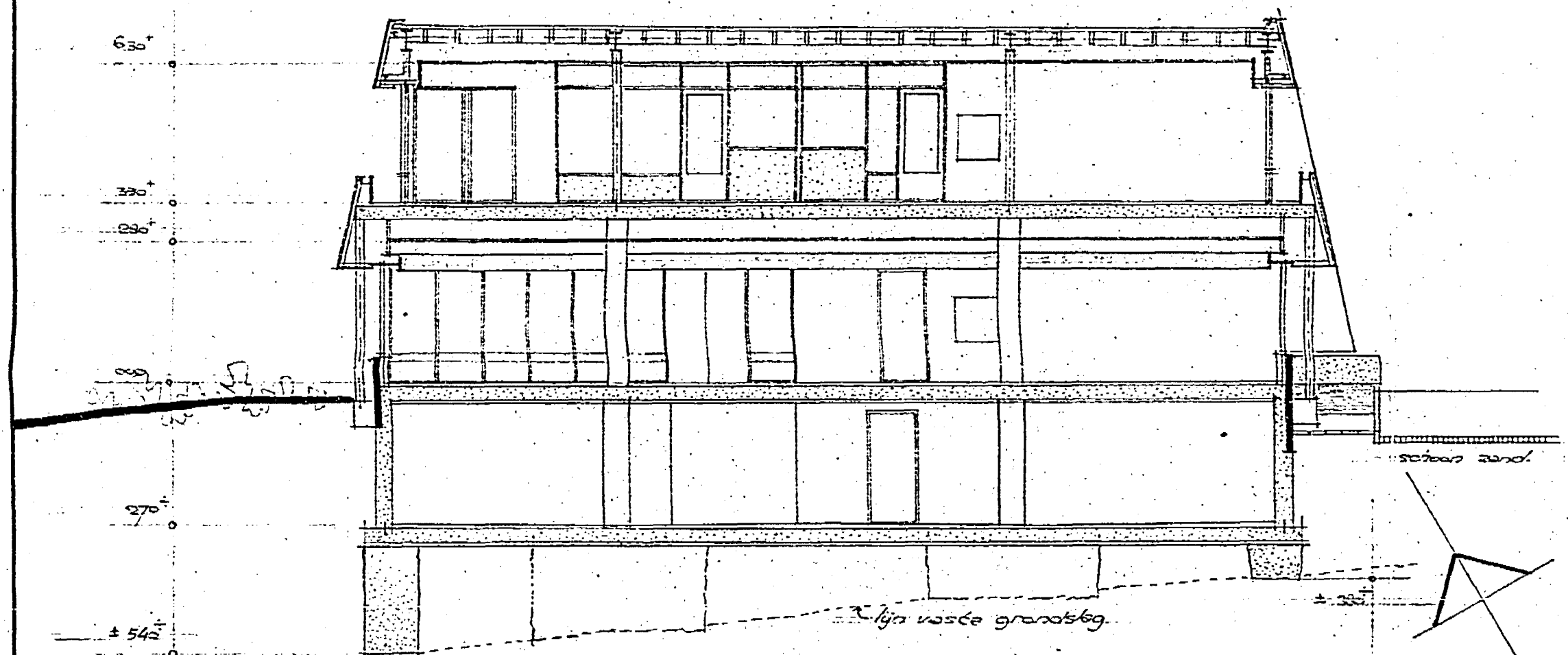
DOORSNEDE A-B
