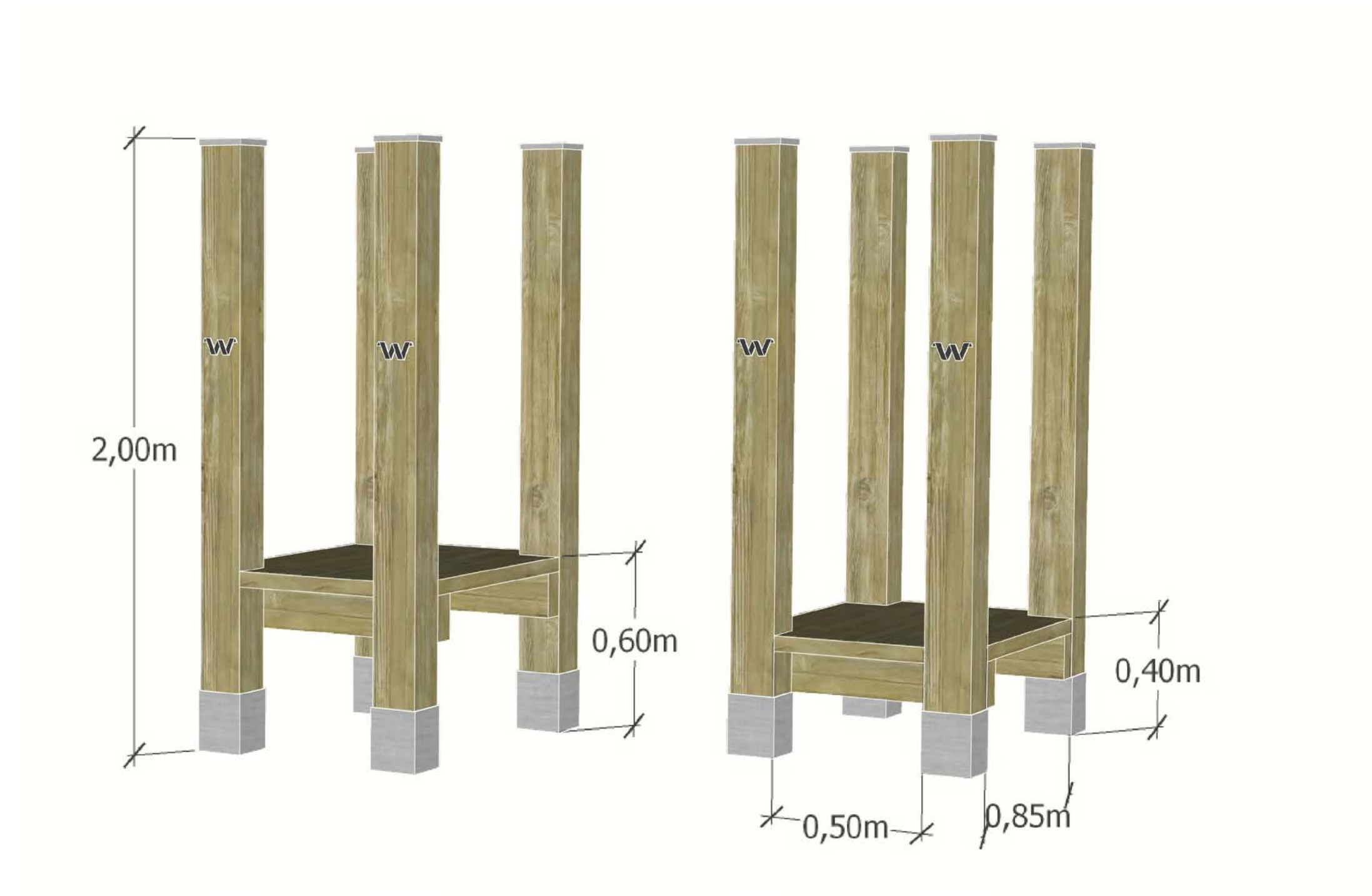
plateau voor het klimparcours
