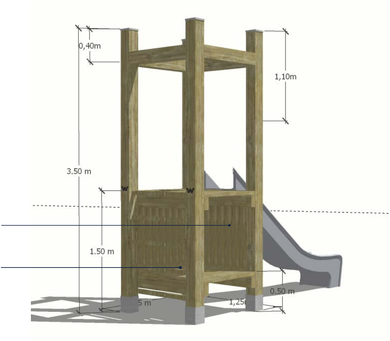
speelhuisje met glijbaan (achterzijde)
