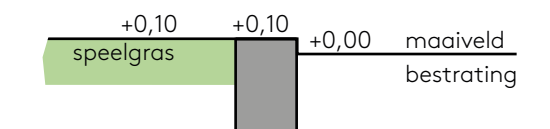
principe opsluitband/betonnen rand
