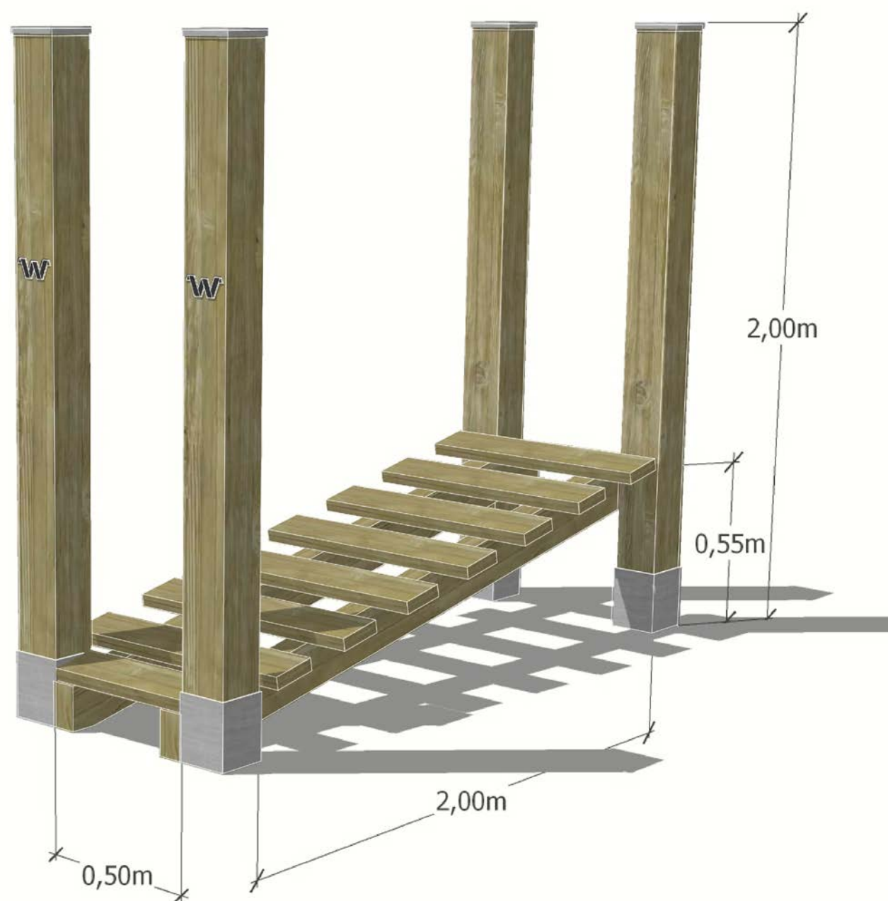
voorbeeld van een bevestigingsonderdeel: trap
