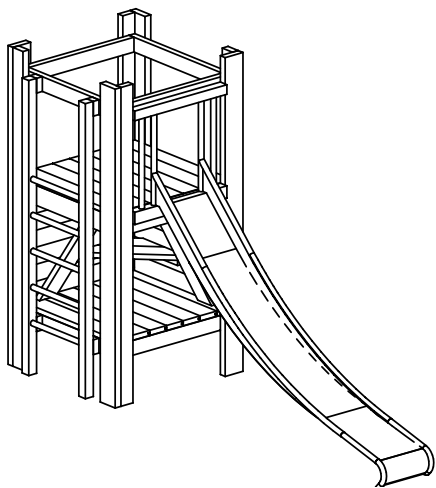
A: Huttencombinatie 320 (2.13200) met kabelladder 1 platformhut met ladder, 1 smalle glijbaan H 1,5 m, kabelladder (3.69410)
