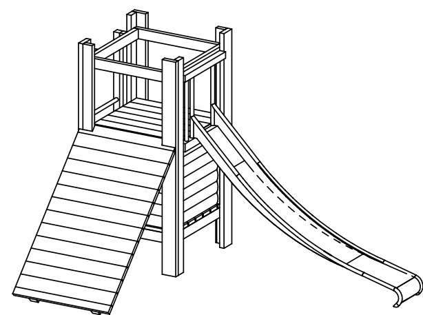
A: Huttencombinatie 216 (212160) platformhut zonder dak (H 2,5 m), glijbaan (H 1,5 m), schuine wand (H 1,5 m), ladder
