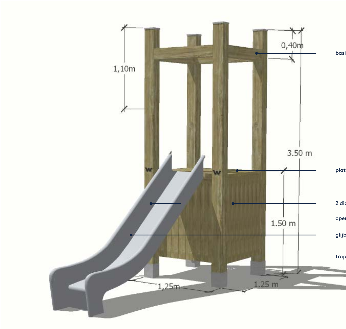
speelhuisje met glijbaan (voorzijde)
