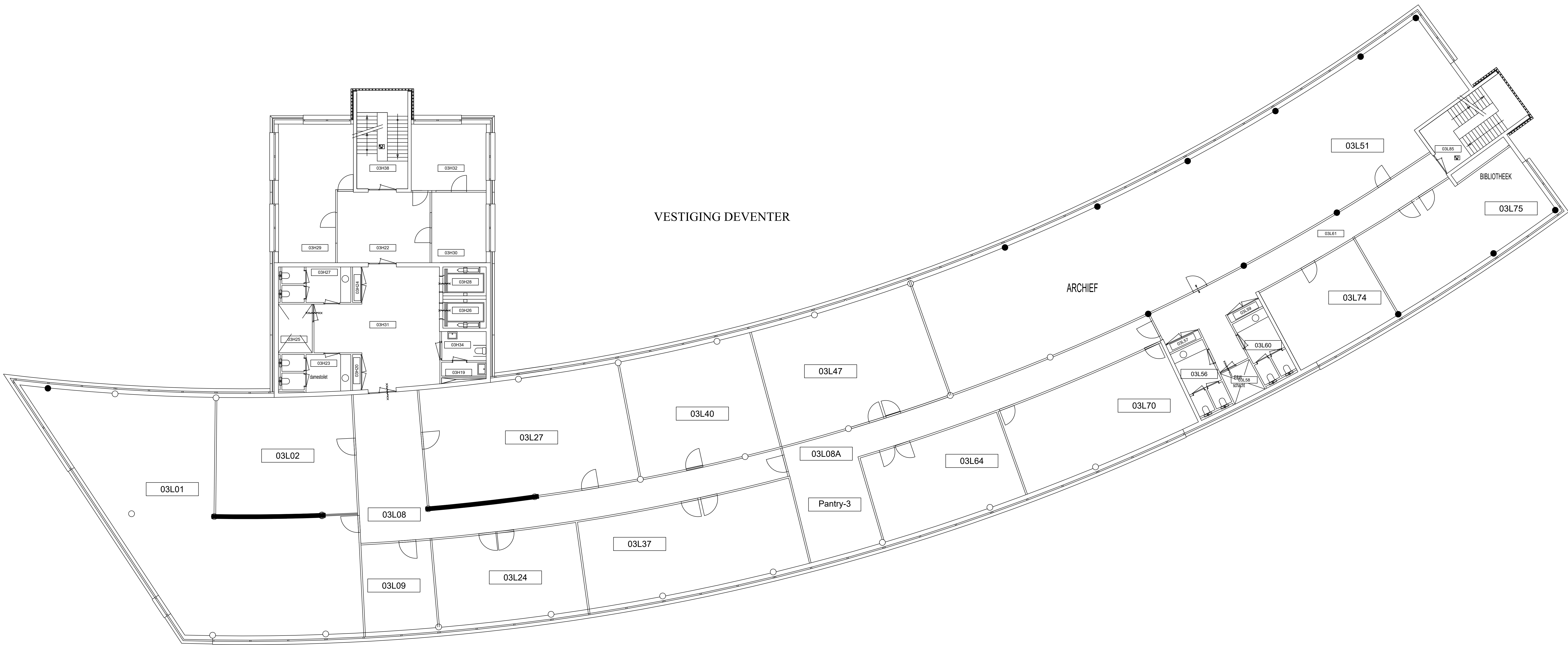
3e Verdieping
