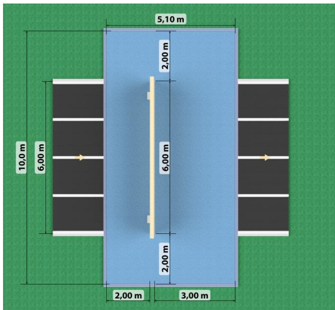
Bovenaanzicht en maatvoering
