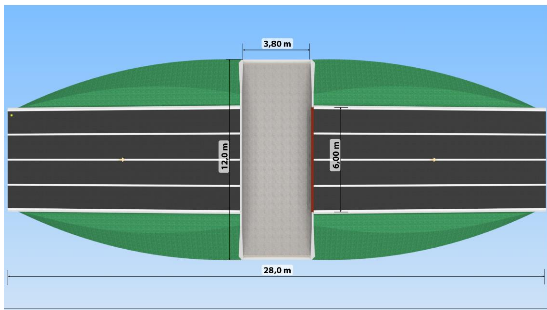
Bovenaanzicht en maatvoering
