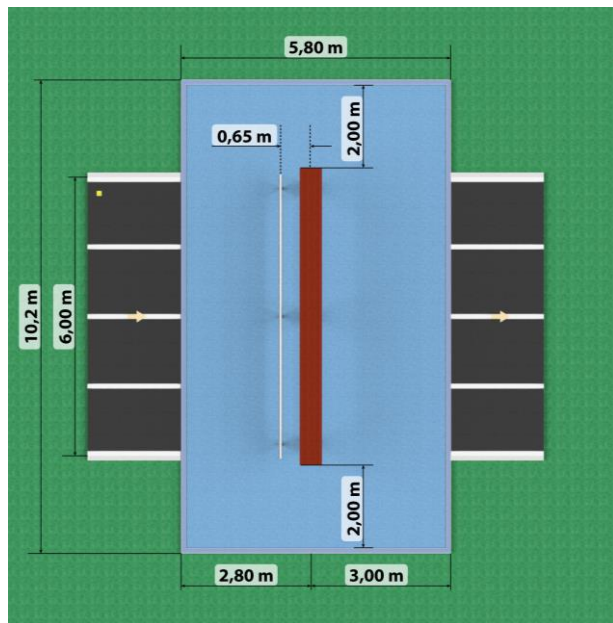
Bovenaanzicht en maatvoering
