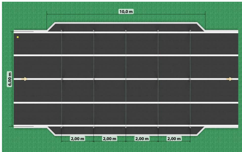
Bovenaanzicht en maatvoering
