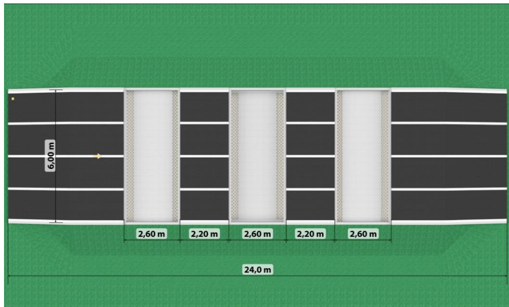
Bovenaanzicht en maatvoering
