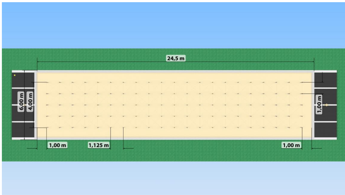
Bovenaanzicht en maatvoering
