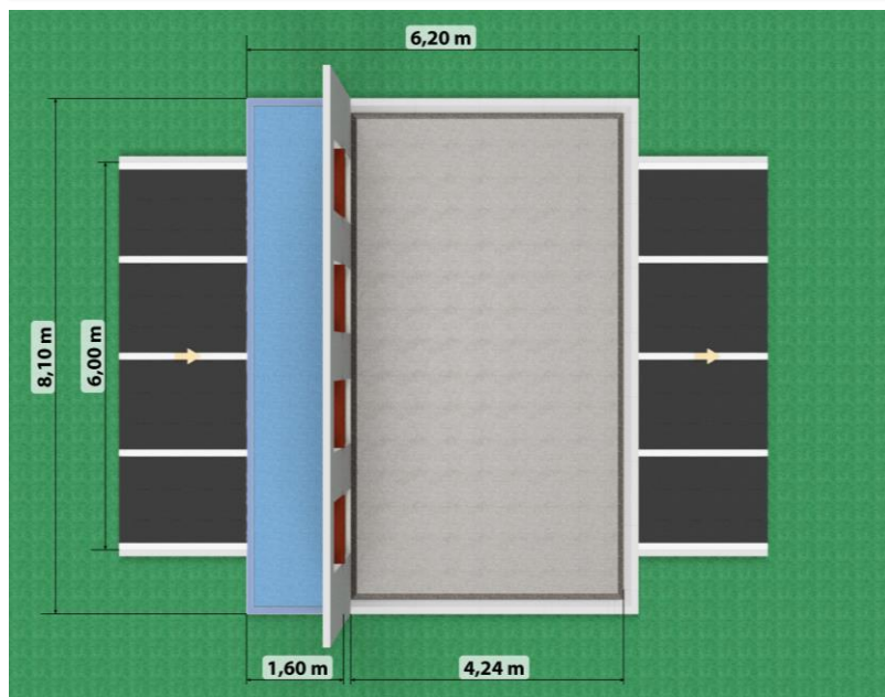
Bovenaanzicht en maatvoering
