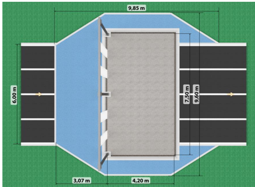
Bovenaanzicht en maatvoering
