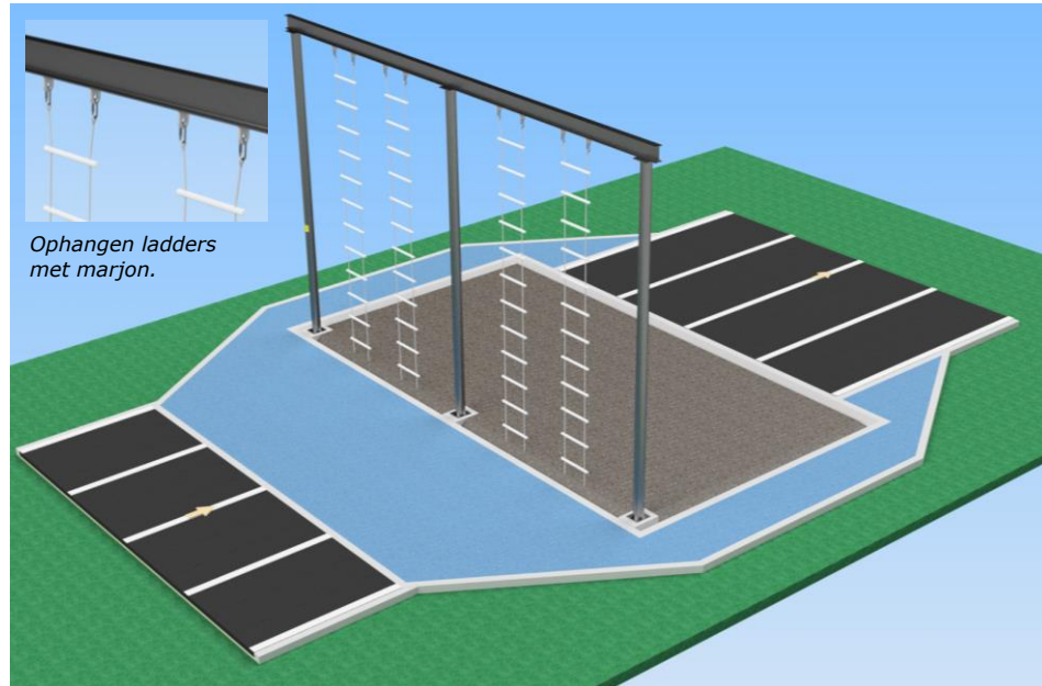
Isometrie
