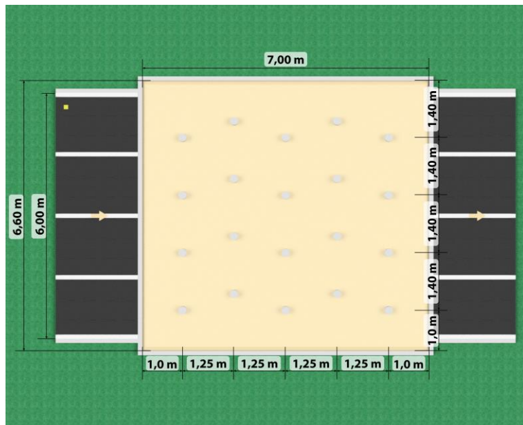
Bovenaanzicht en maatvoering
