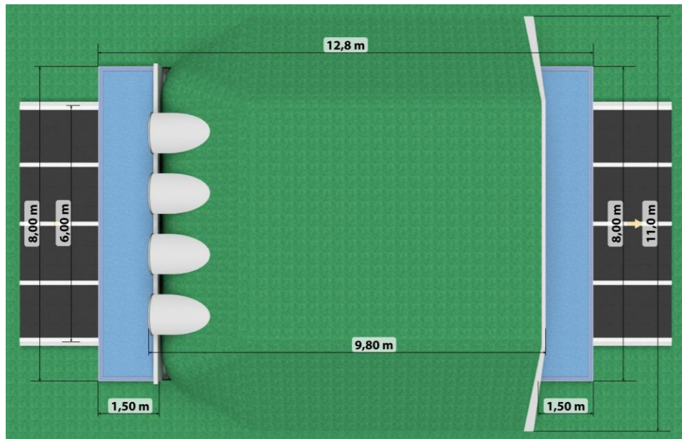
Bovenaanzicht en maatvoering
