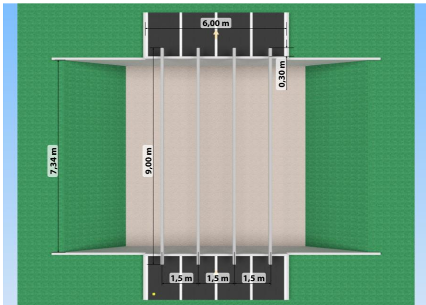
Bovenaanzicht en maatvoering
