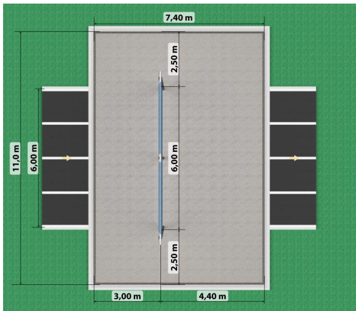
Bovenaanzicht en maatvoering
