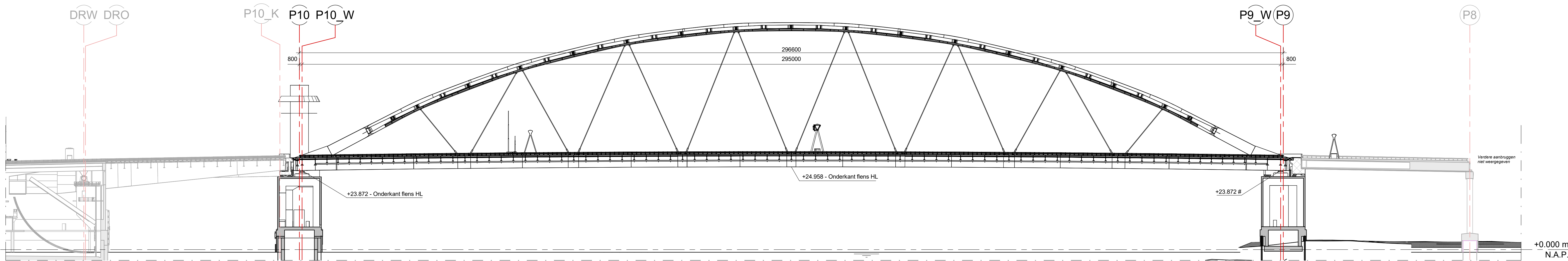
Zijaanzicht Westzijde WBBb schaal: 1 : 500
