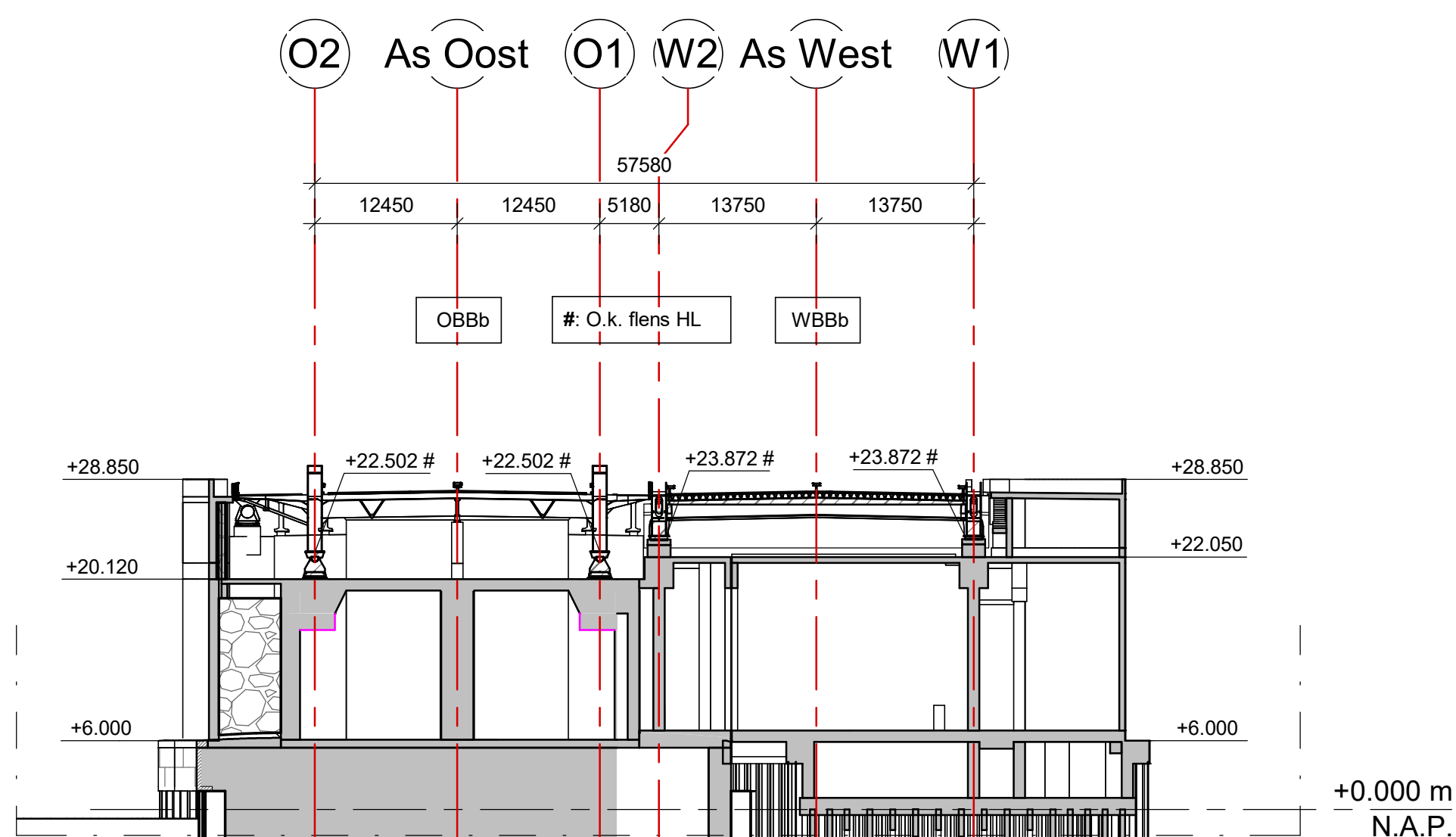
Doorsnede Pijler 9 schaal: 1 : 500
