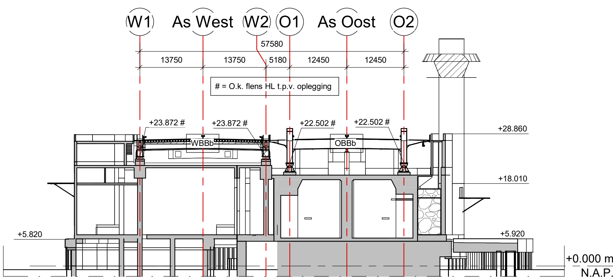
Doorsnede Pijler 10 schaal: 1 : 500
