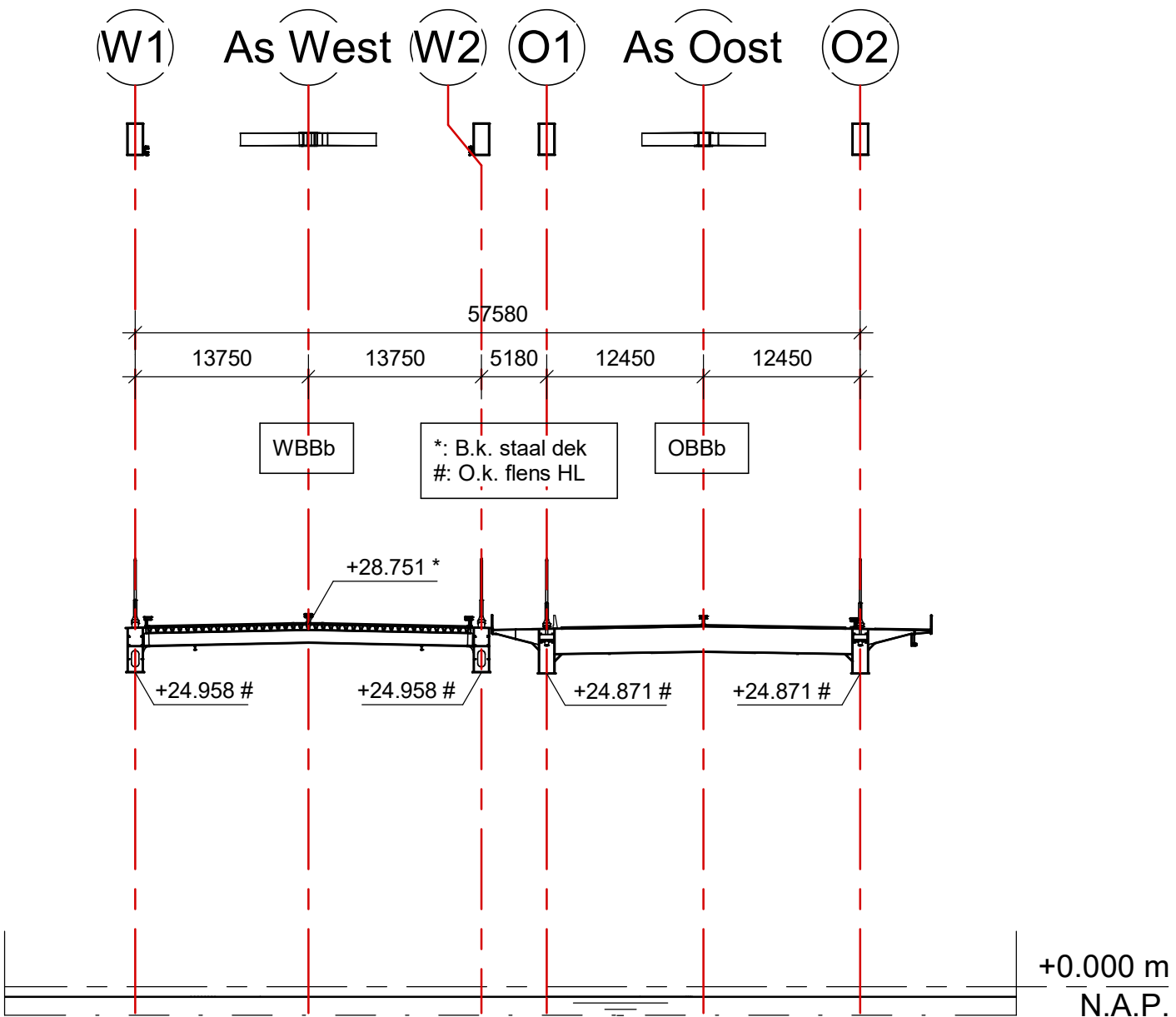
Doorsnede Midden overspanning schaal: 1 : 500
