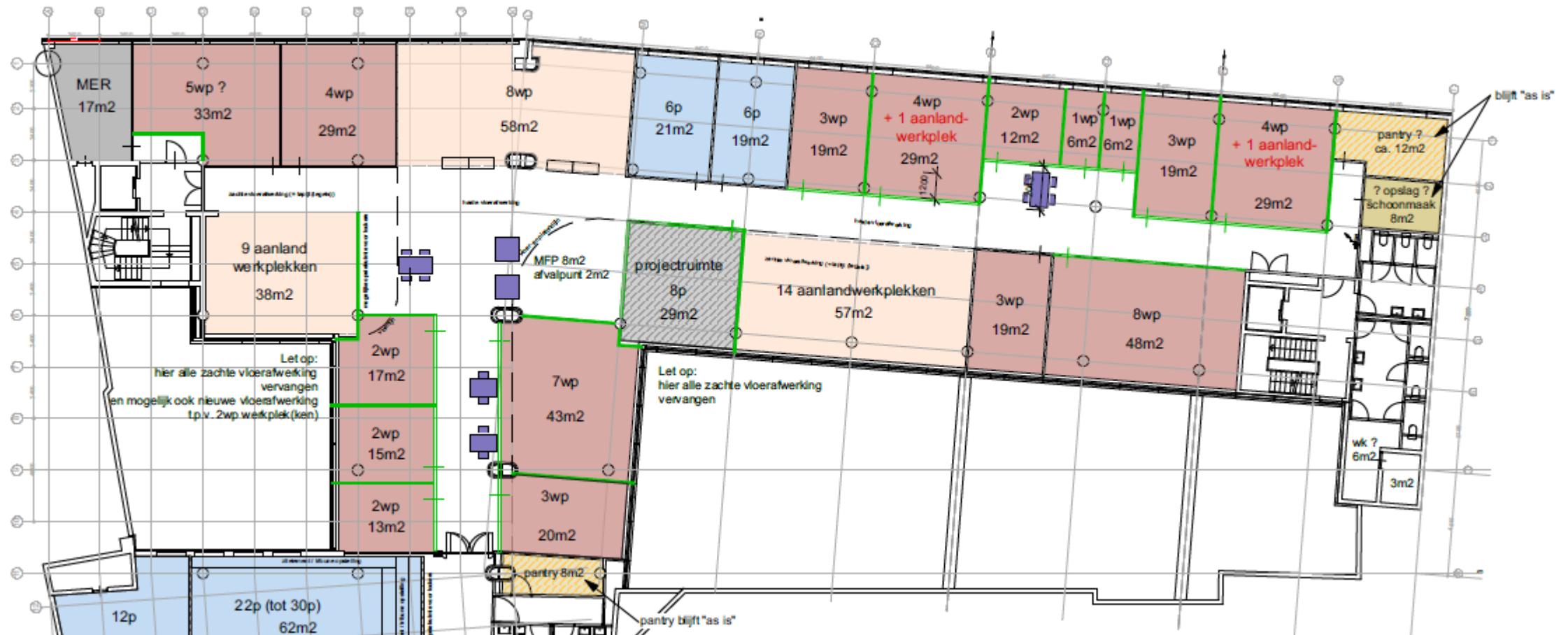
Uitsnede 1 e verdieping
