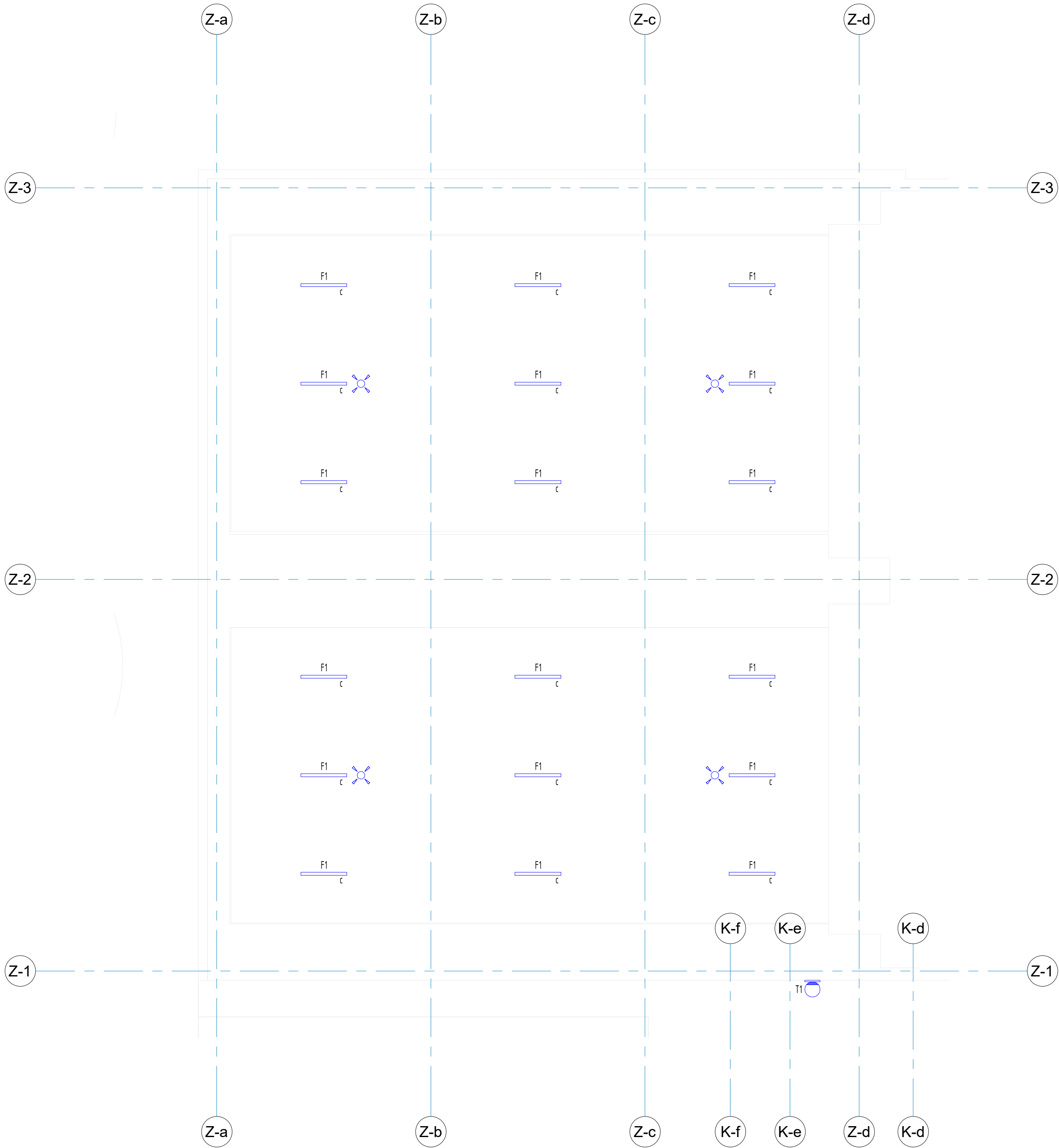
00 Verlichting Zoutopslag 1 : 100
