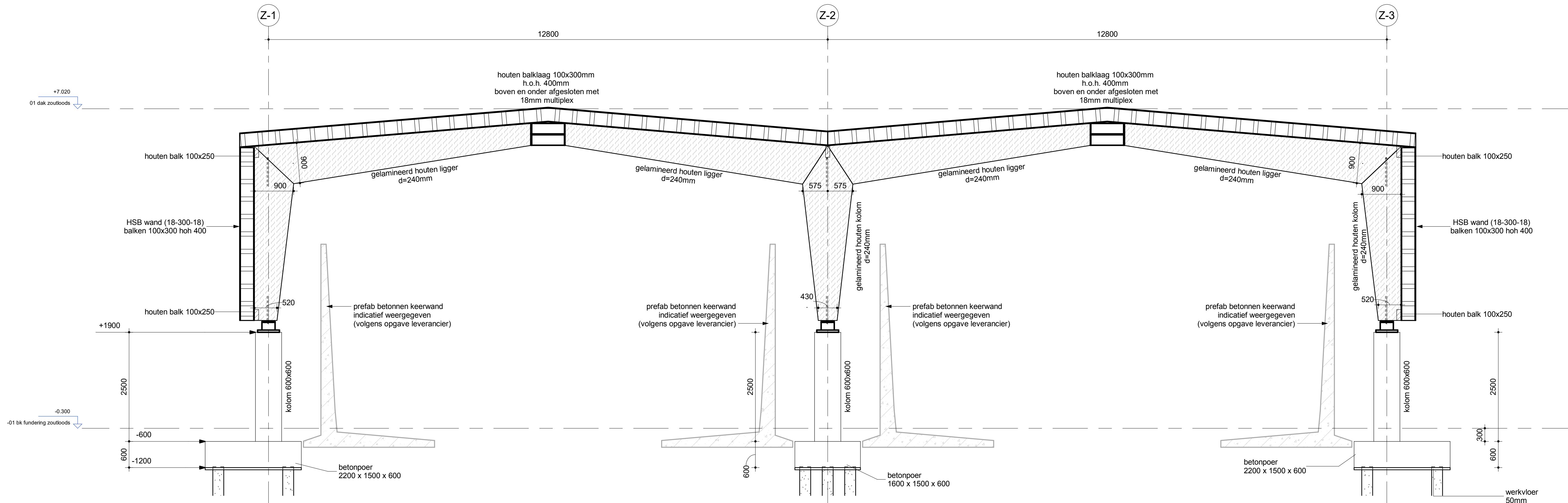
1 Doorsnede Schaa: 1 : 50
