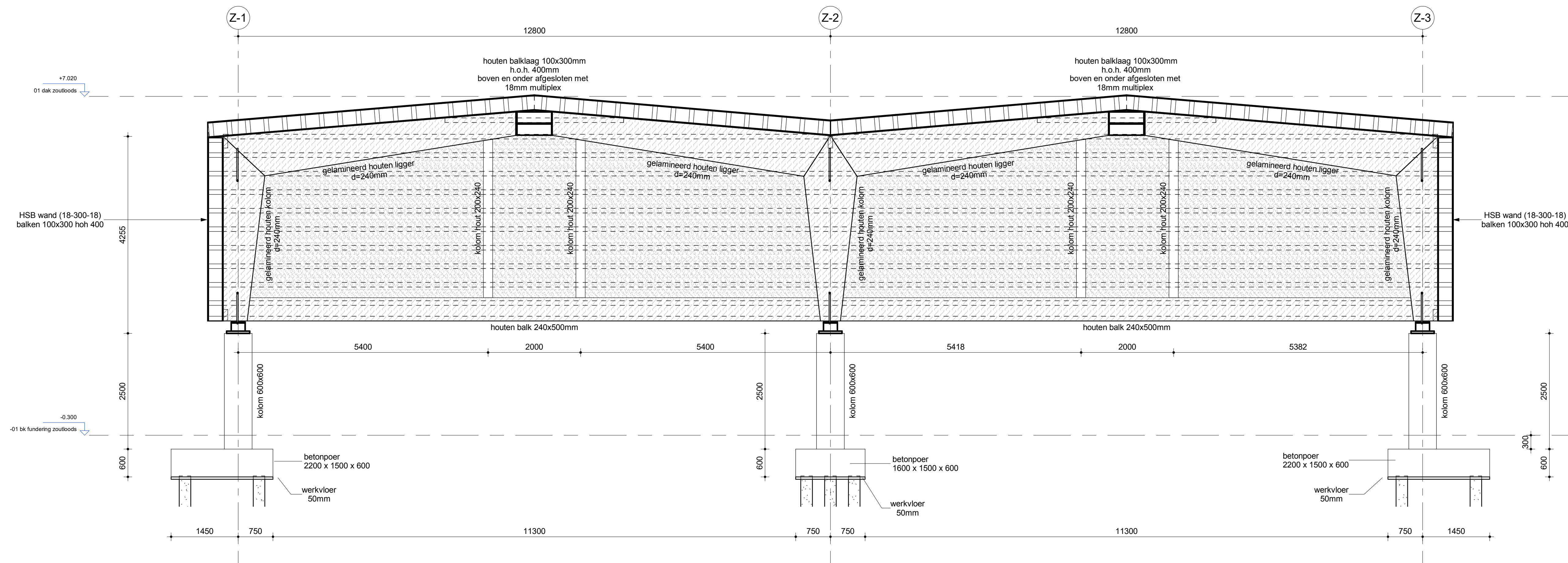
2 Doorsnede Schaa: 1 : 50
