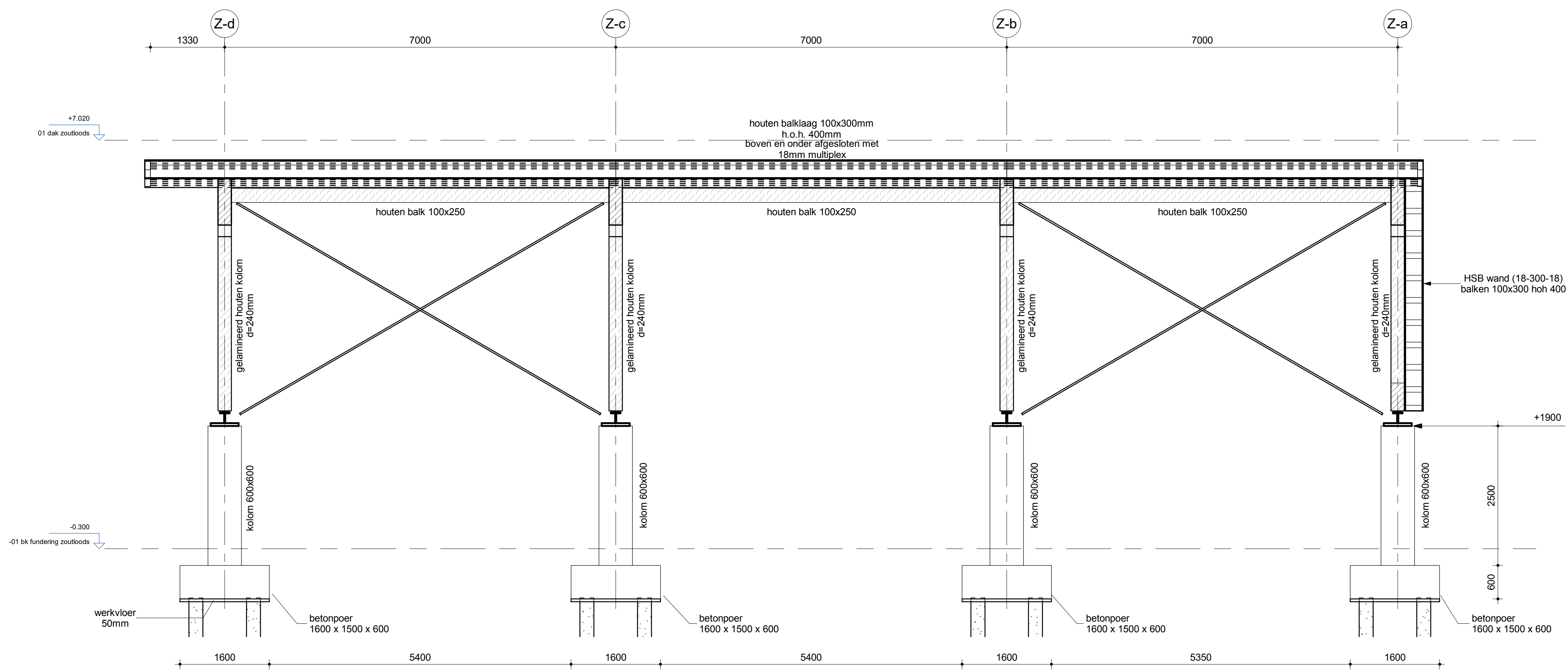
3 Doorsnede Schaa: 1 : 50
