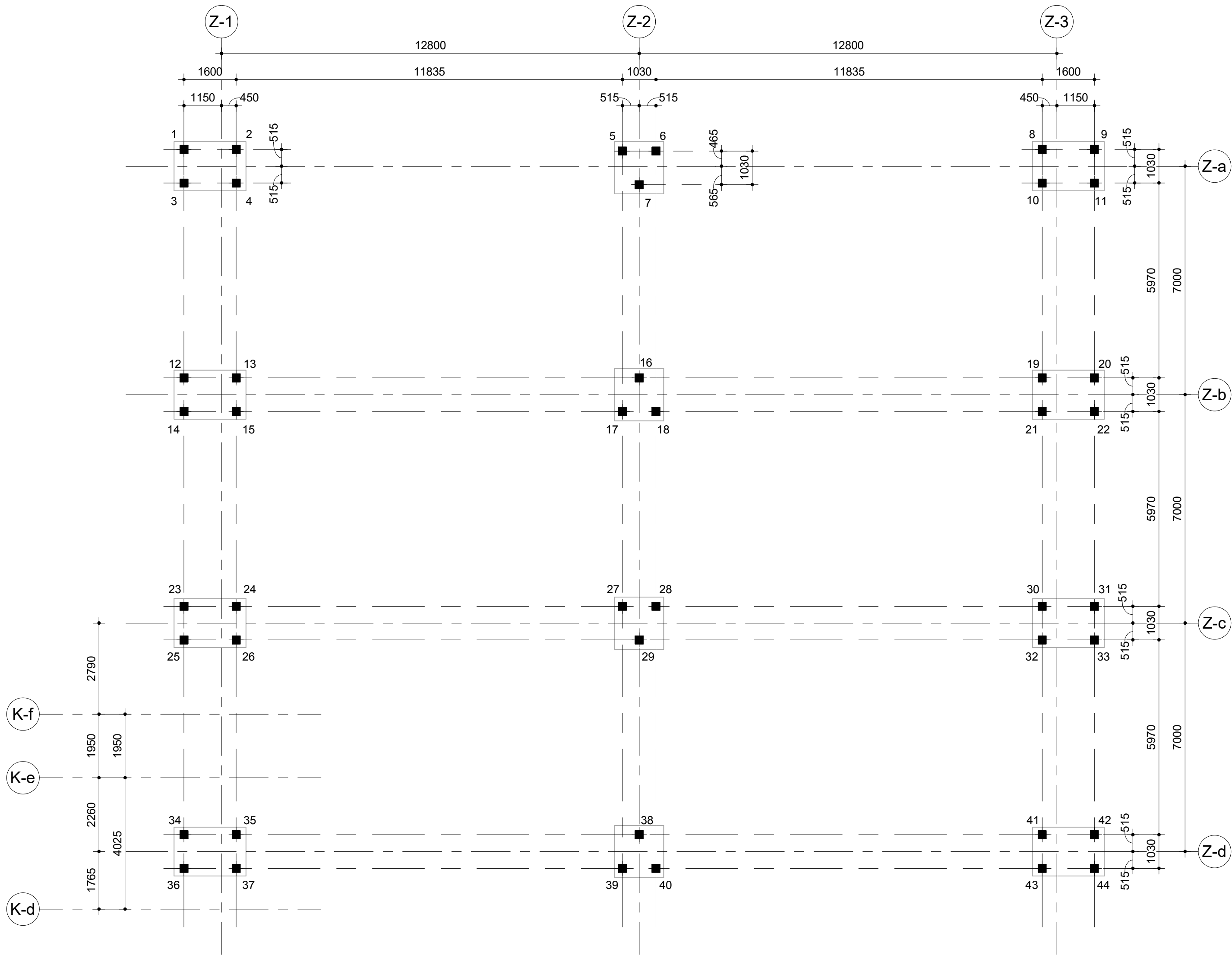
P Palenplan Schaal: 1 : 100
