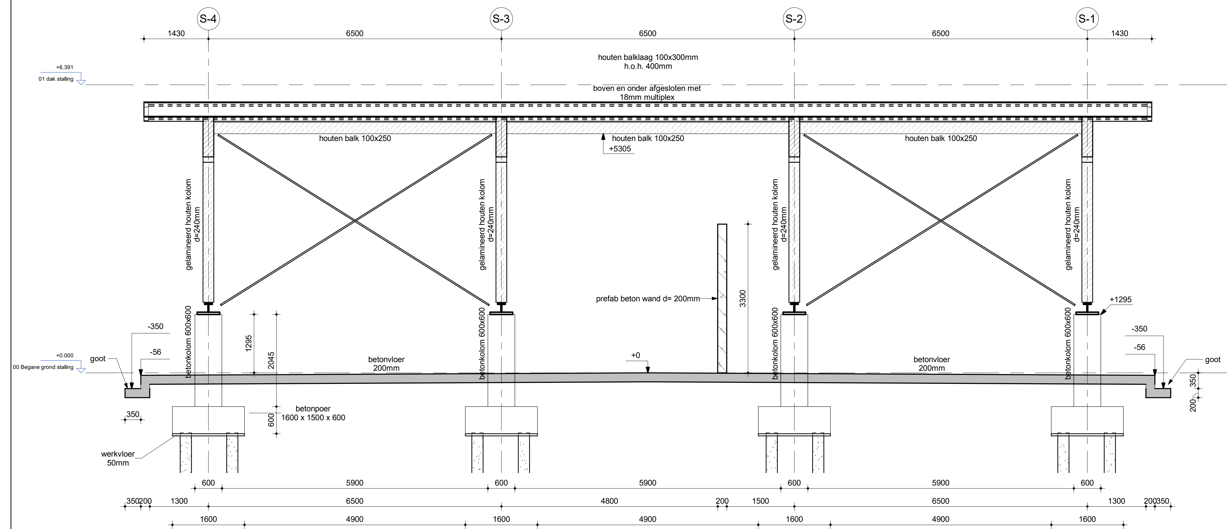
1 Doorsnede Schaal: 1 : 50
