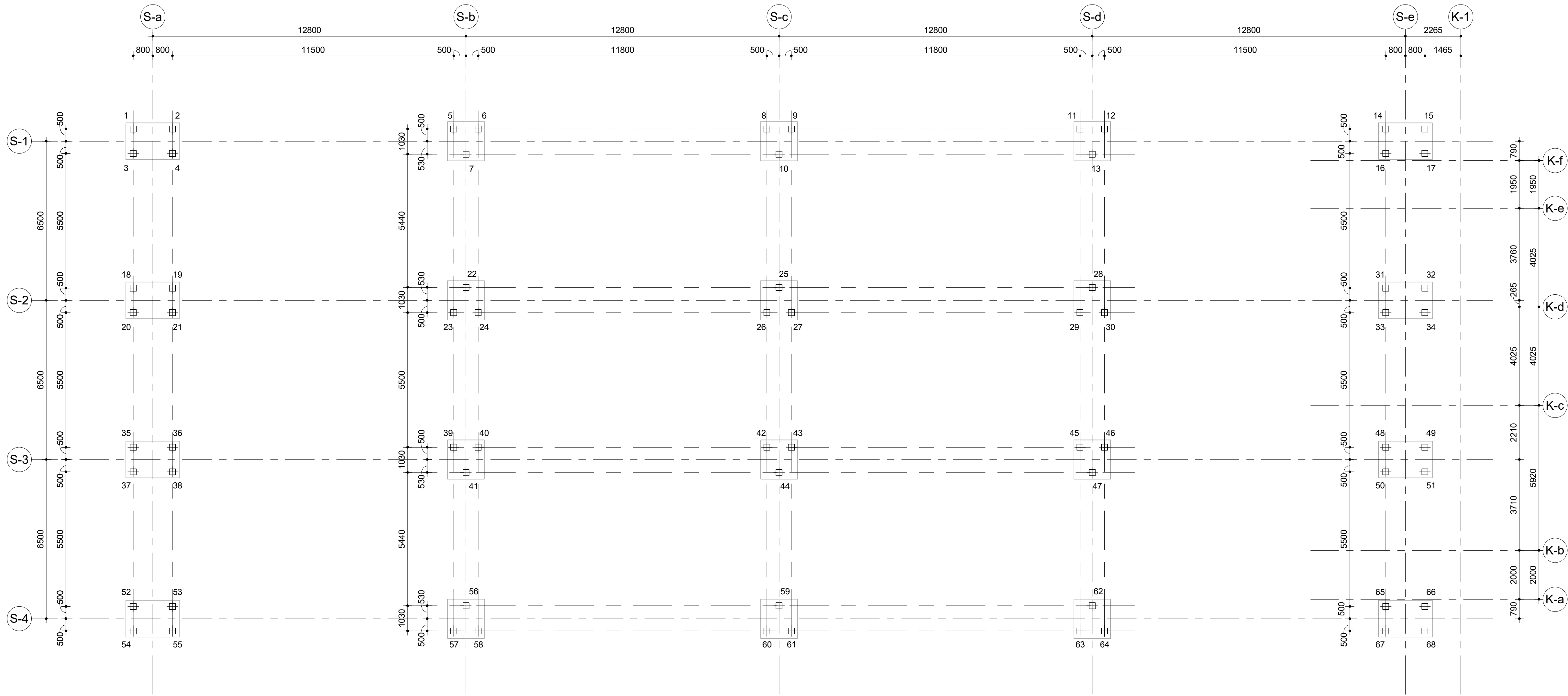
P Palenplan Schaal: 1 : 100
