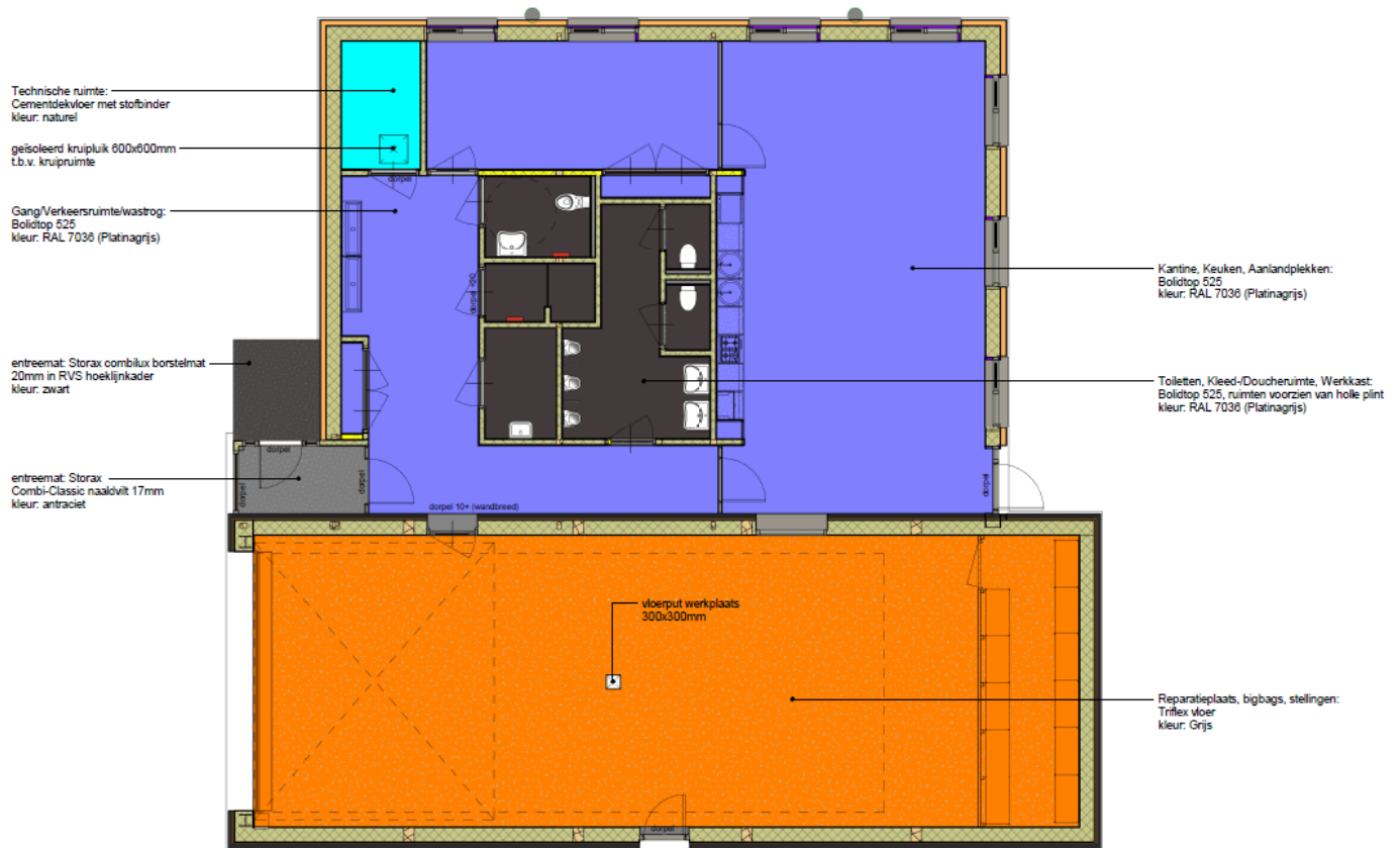
Vloerafwerkingen Dienstengebouw
