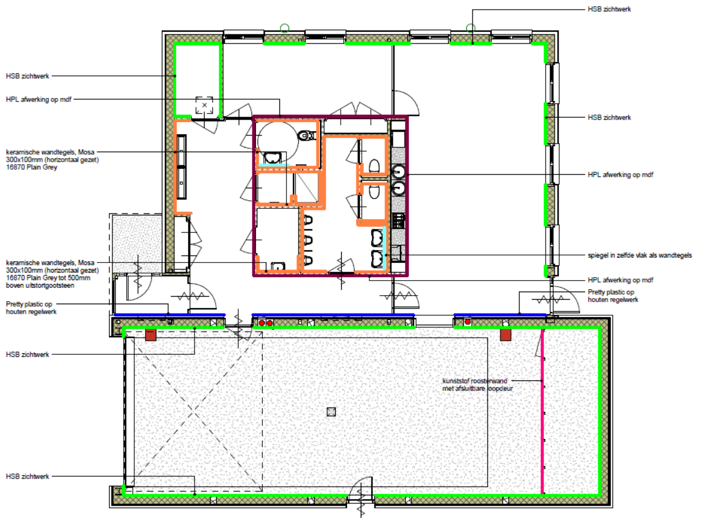
Begane grond - kantine / kantoor / werkplaats
