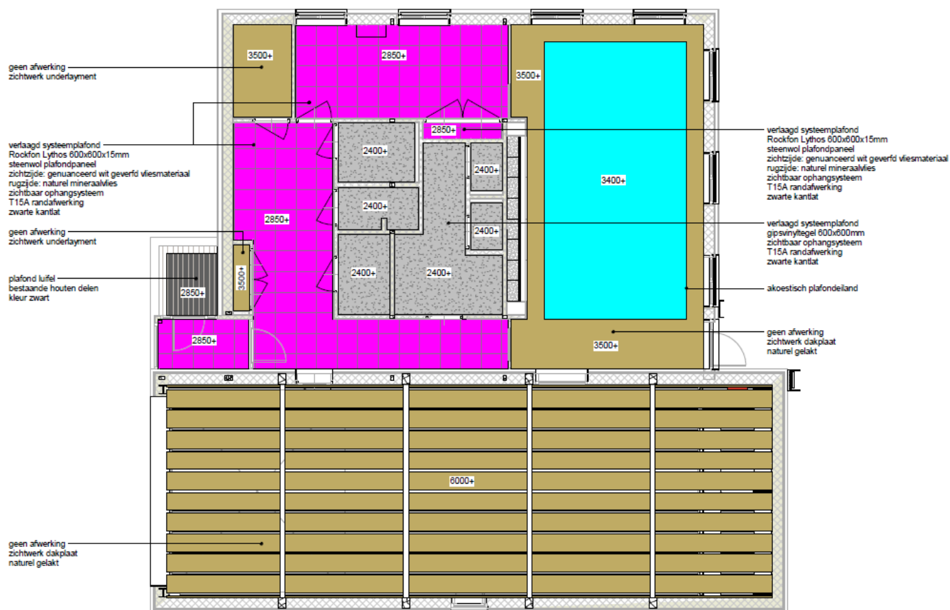
Plafondafwerking Dienstengebouw
