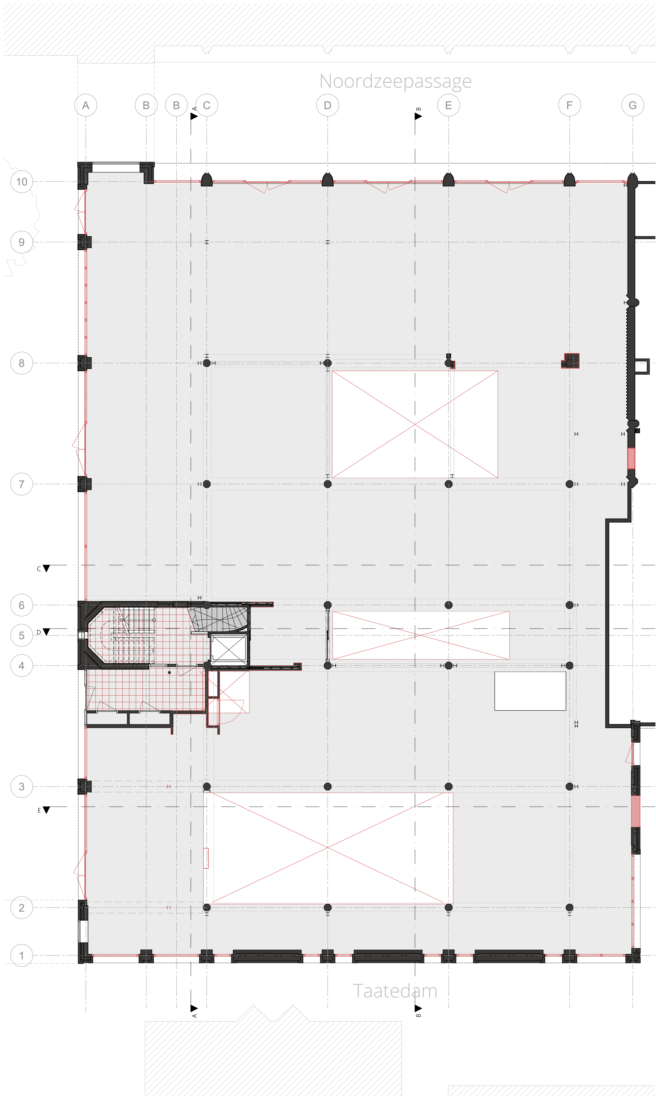
BEGANE GROND 1:100
