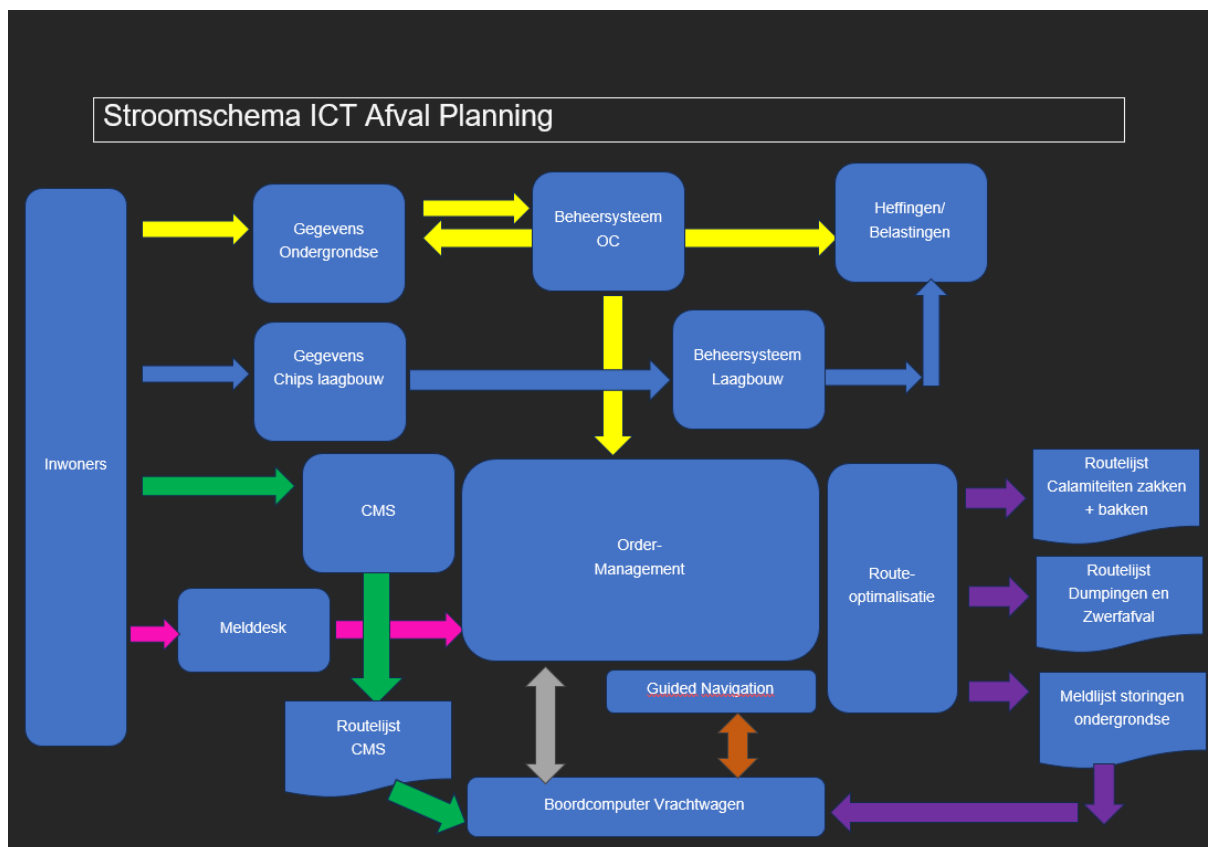
Figuur 2 Stroomschema ICT Afval Planning
